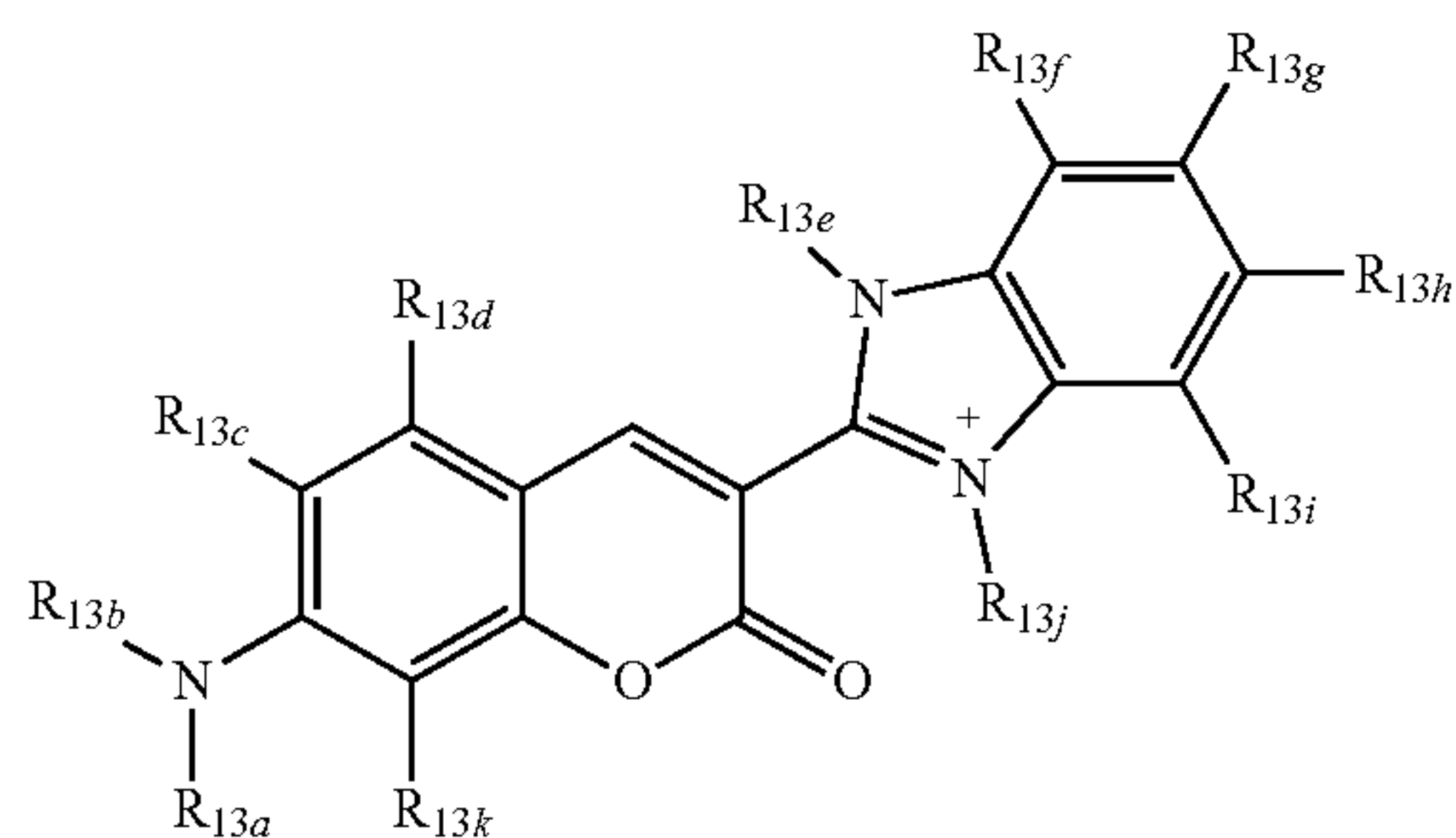
(XXVIIm)
