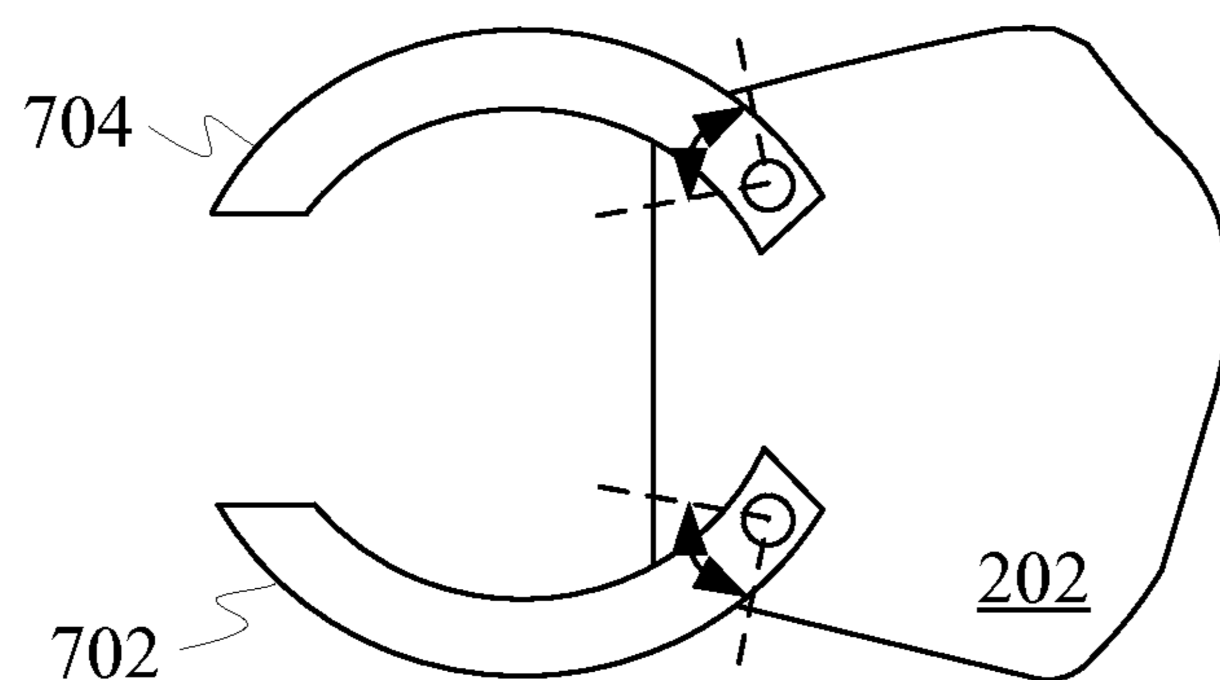
FIG. 7A
