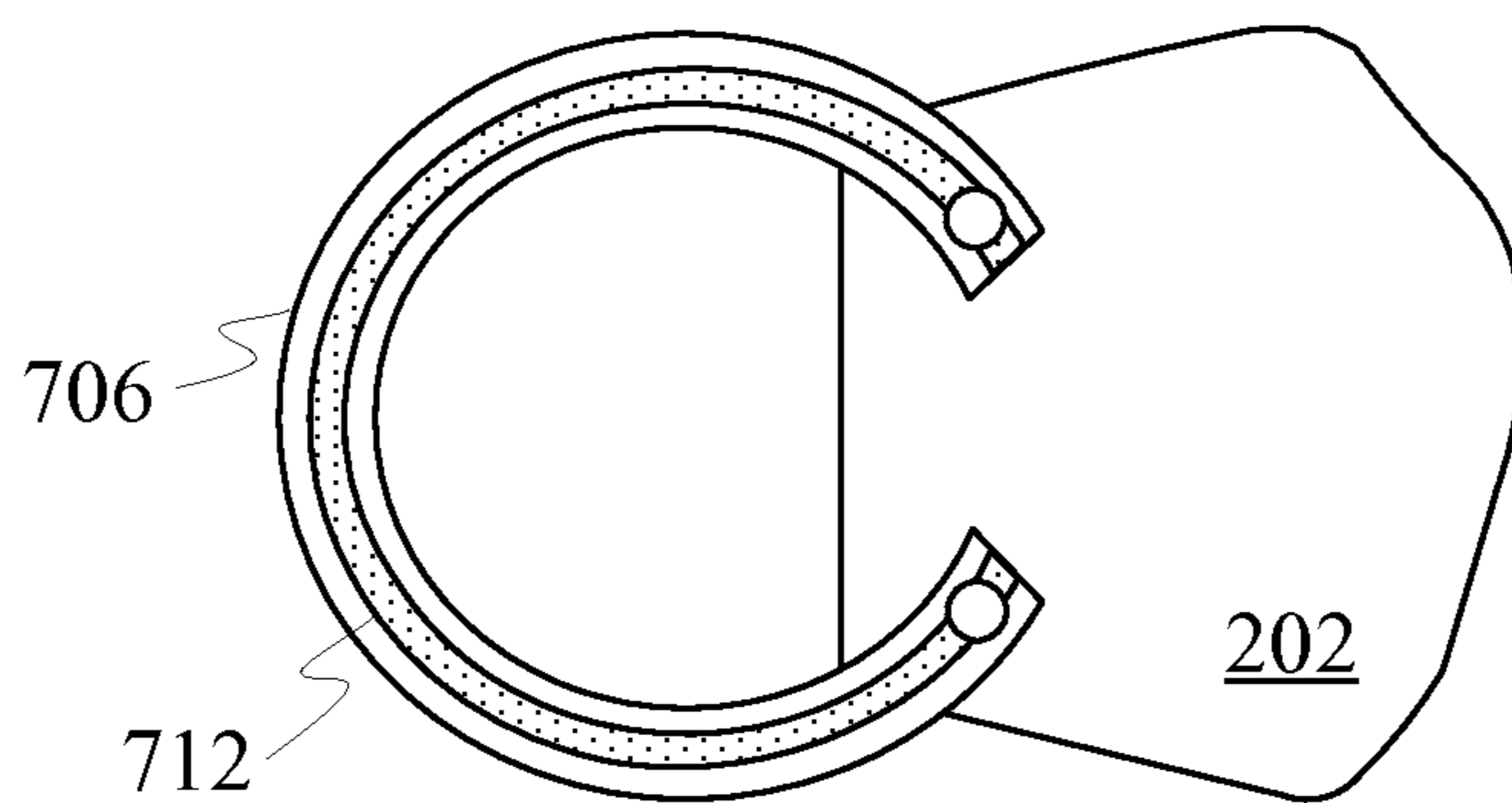
FIG. 7C
