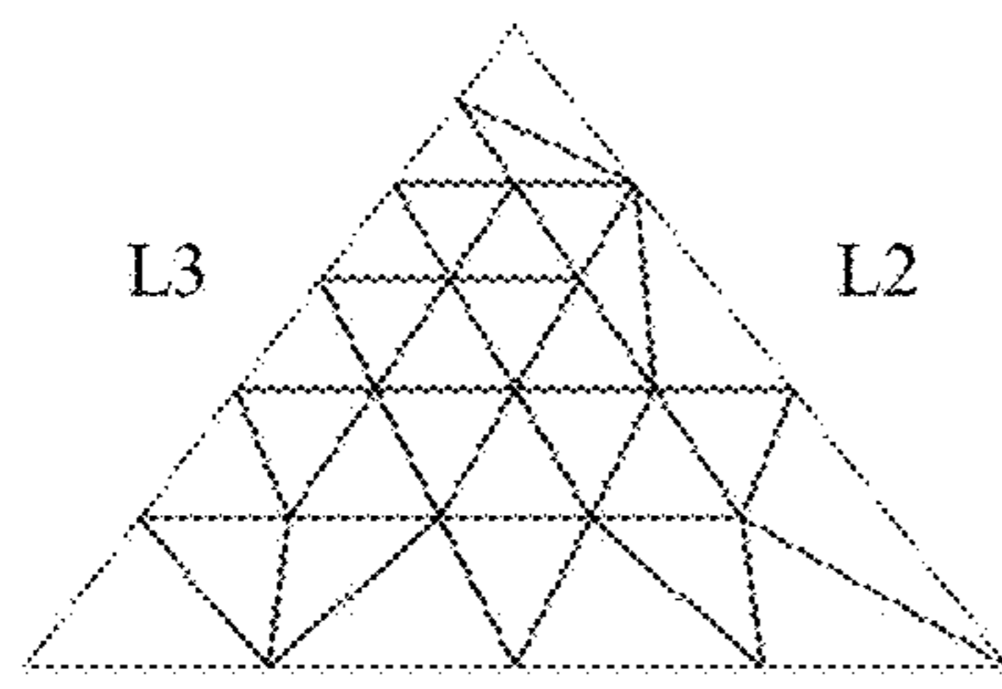
L1 L1=3, L2=2, L3=5
