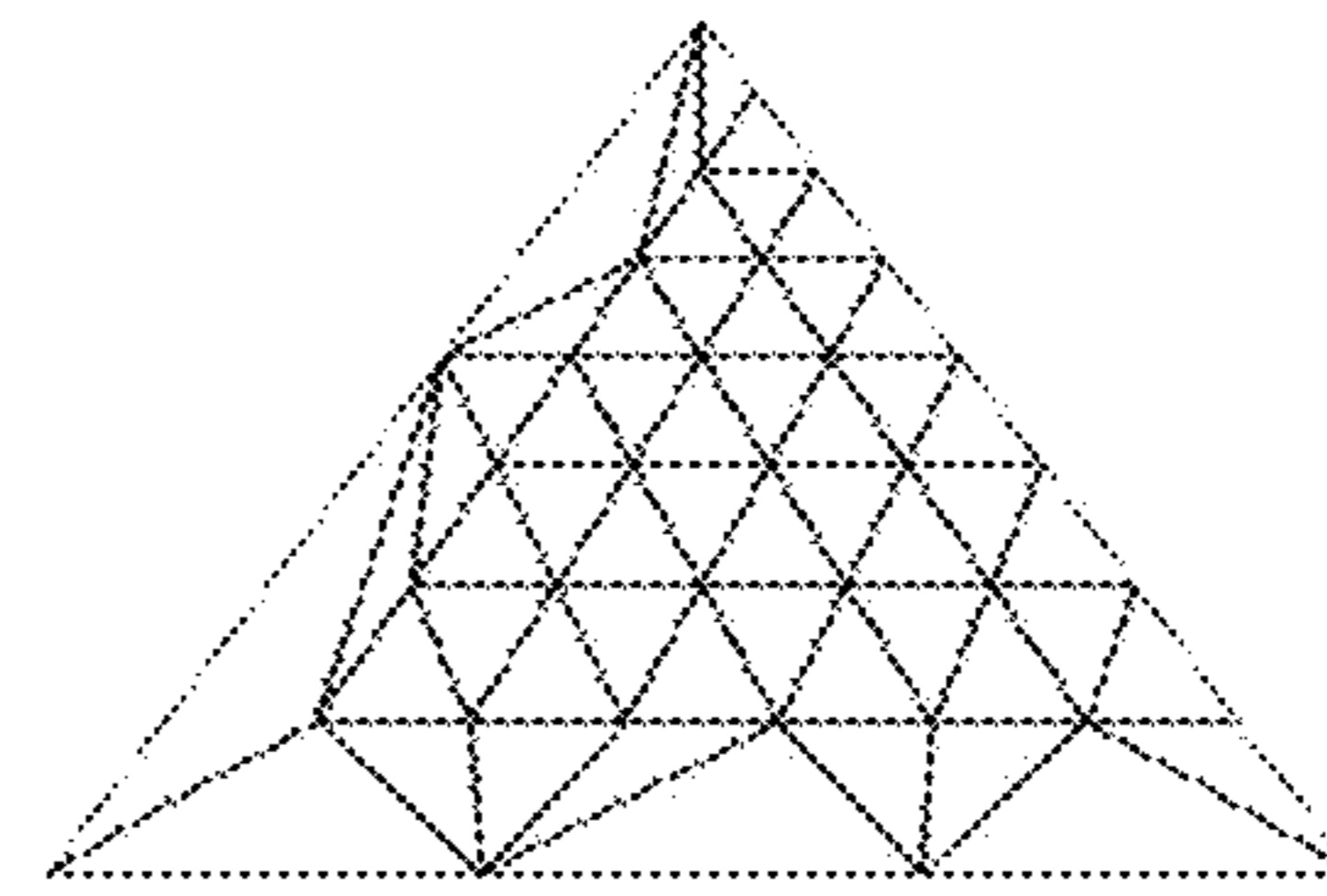
L1=2, L2=7, L3=1
