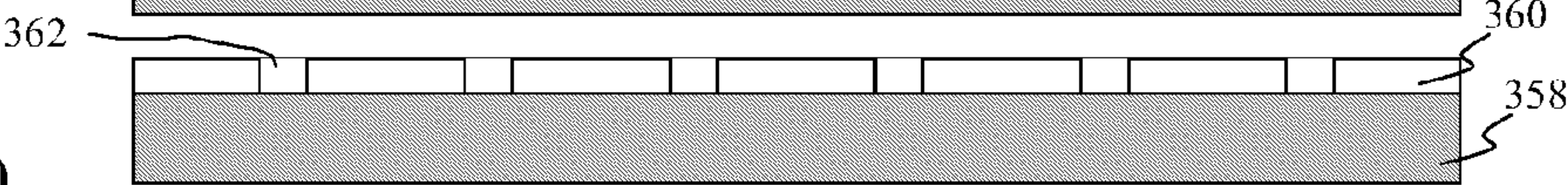
FIG. 44C (patterning)
