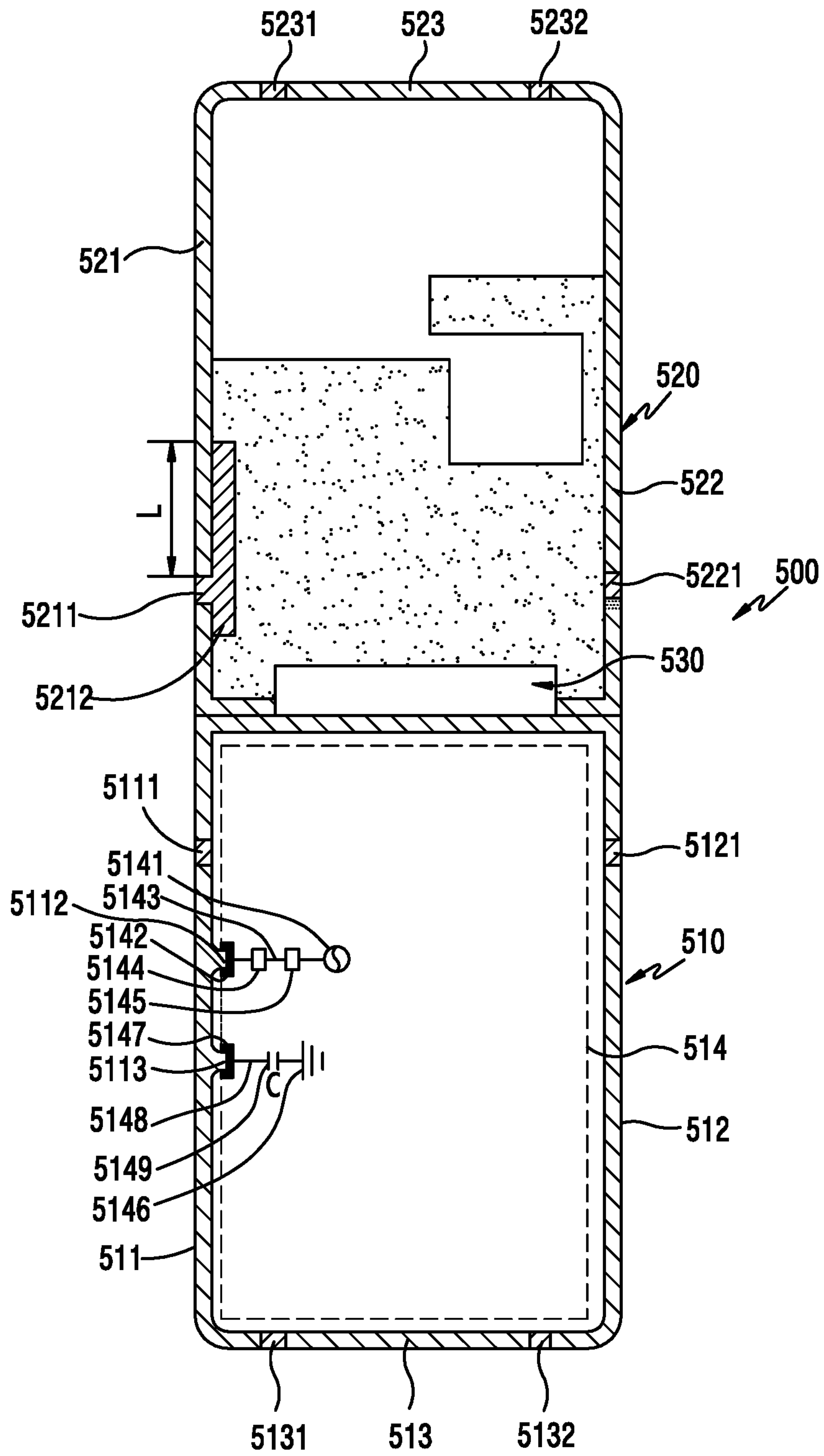
FIG. 5B
