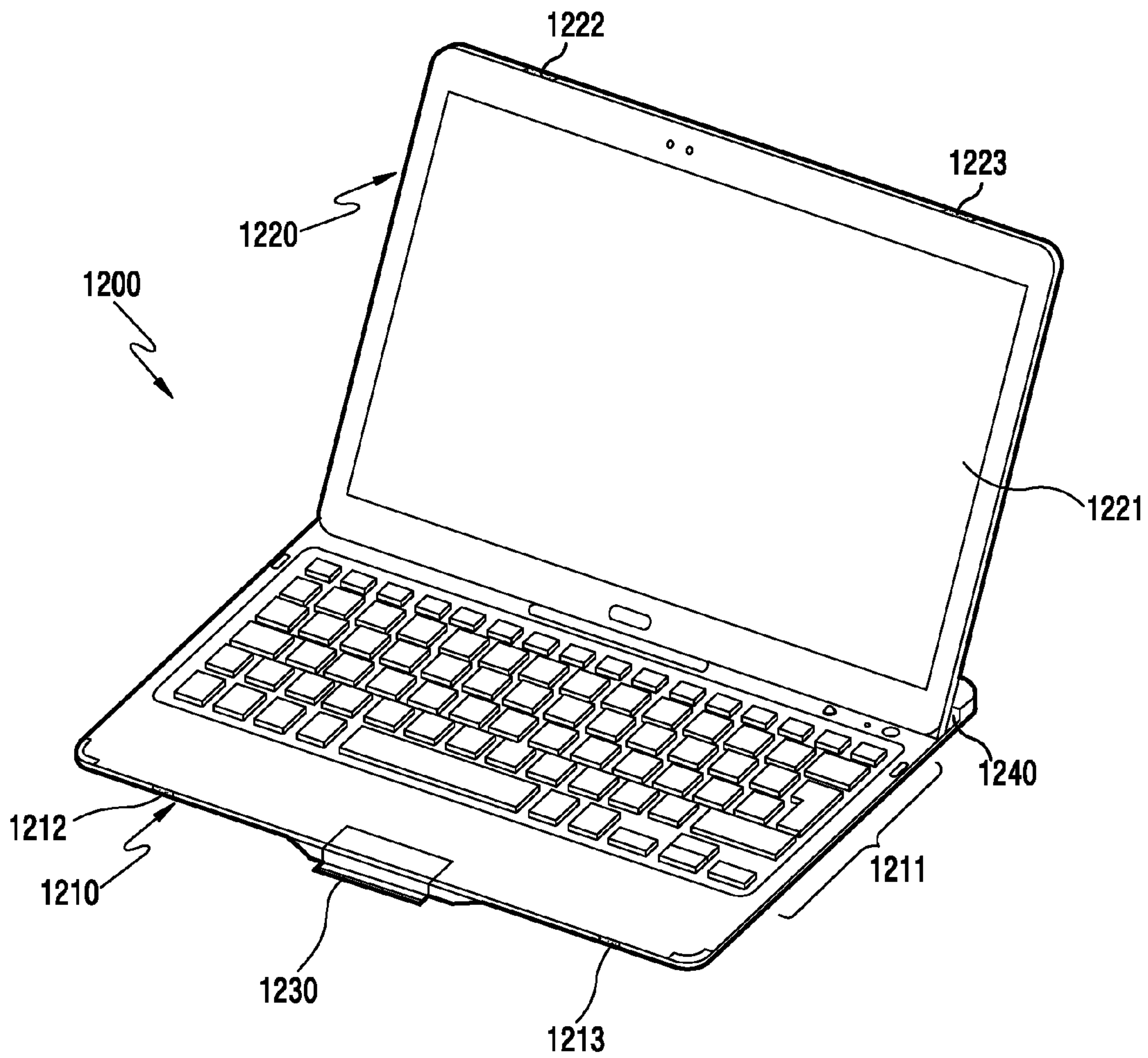
FIG. 12A
