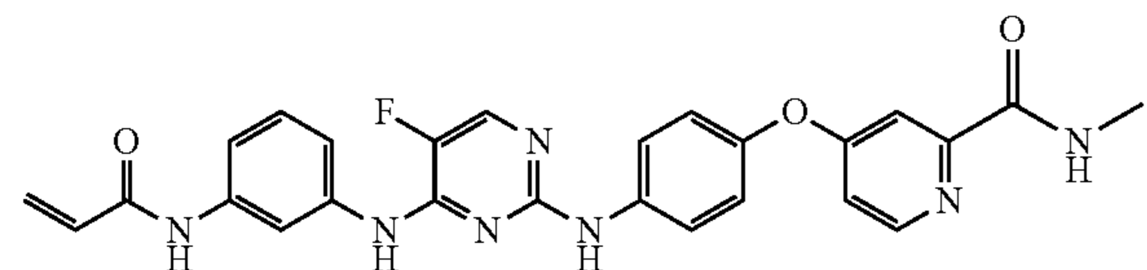
CNX-774
