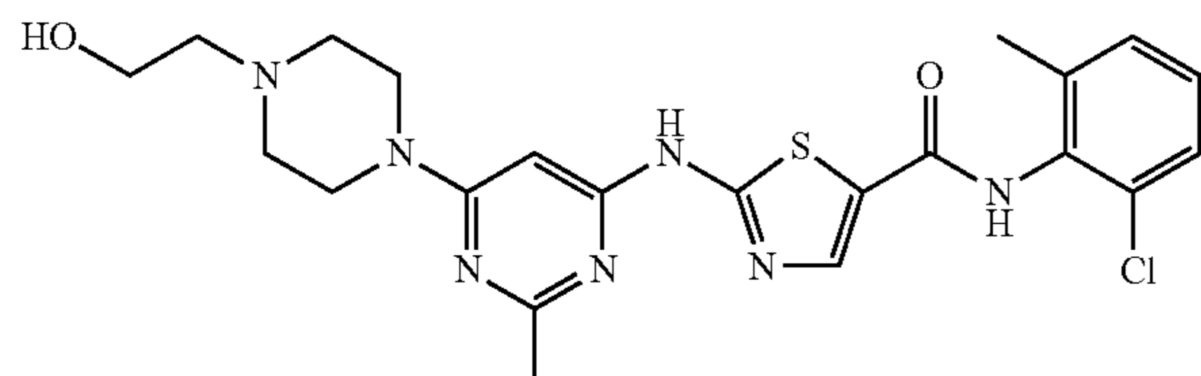
Dasatinib
