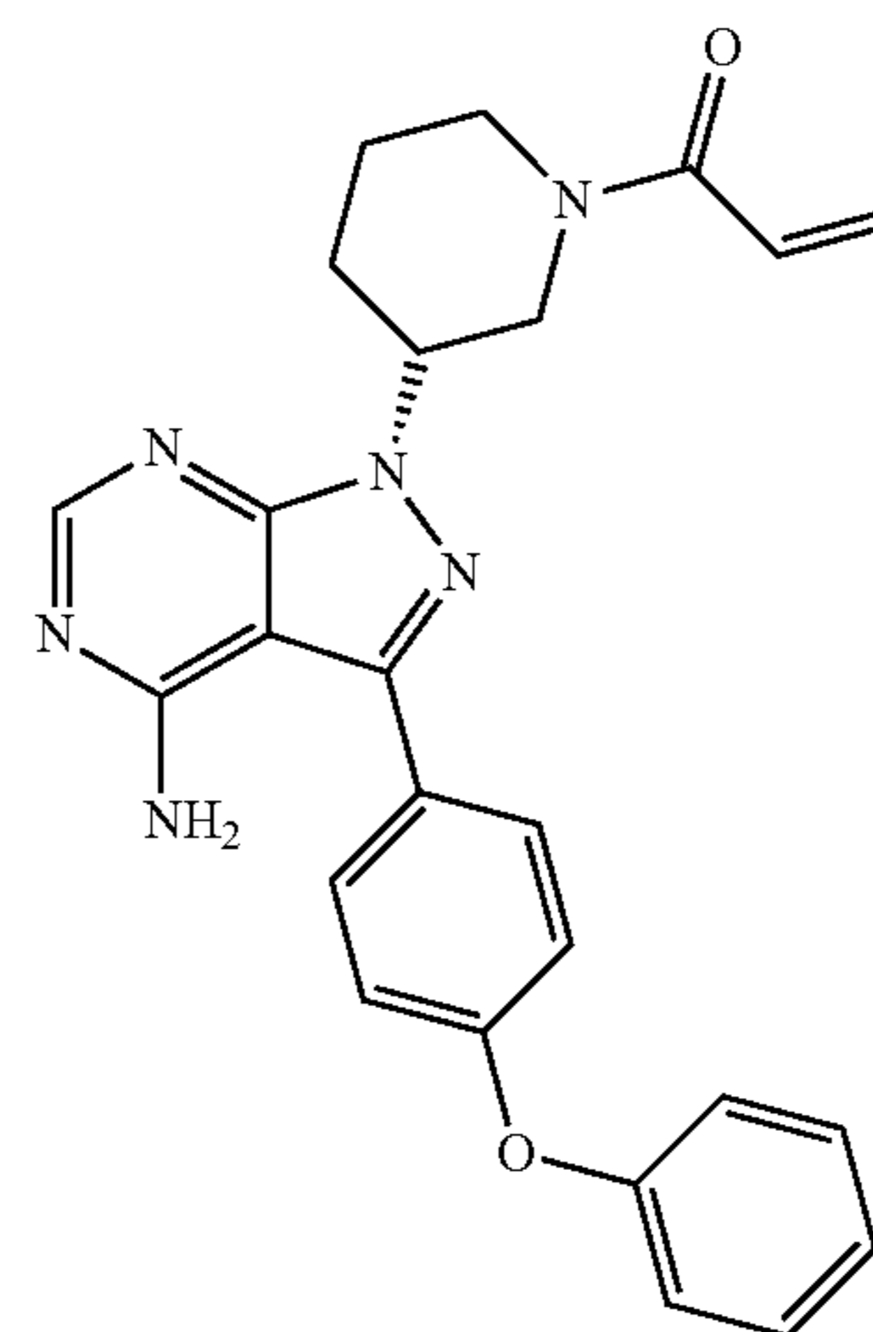
Ibrutinib
