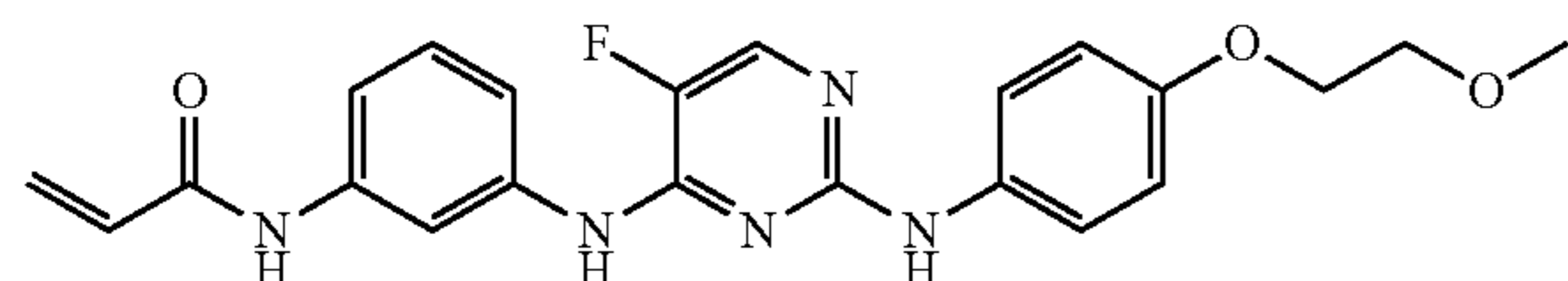
CC-292
