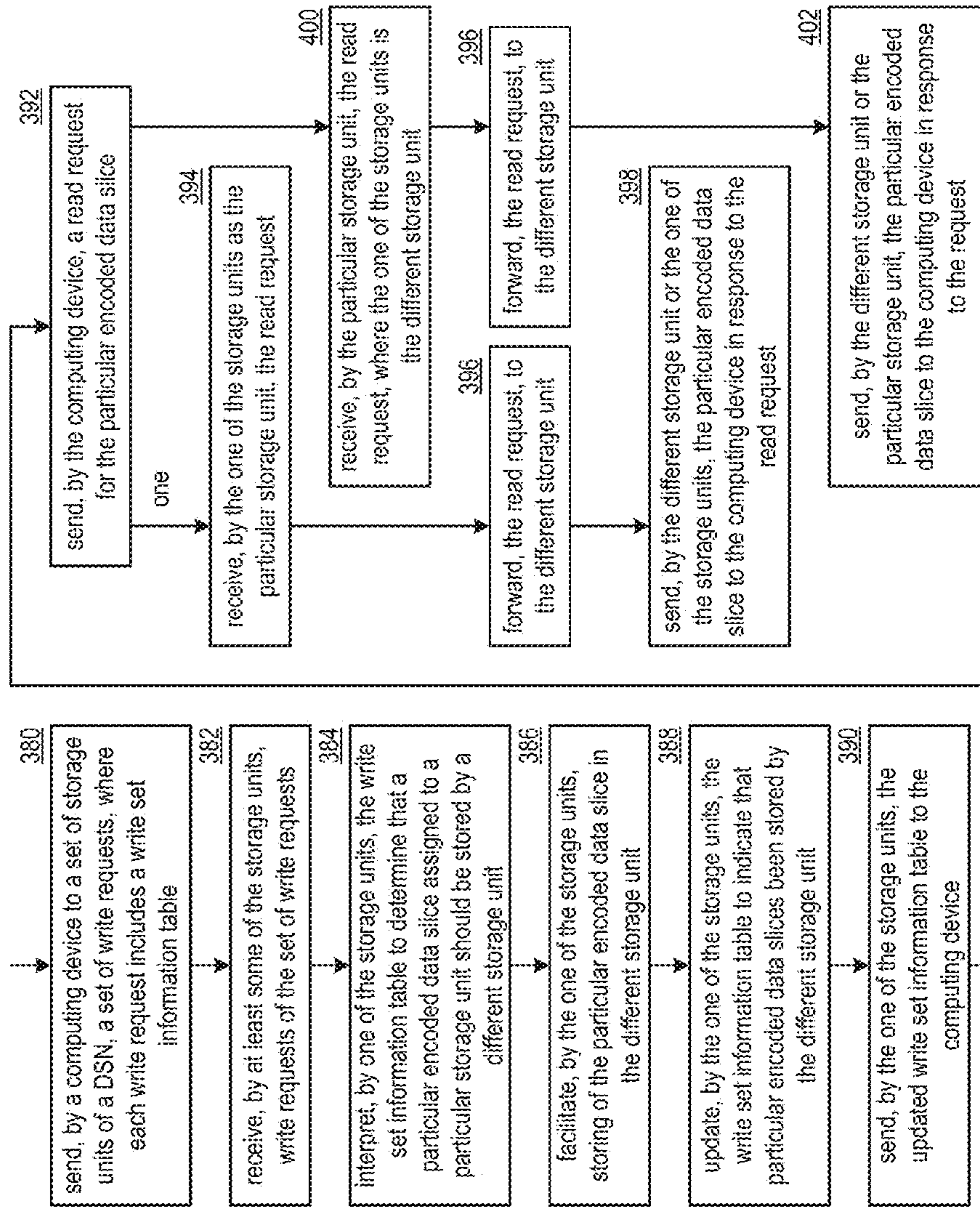
FIG. 400
