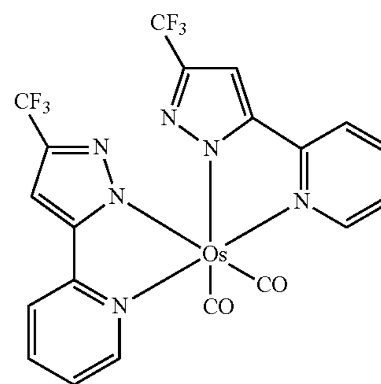
Os(fppz) 2 (CO) 2
