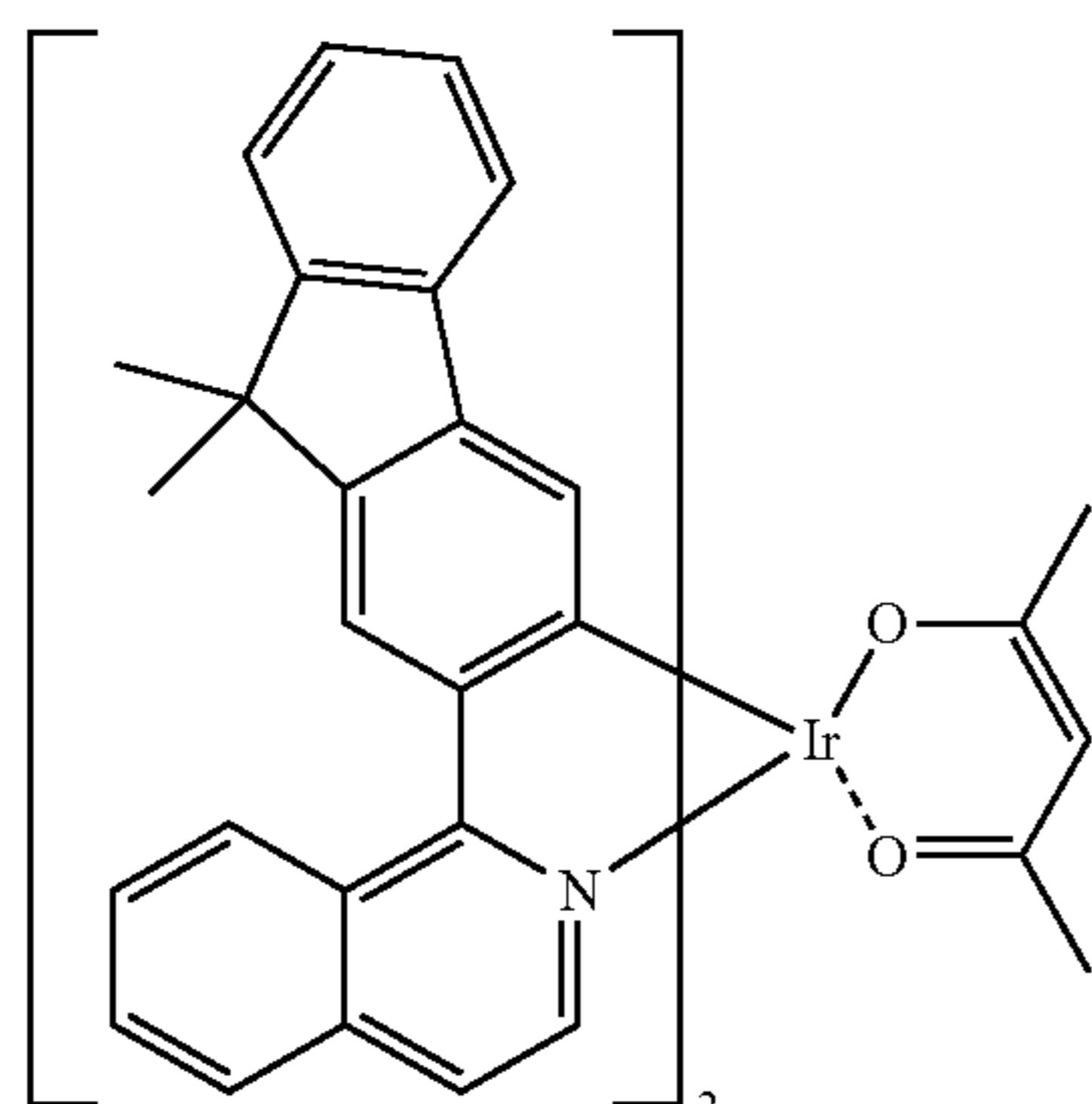
Ir(fliq) 2 (acac)
