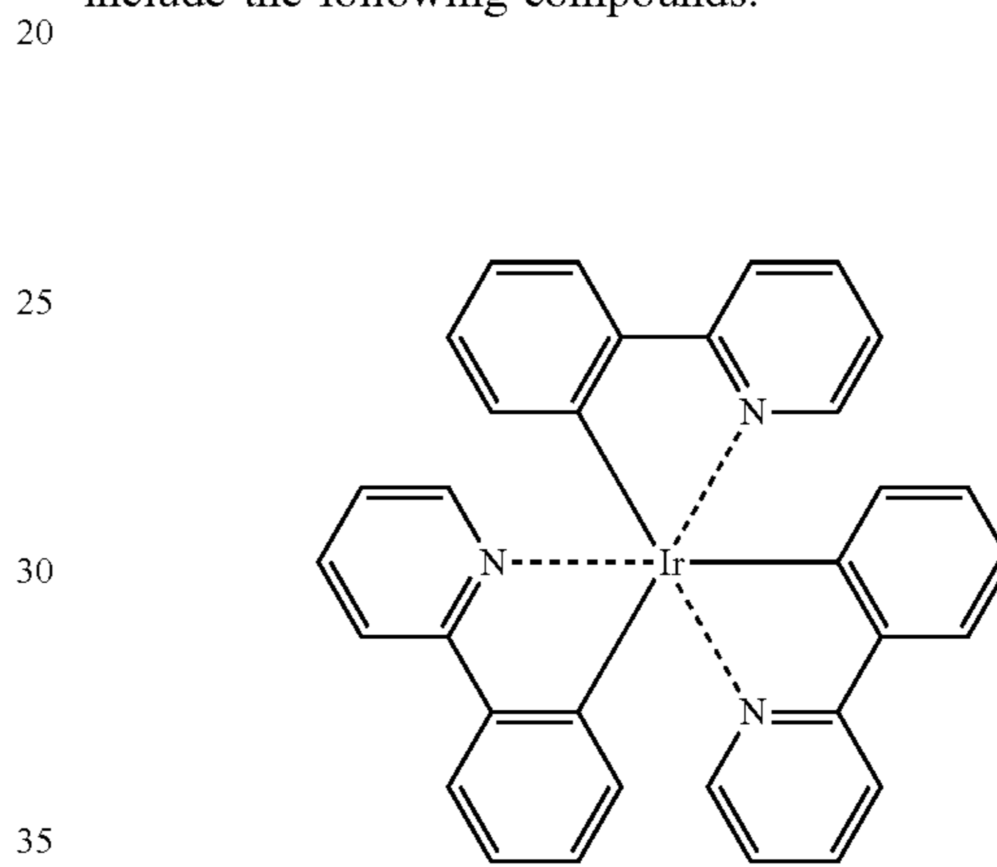
Ir(ppy) 3
