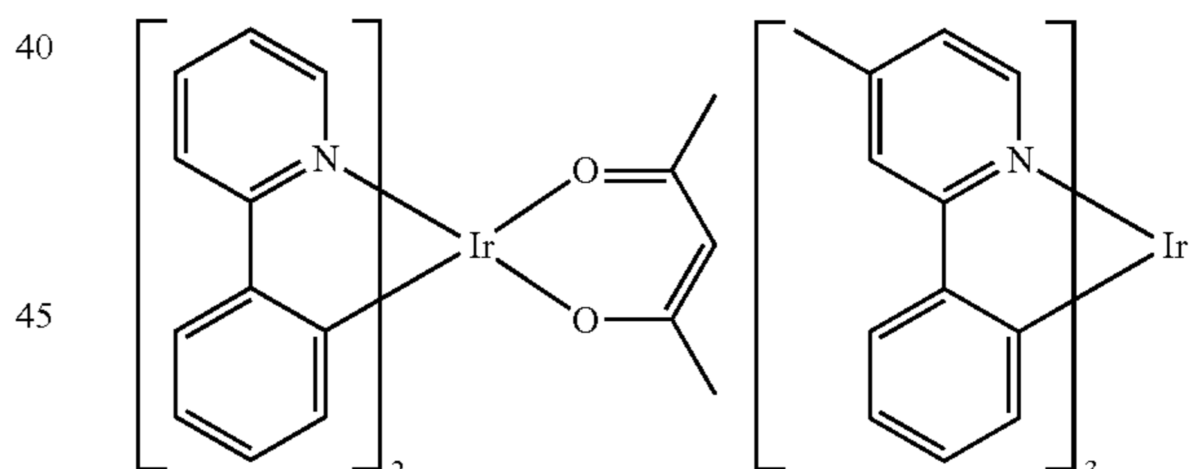
Ir(ppy) 2 (acac)
