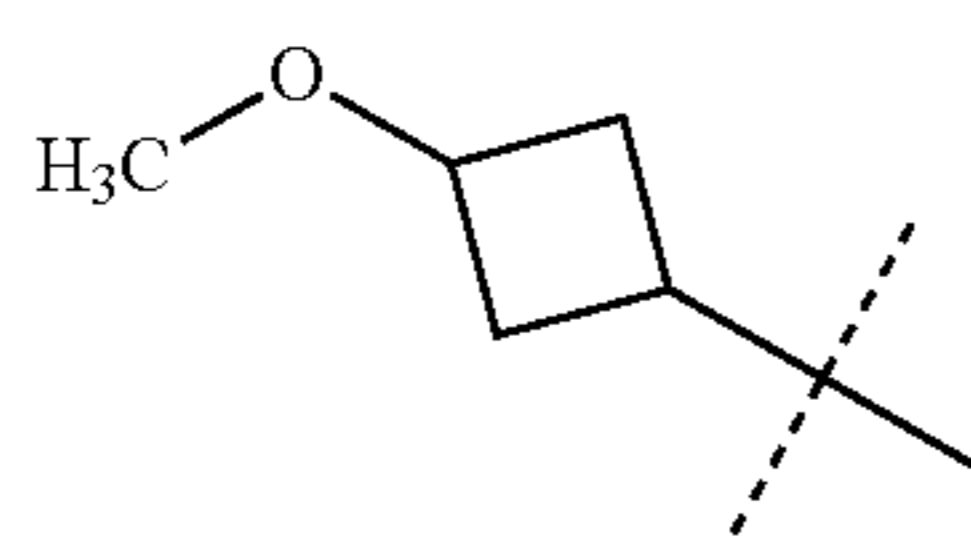
1-methoxycyclobut-3-yl/3-methoxycyclobut-1-yl
