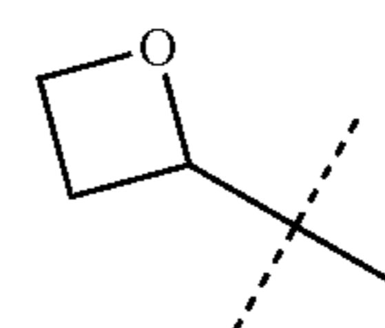
Oxetan-2-yl
