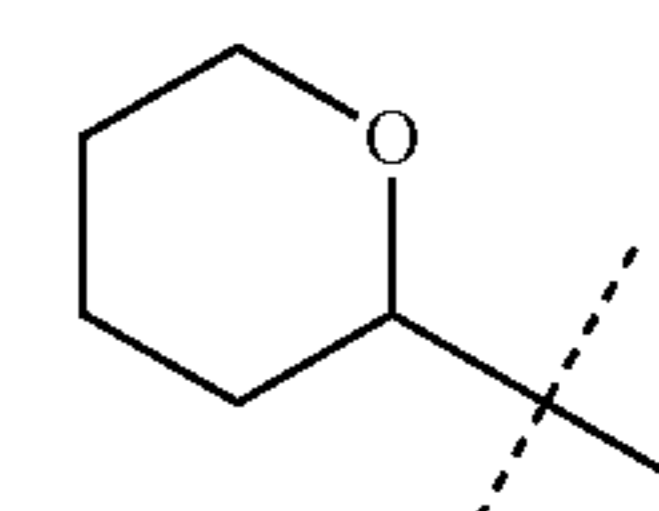
Oxan-2-yl
