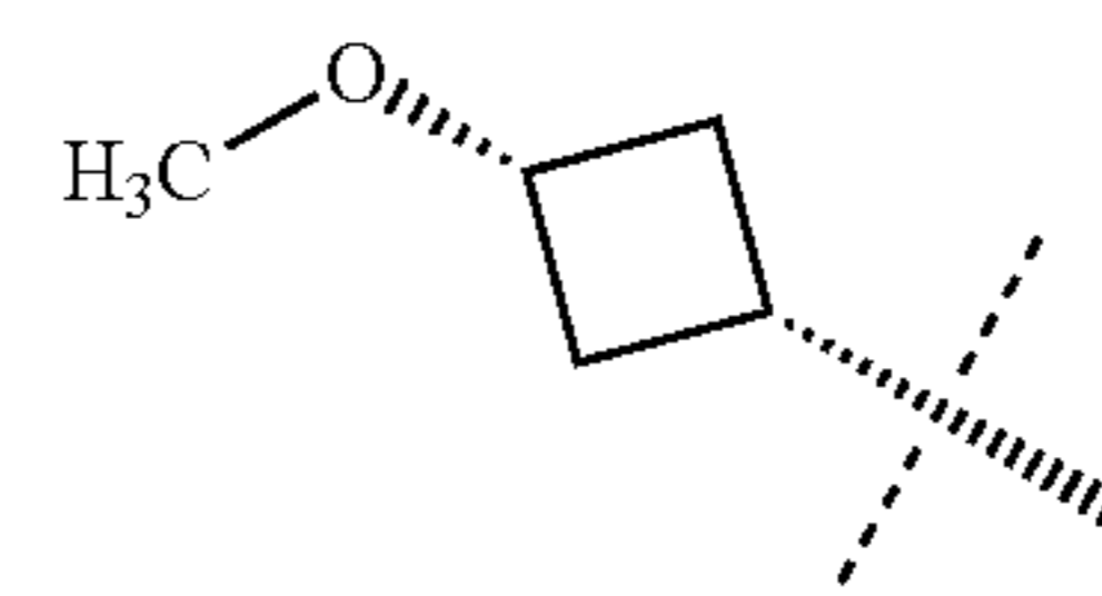
cis-1-methoxycyclobut-3-yl/cis-3-methoxycyclobut-1-yl
