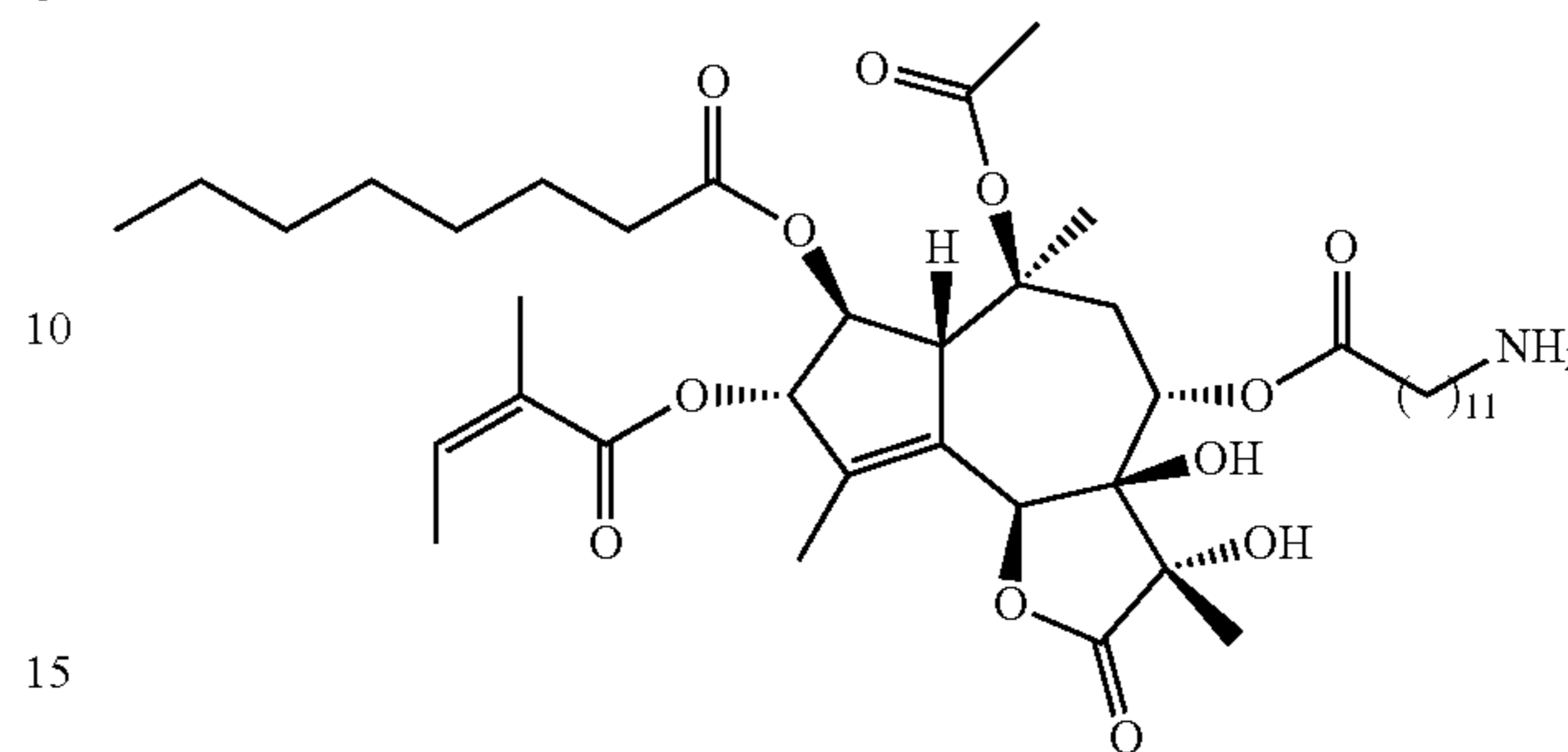
12-ADT C 42 H 67 NO 12 Mol. Wt.: 777.98 (TFA salt MW = 892.00)
