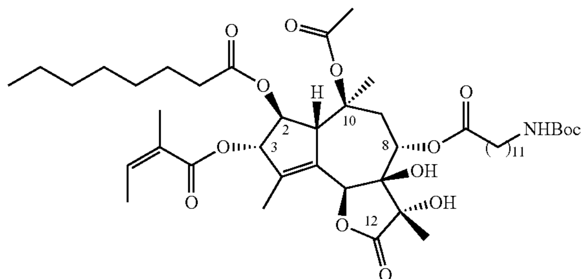
Boc-12ADT C 47 H 75 NO 14 Mol. Wt.: 878.1
