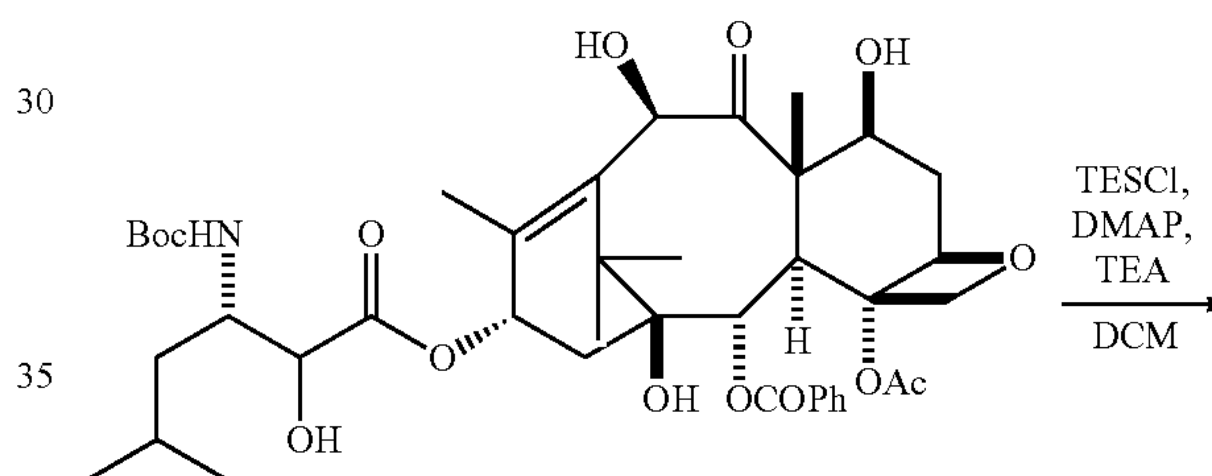
C_{41}H_{57}NO_{14} Mol. Wt.: 787.89 Formula 38
