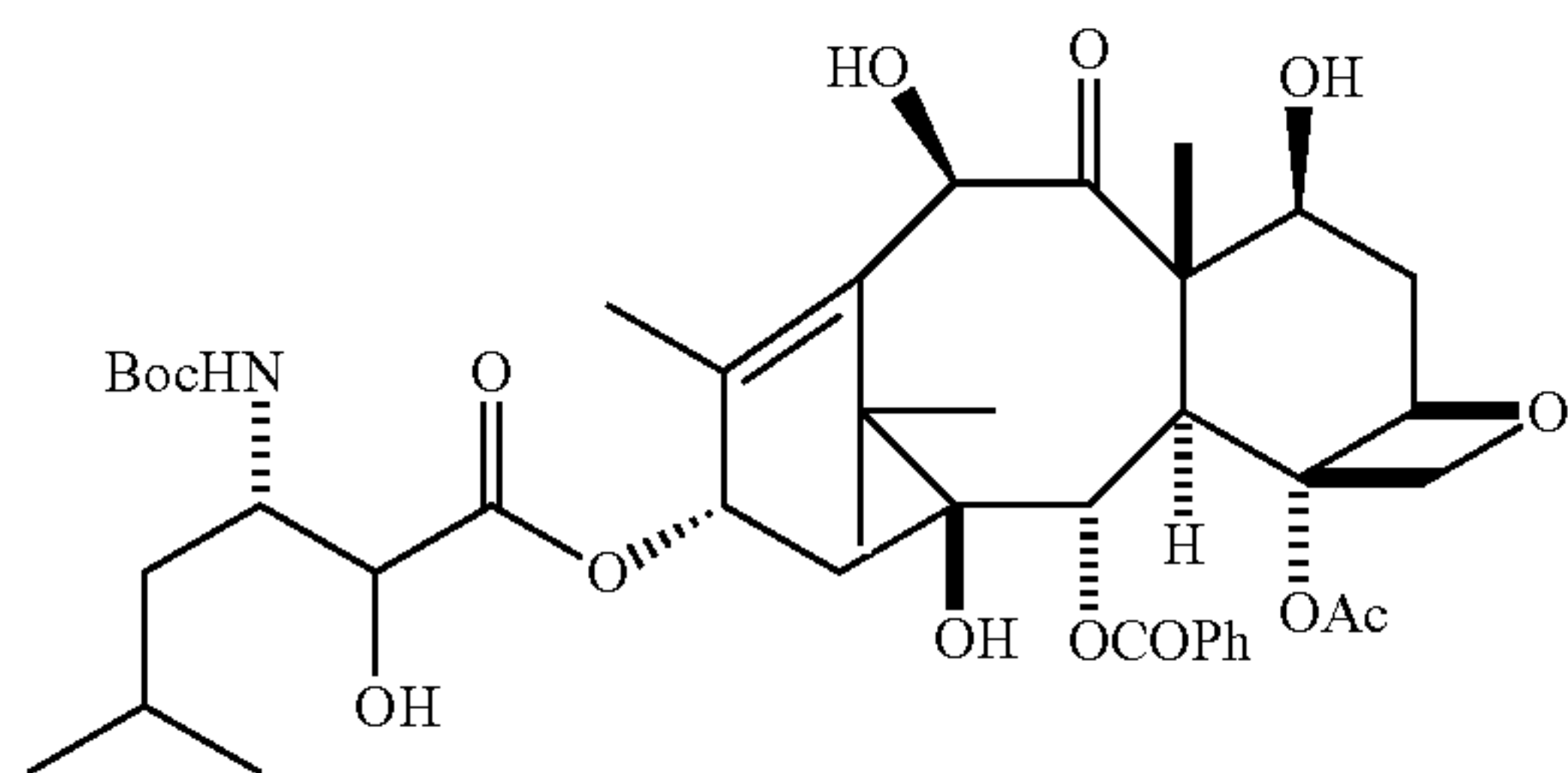
C_{41}H_{57}NO_{14} Mol. Wt.: 787.89 Formula 38
