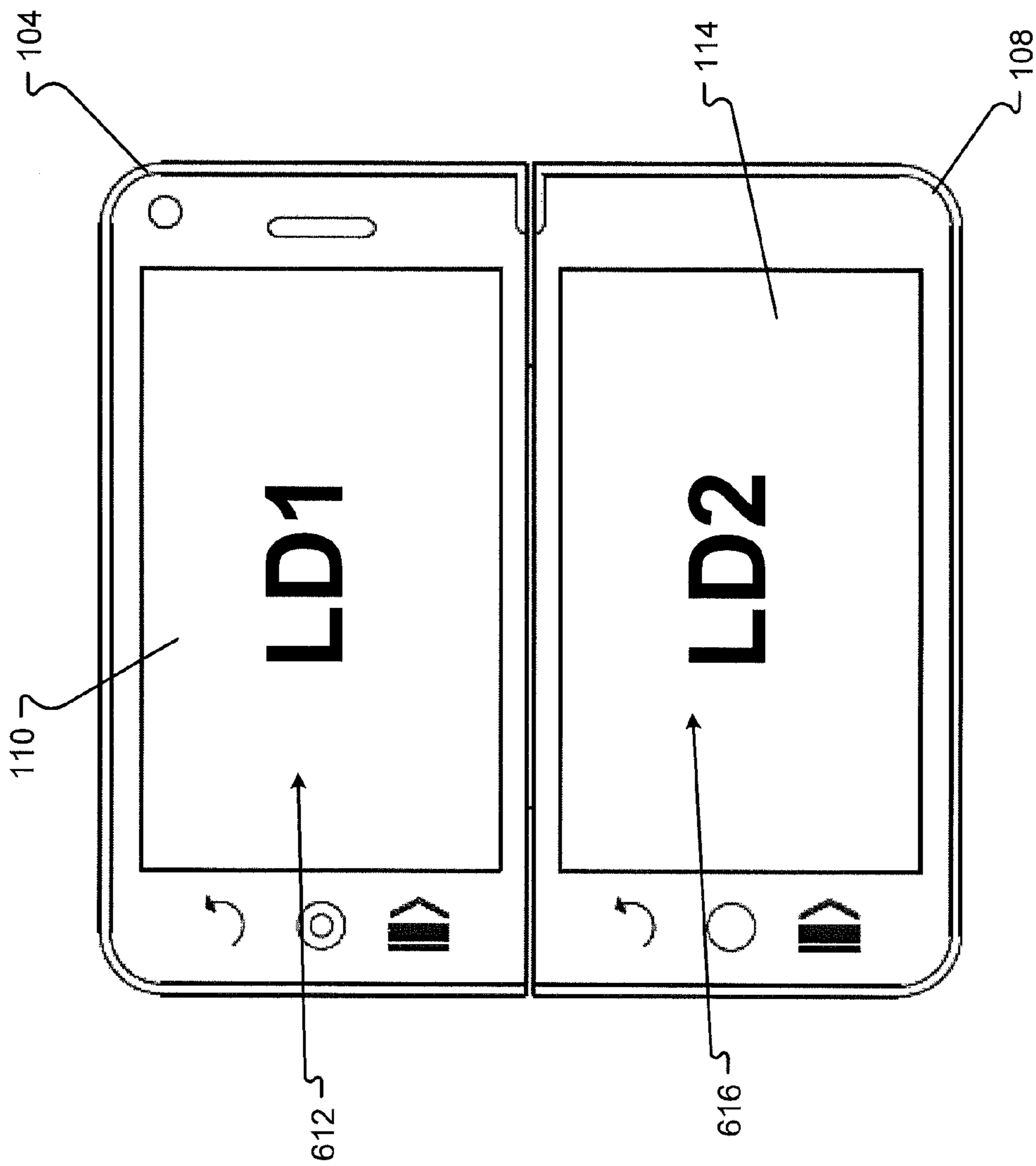
FIG. 6F
