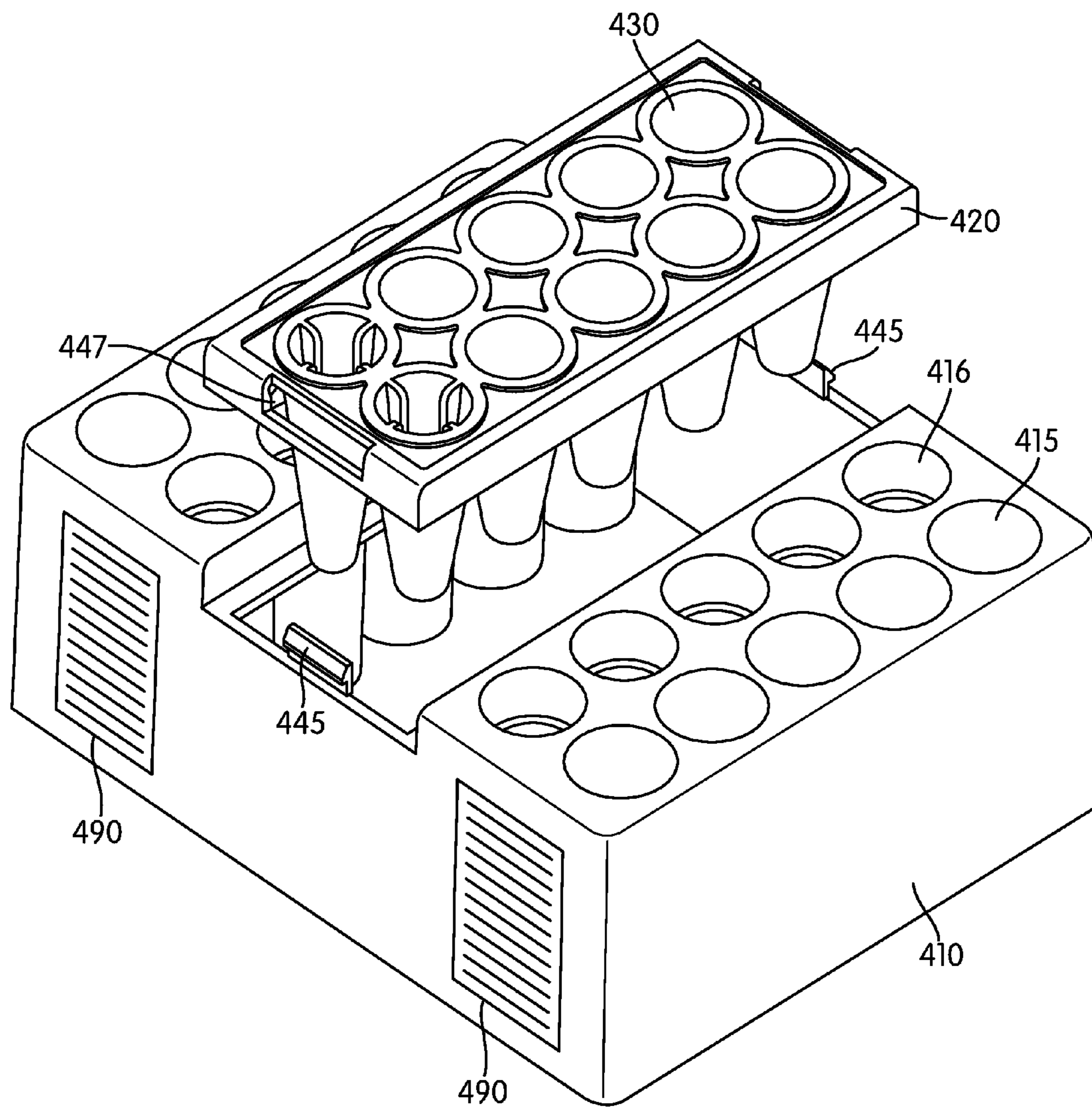
FIG. 4B
