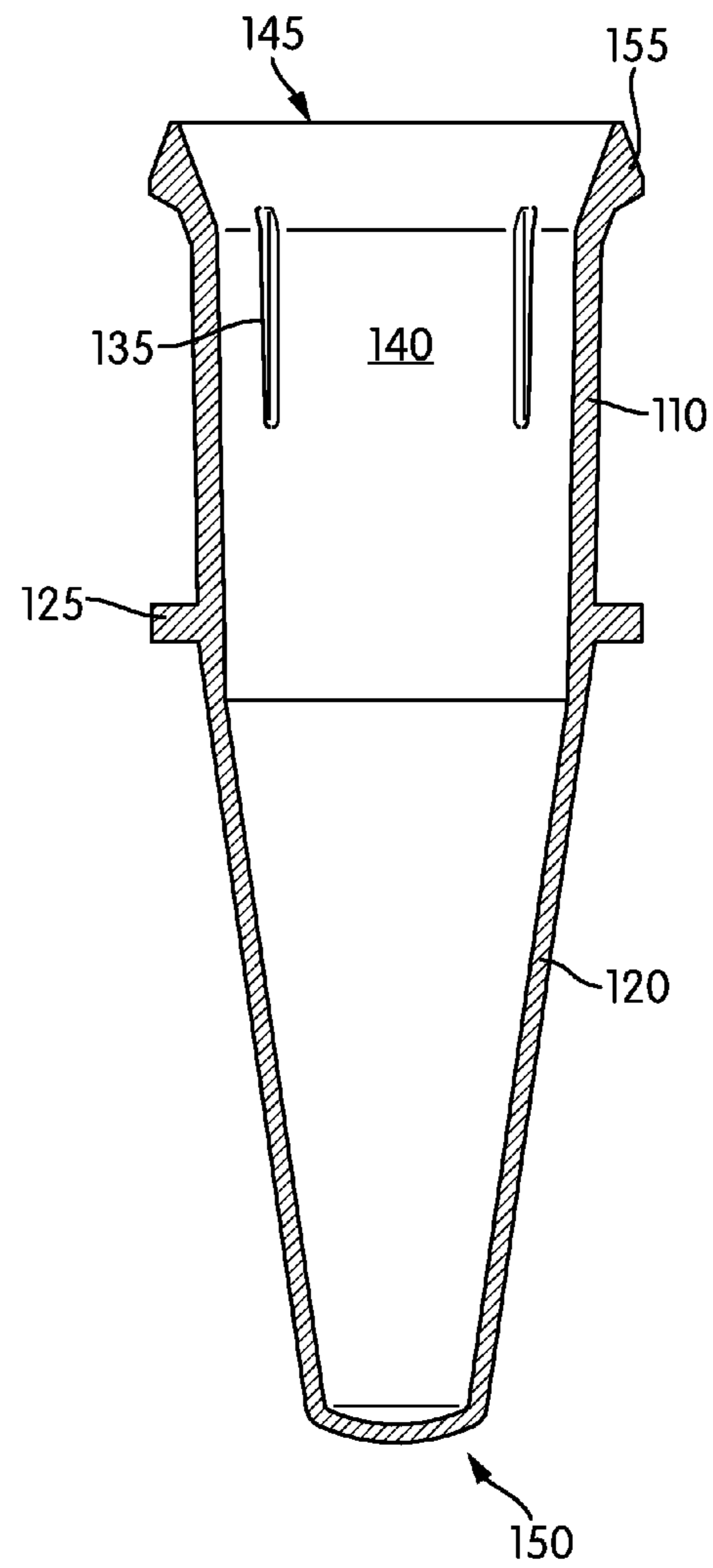
FIG. 1B
