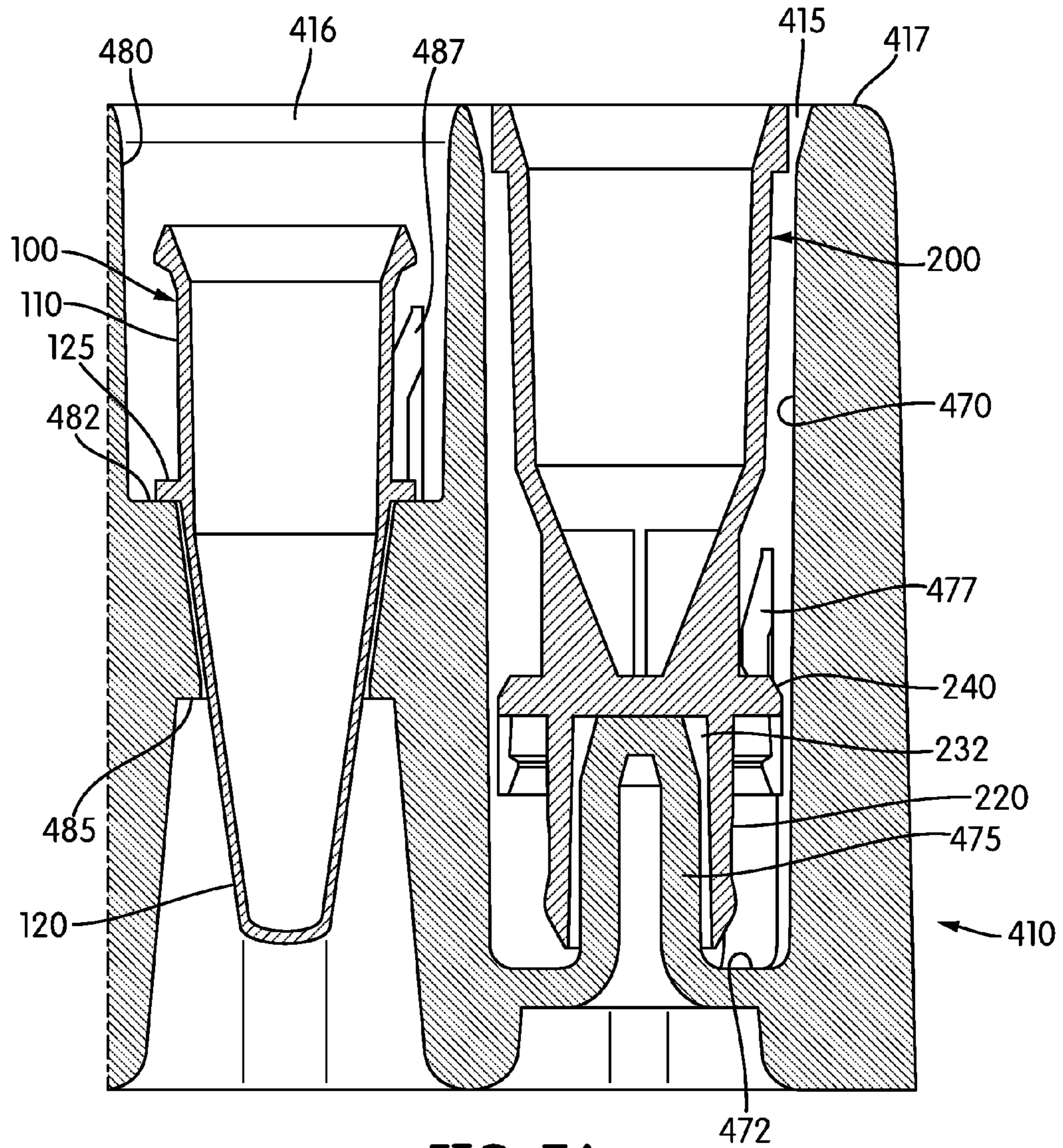
FIG. 7A
