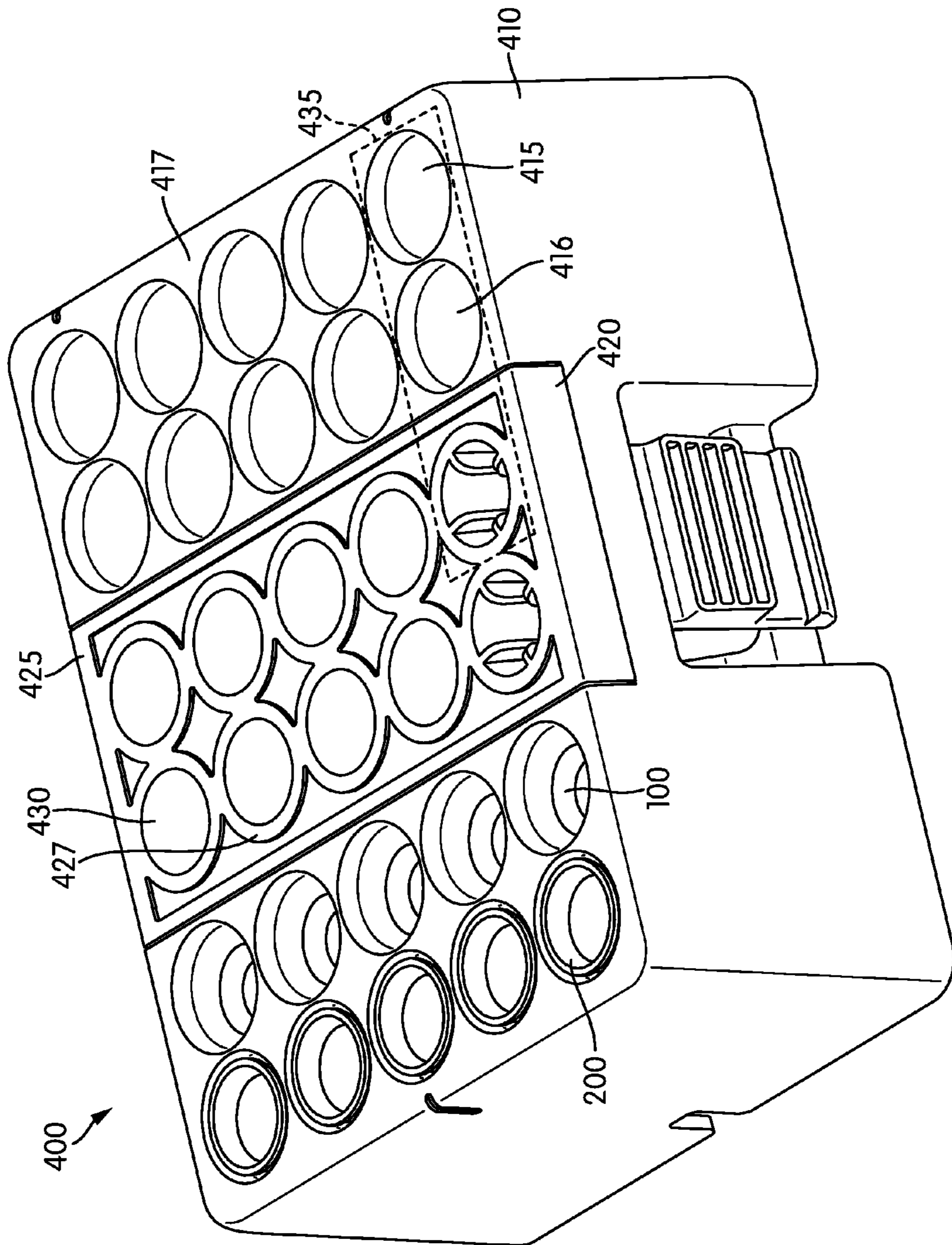
FIG. 4A
