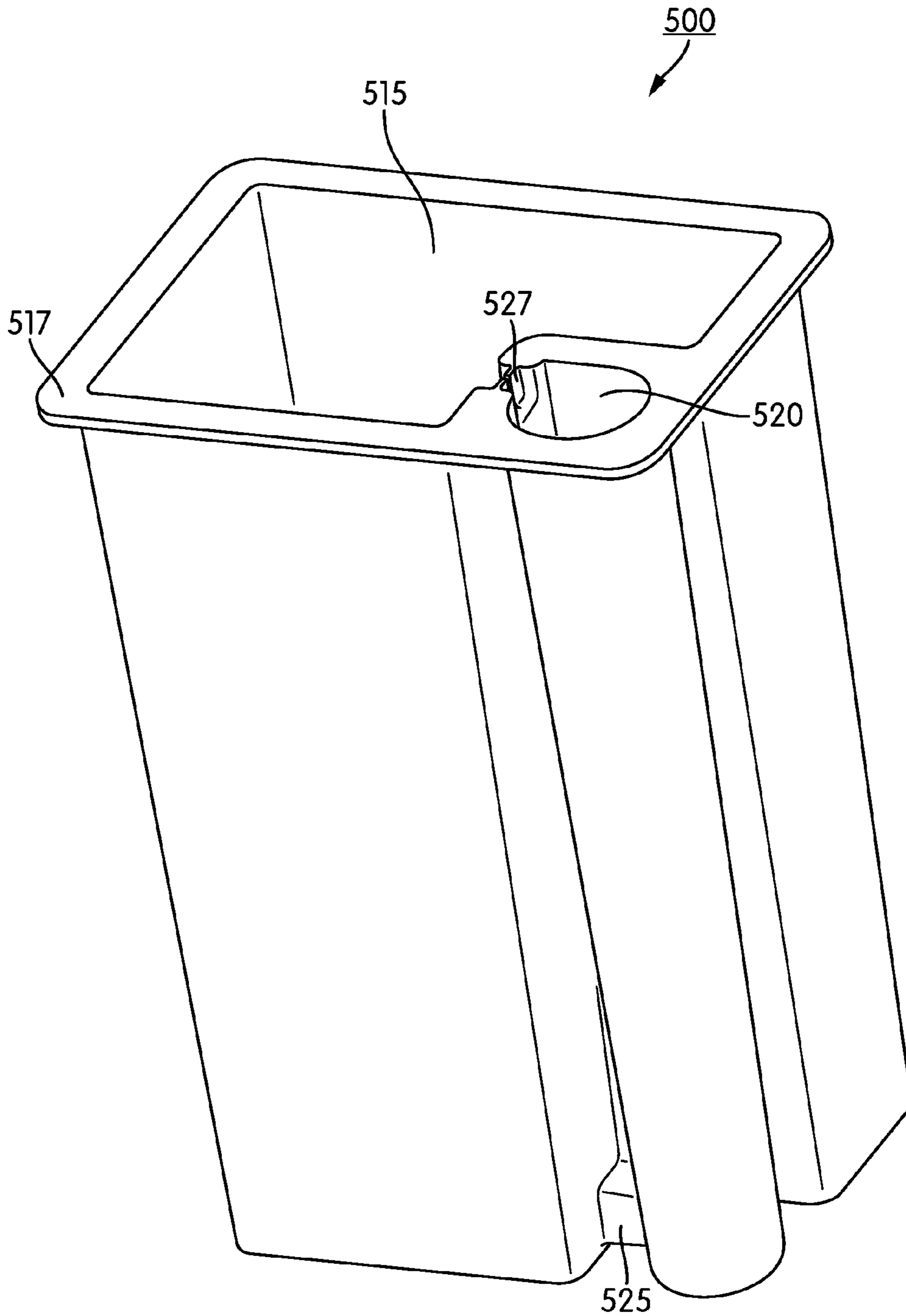
FIG. 10B
