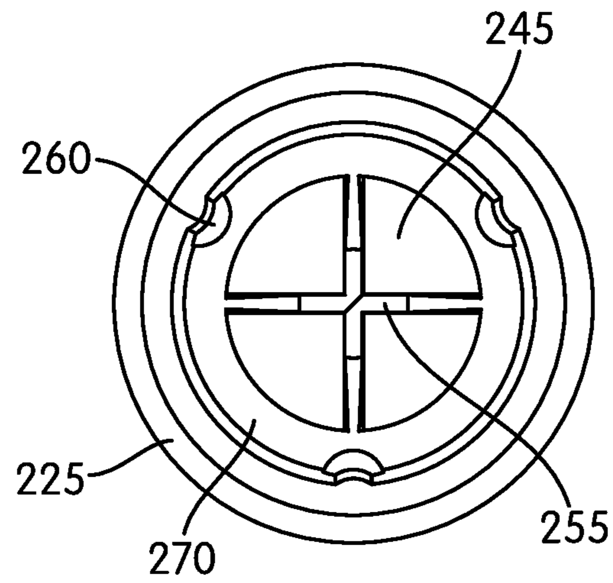
FIG. 2C
