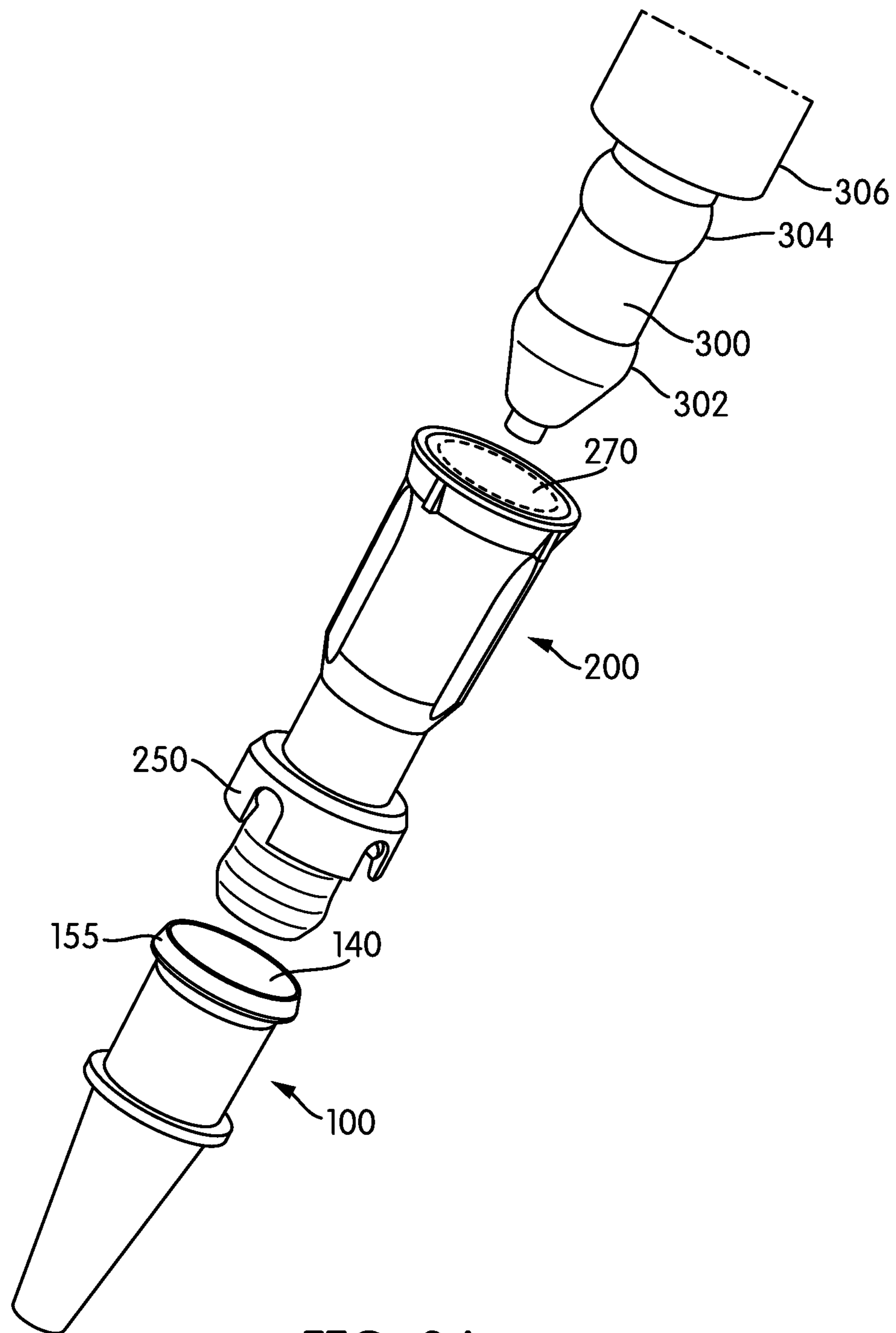
FIG. 3A
