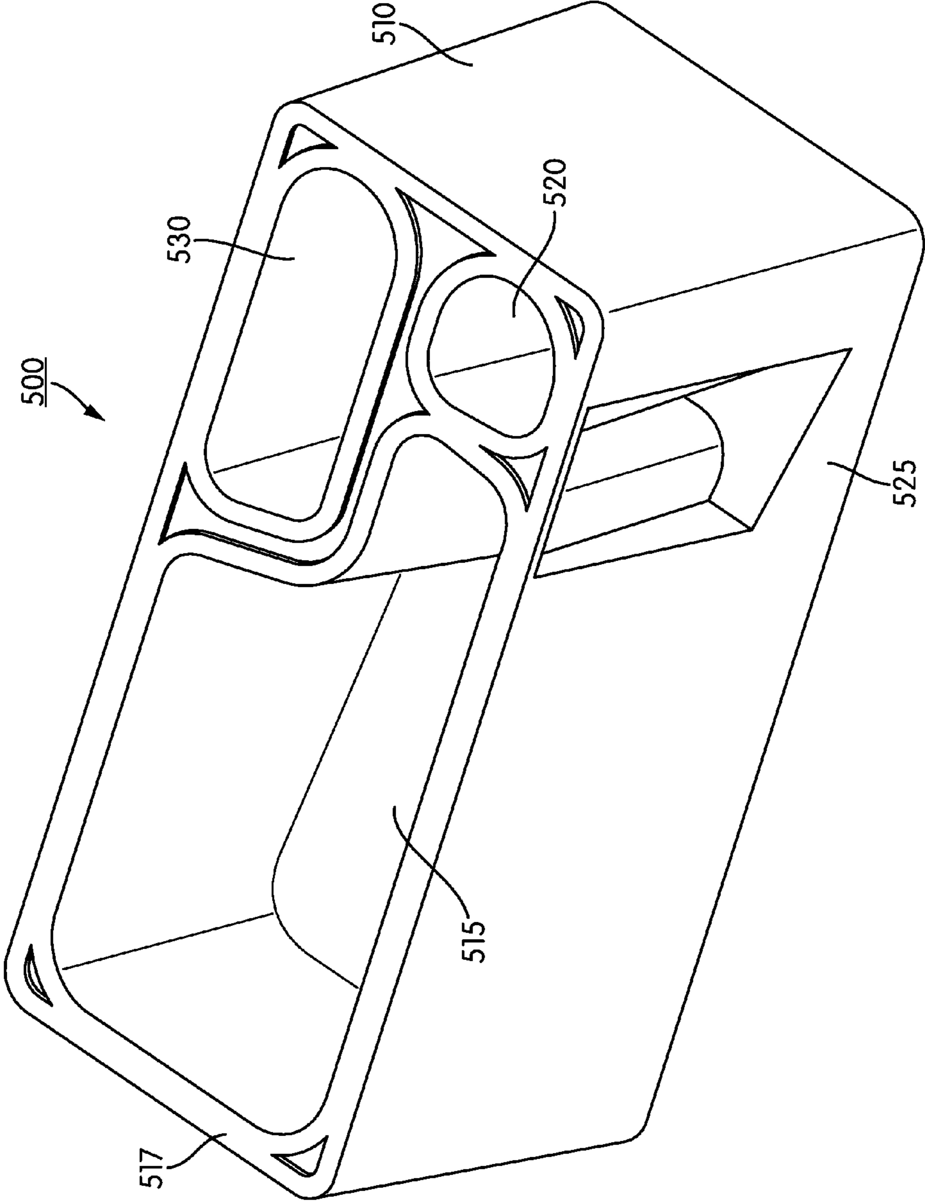
FIG. 10A
