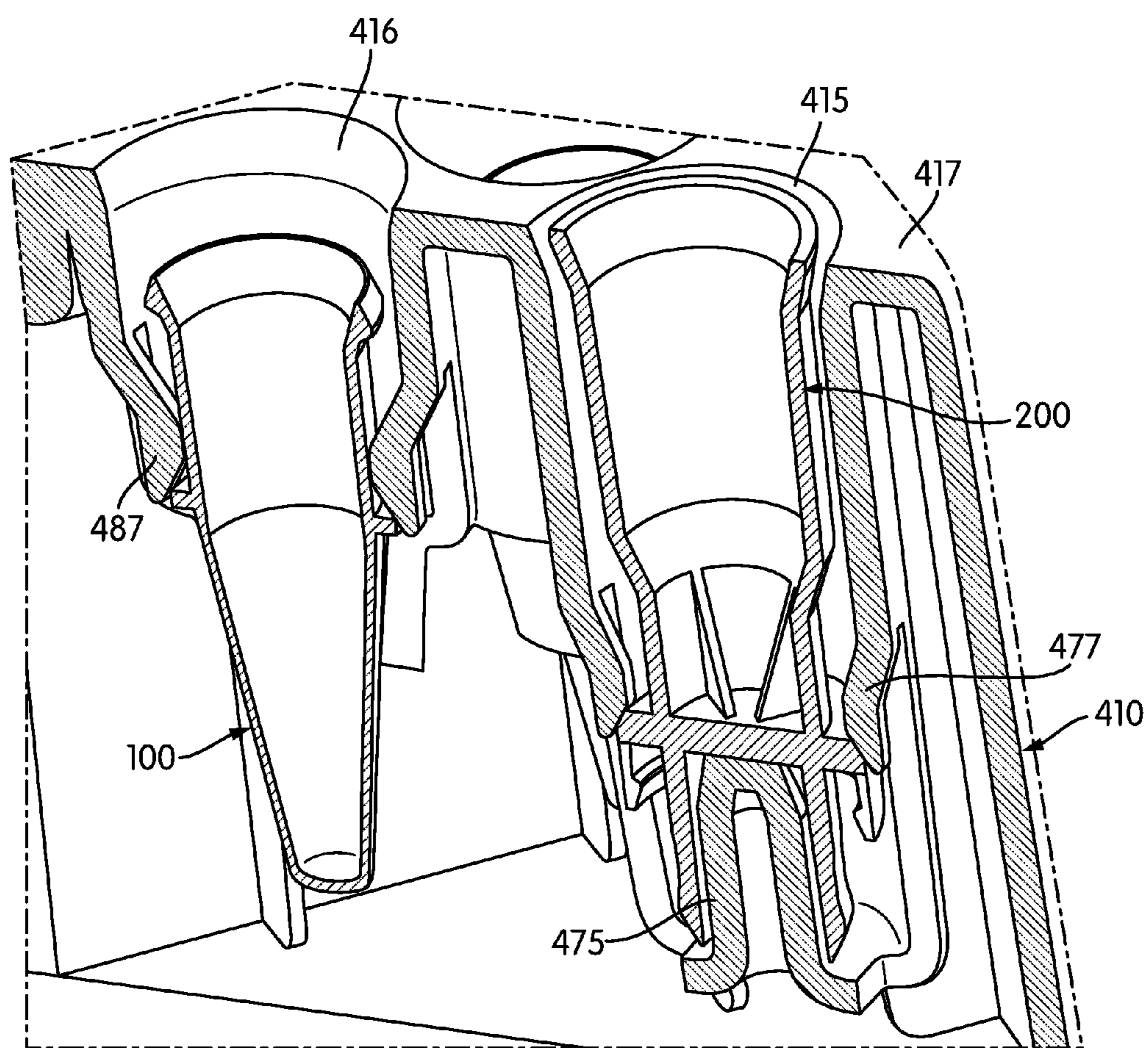
FIG. 7B
