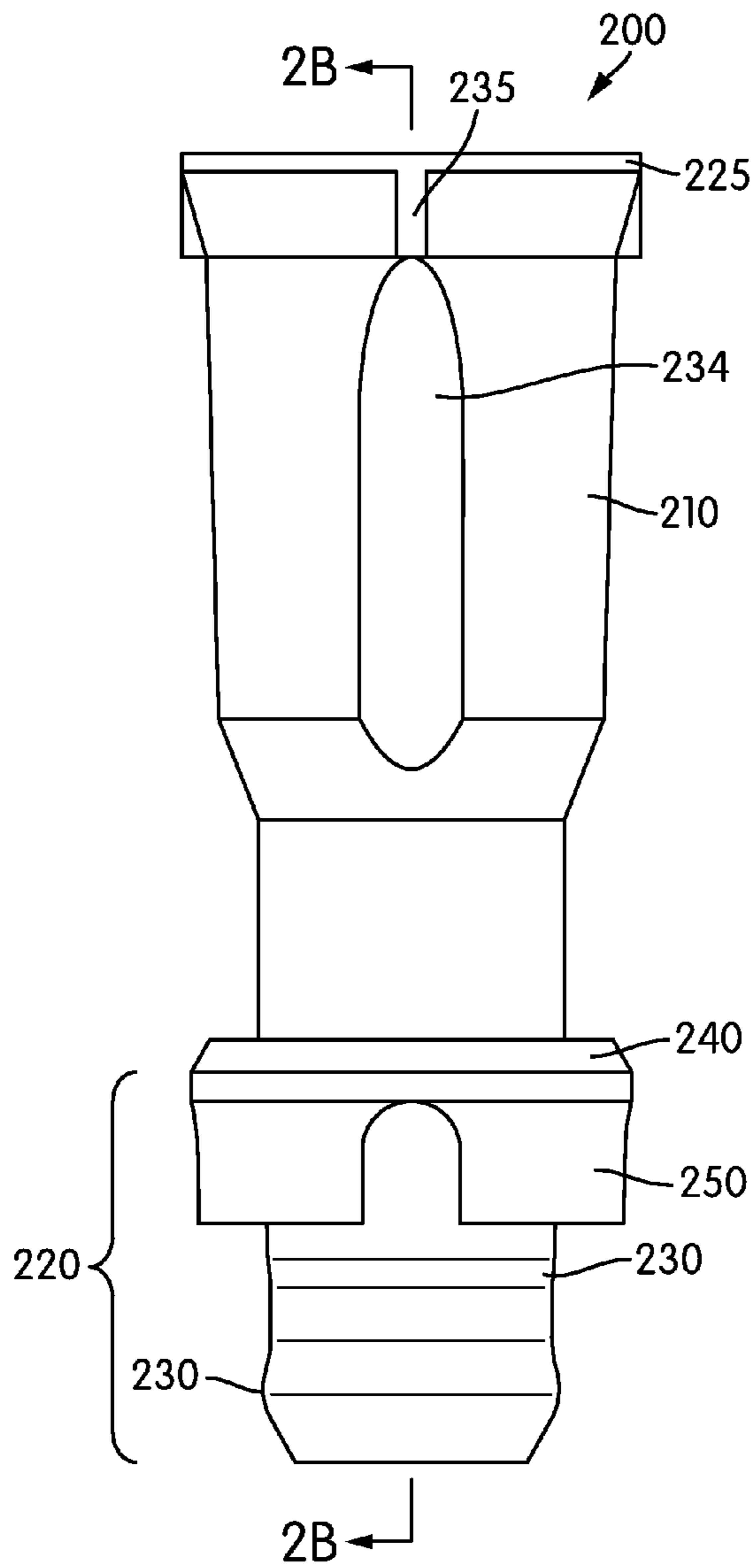
FIG. 2A
