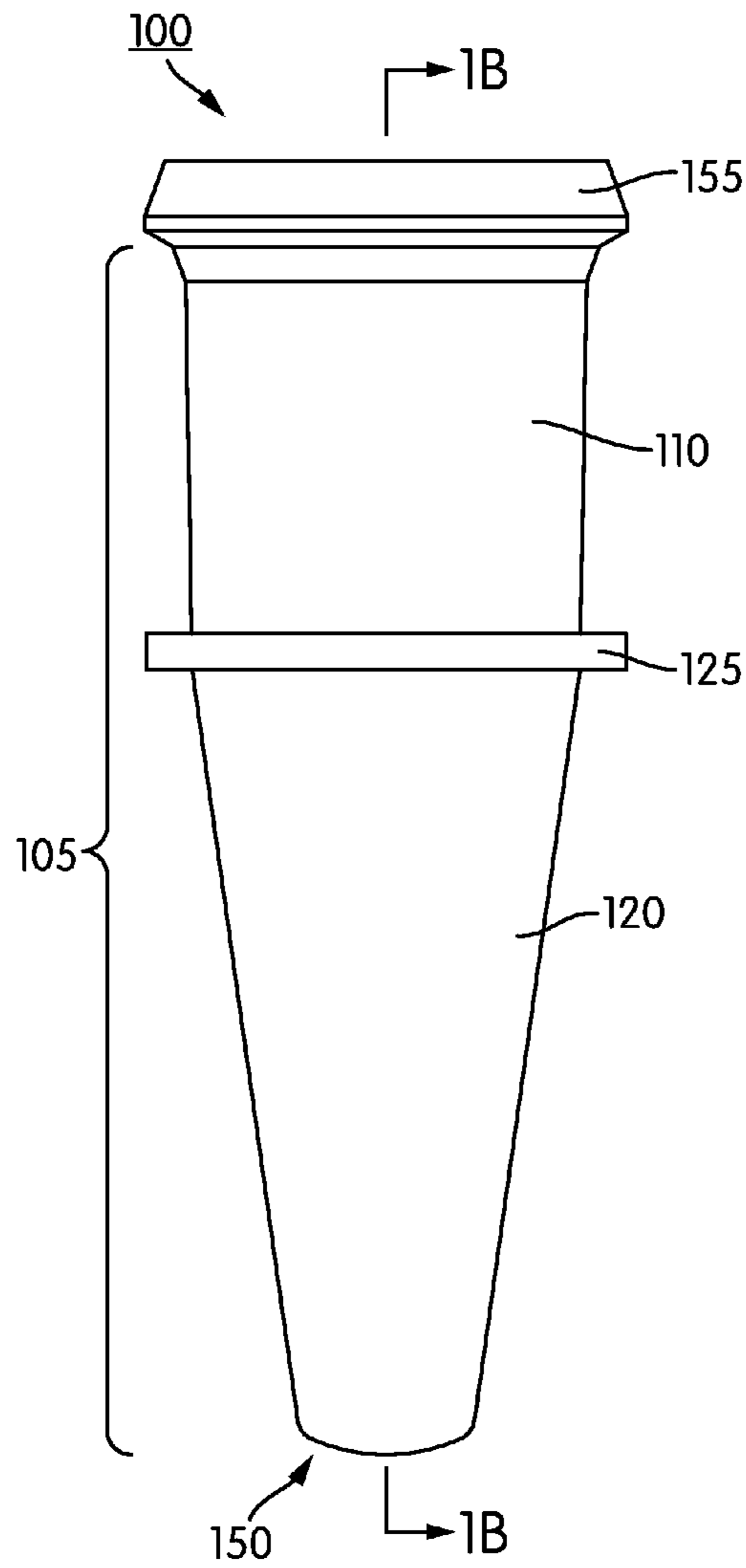
FIG. 1A
