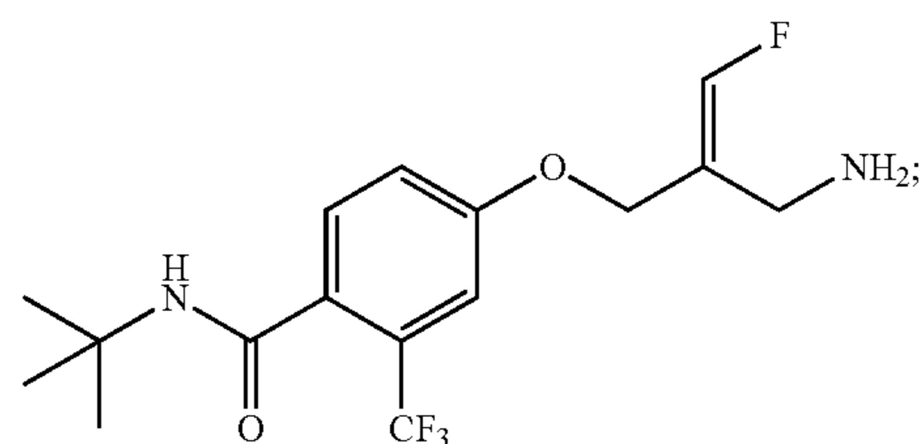
(E)-4-(2-(Aminomethyl)-3-fluoroallyloxy)-N-tert-butyl-2-(trifluoromethyl)benzamide
