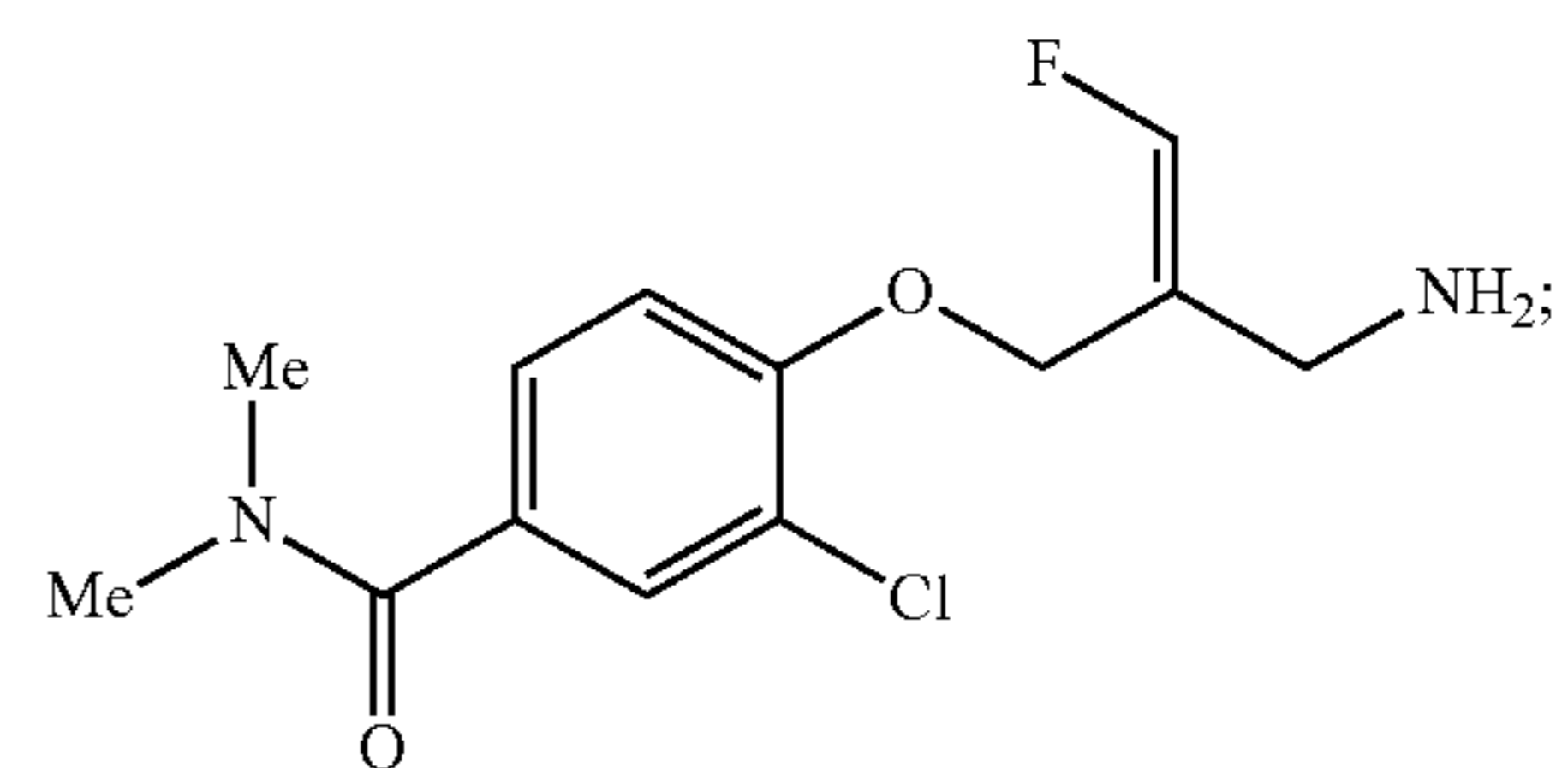
(Z)-4-(2-(Aminomethyl)-3-fluoroallyloxy)-3-chloro-N,N-dimethylbenzamide
