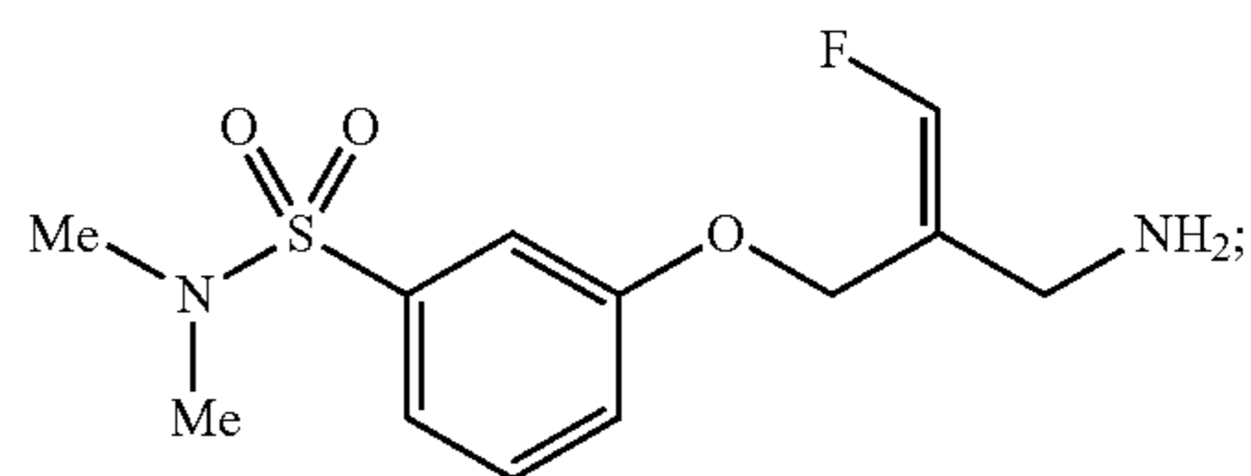
(Z)-3-(2-(Aminomethyl)-3-fluoroallyloxy)-N,N-dimethylbenzenesulfonamide
