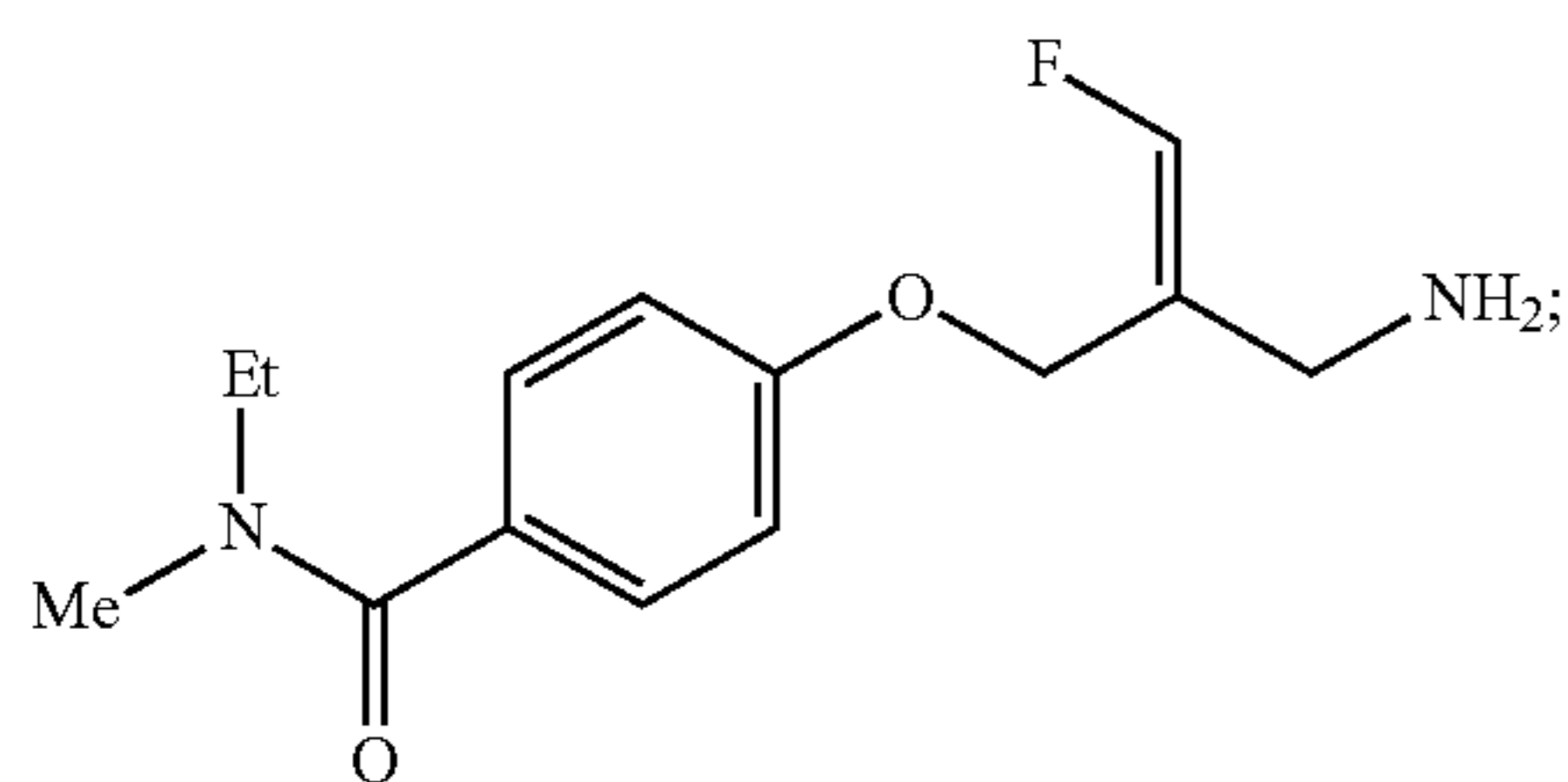
(Z)-4-(2-(Aminomethyl)-3-fluoroallyloxy)-N-ethyl-N-methylbenzamide
