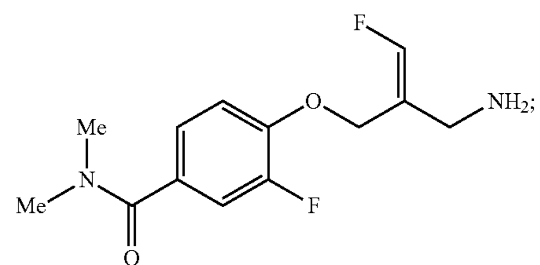
(Z)-4-(2-(Aminomethyl)-3-fluoroallyloxy)-3-fluoro-N,N-dimethylbenzamide
