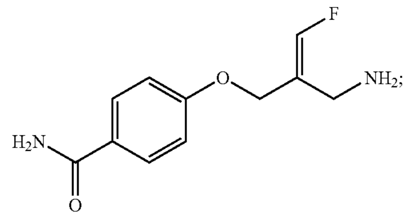
(E)-4-(2-(Aminomethyl)-3-fluoroallyloxy)benzamide
