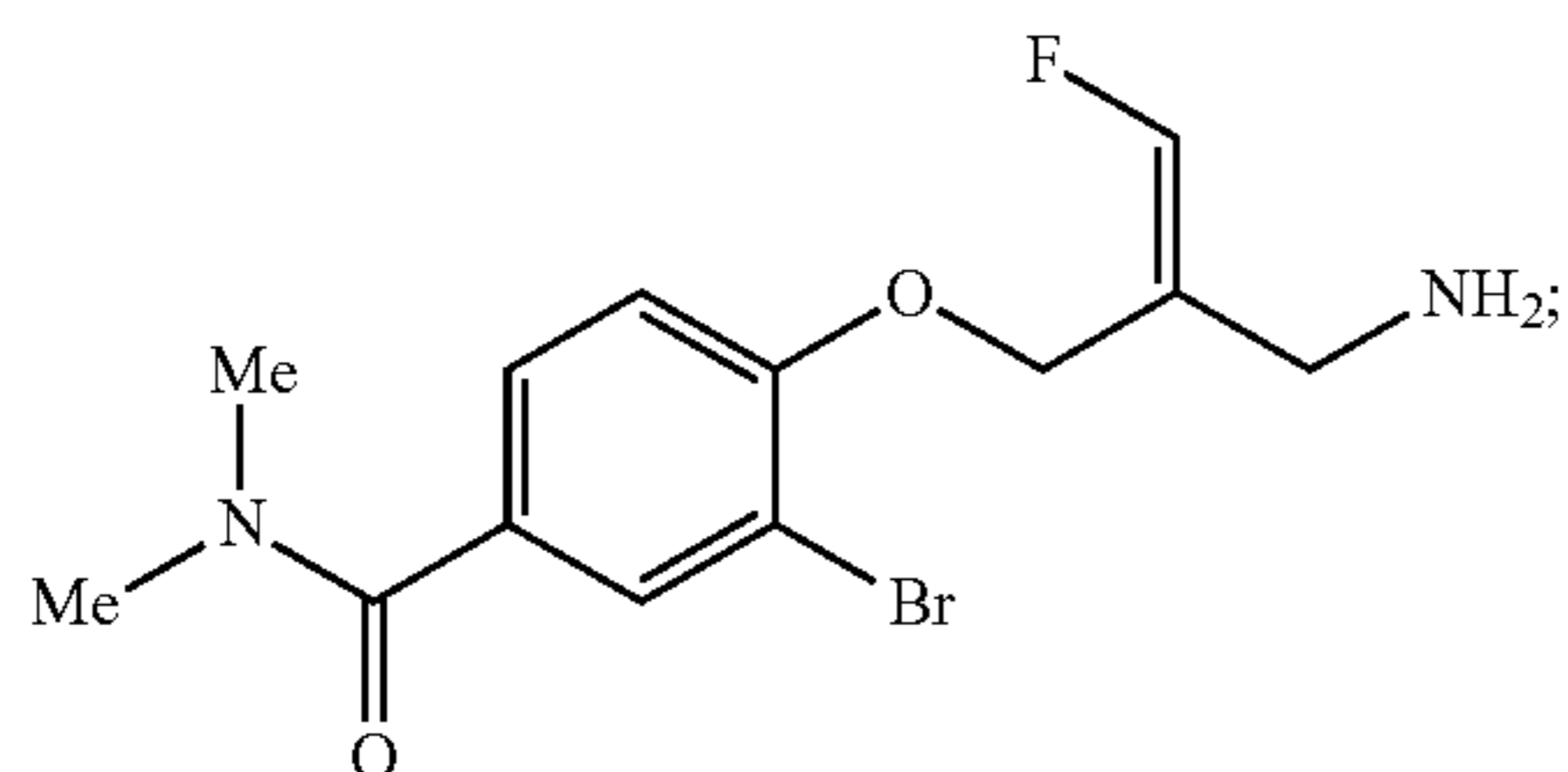
(Z)-4-(2-(Aminomethyl)-3-fluoroallyloxy)-3-bromo-N,N-dimethylbenzamide
