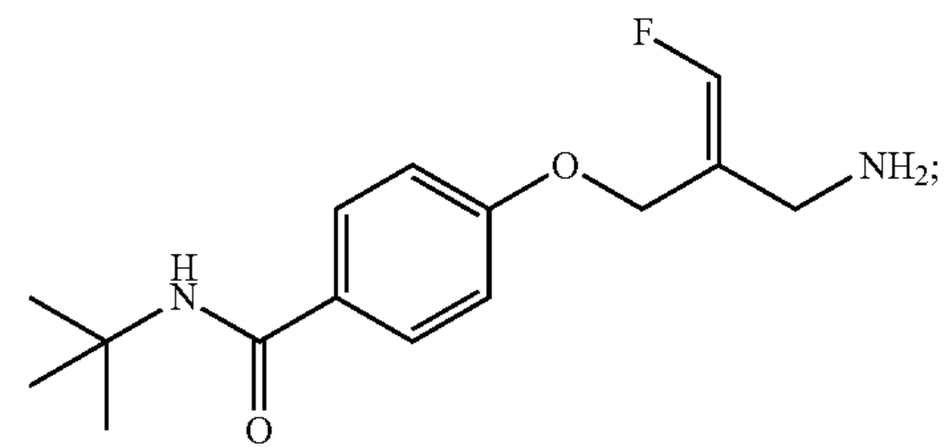
(Z)-4-(2-(Aminomethyl)-3-fluoroallyloxy)-N-tert-butylbenzamide
