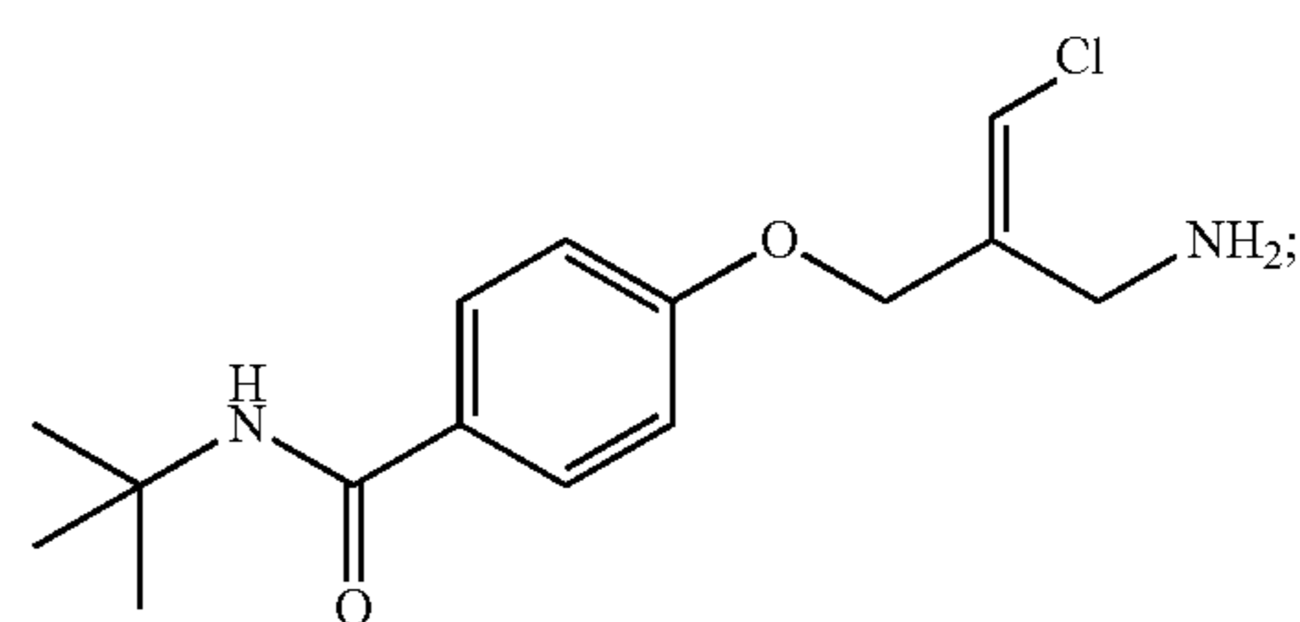
(E)-4-(2-(Aminomethyl)-3-chloroallyloxy)-N-tert-butylbenzamide
