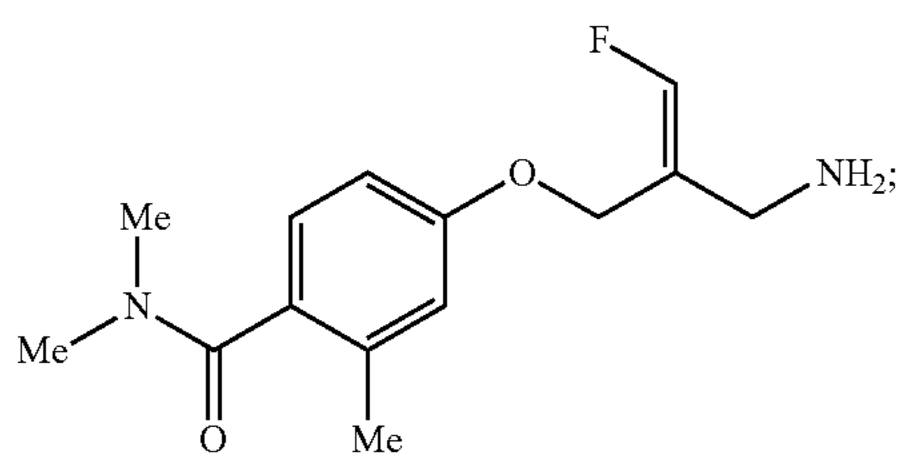
(Z)-4-(2-(Aminomethyl)-3-fluoroallyloxy)-N,N,2-trimethylbenzenamide
