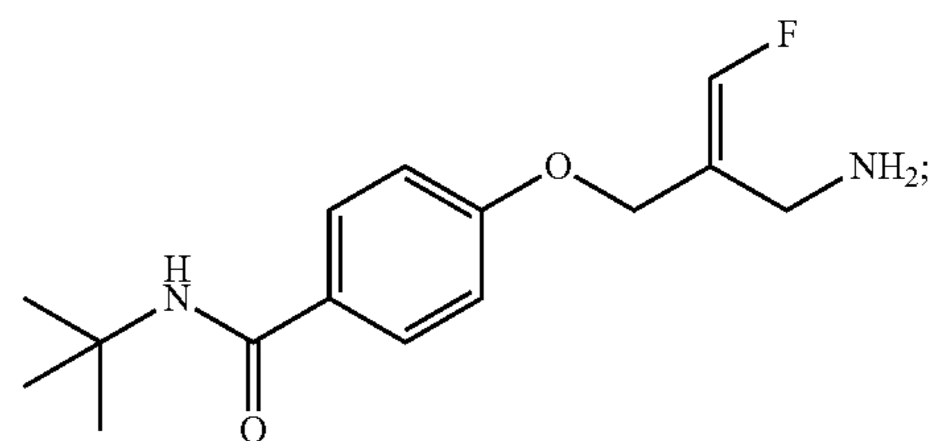
(E)-4-(2-(Aminomethyl)-3-fluoroallyloxy)-N-tert-butylbenzamide
