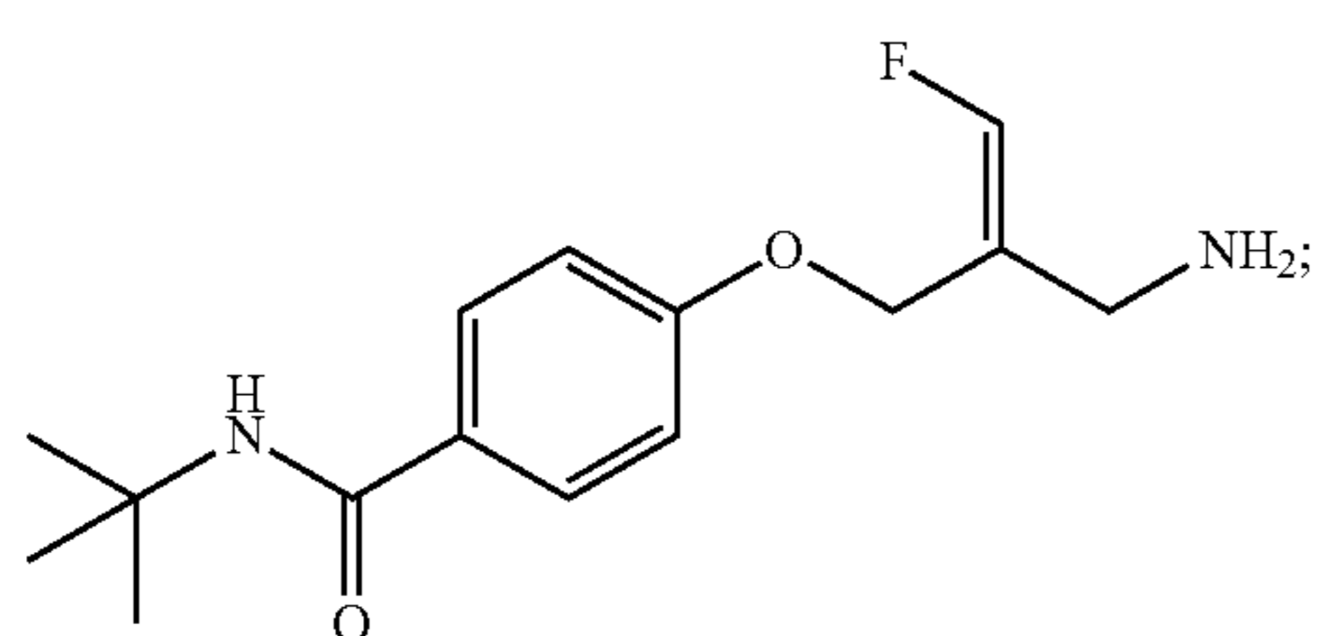
(Z)-4-(2-(Aminomethyl)-3-fluoroallyloxy)-N-tert-butylbenzamide
