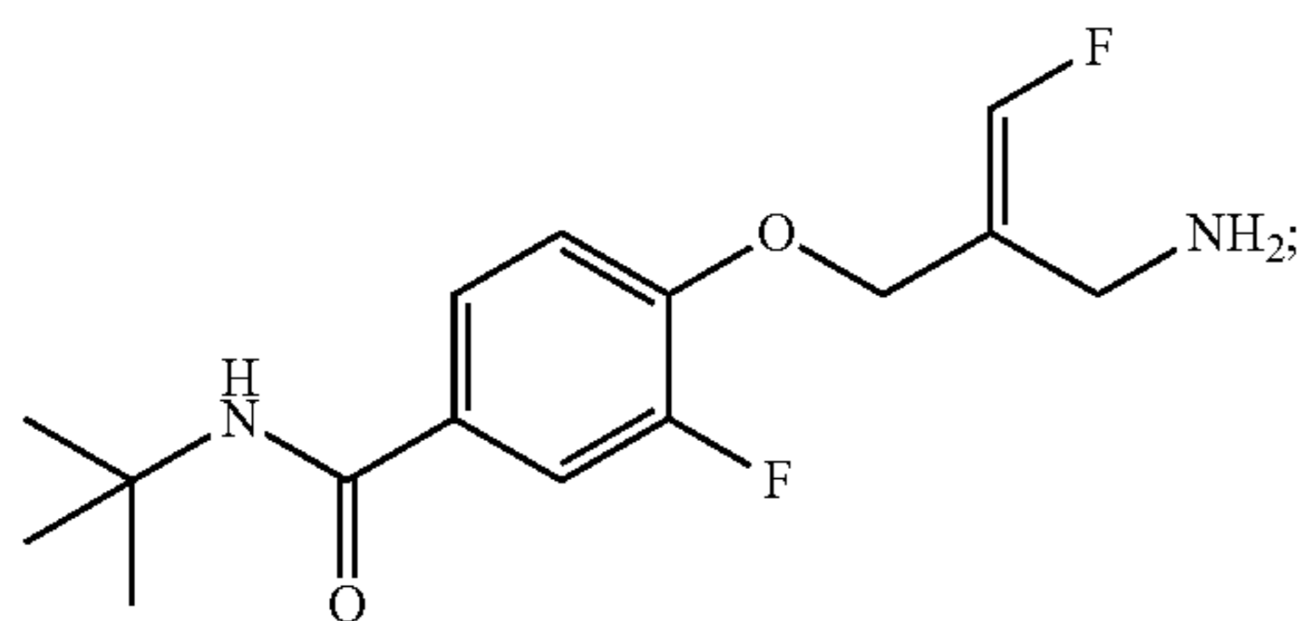
(E)-4-(2-(Aminomethyl)-3-fluoroallyloxy)-N-tert-butyl-3-fluorobenzamide
