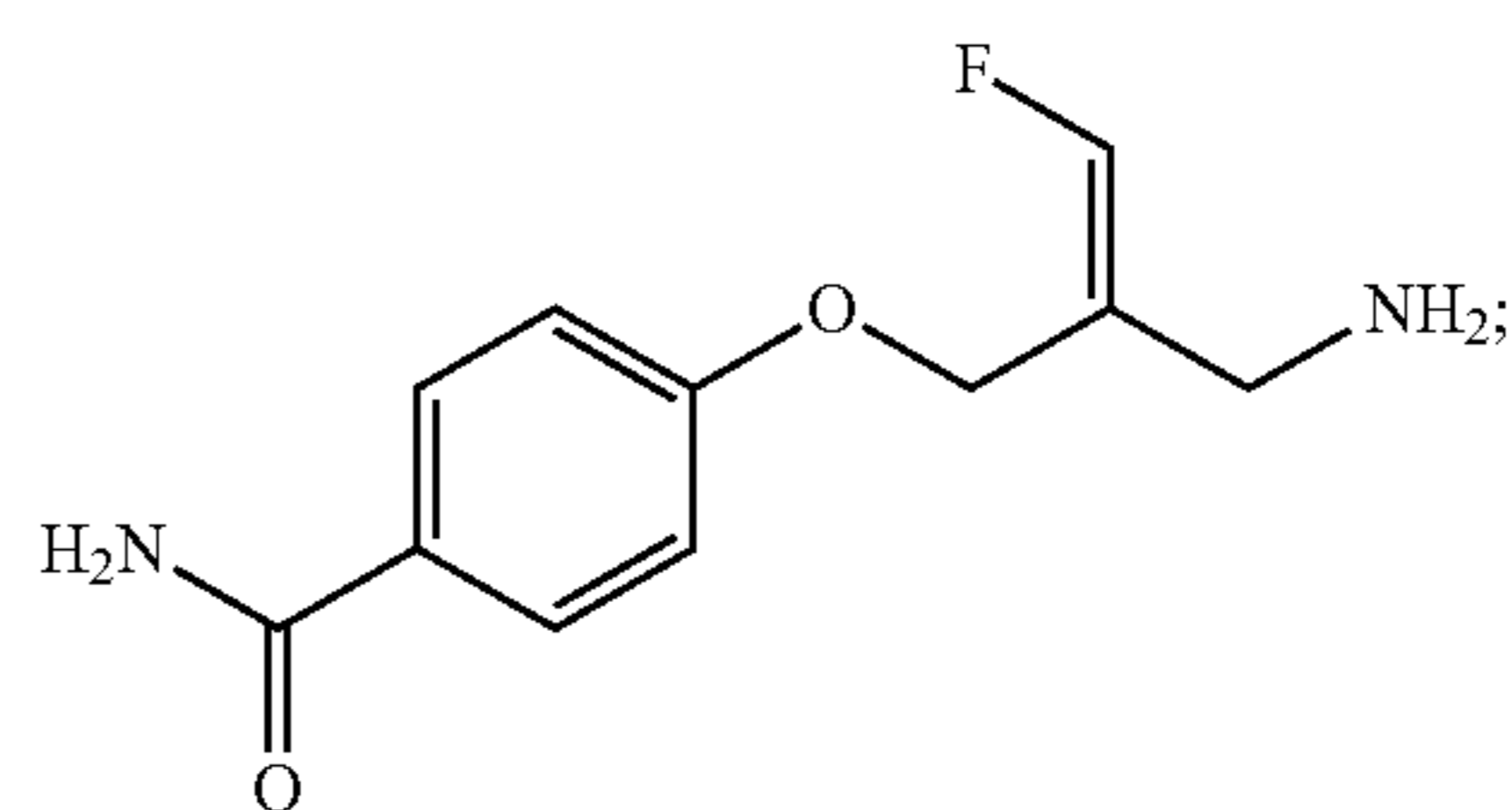
(Z)-4-(2-(Aminomethyl)-3-fluoroallyloxy)benzamide
