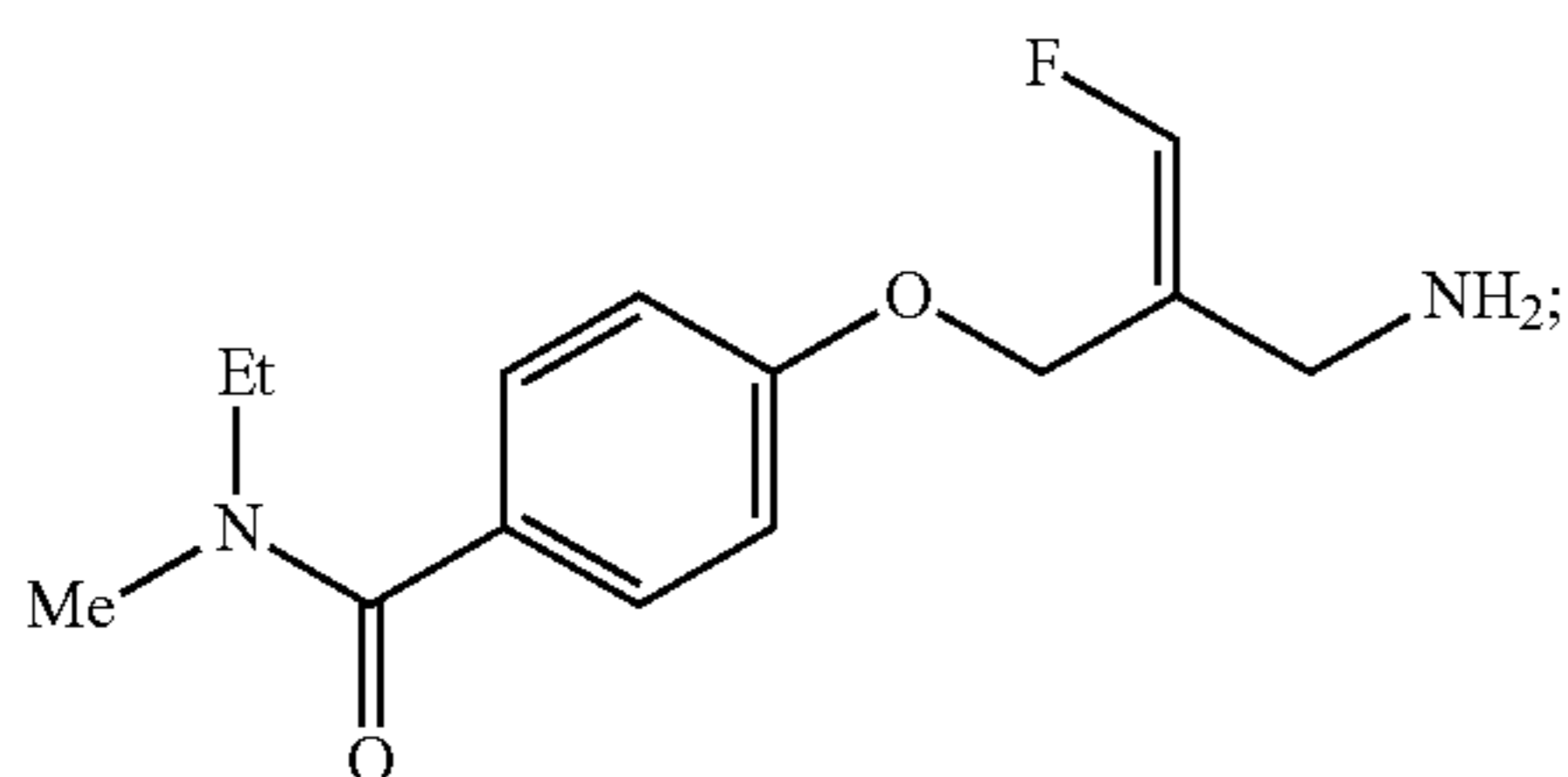
(Z)-4-(2-(Aminomethyl)-3-fluoroallyloxy)-N-ethyl-N-methylbenzamide
