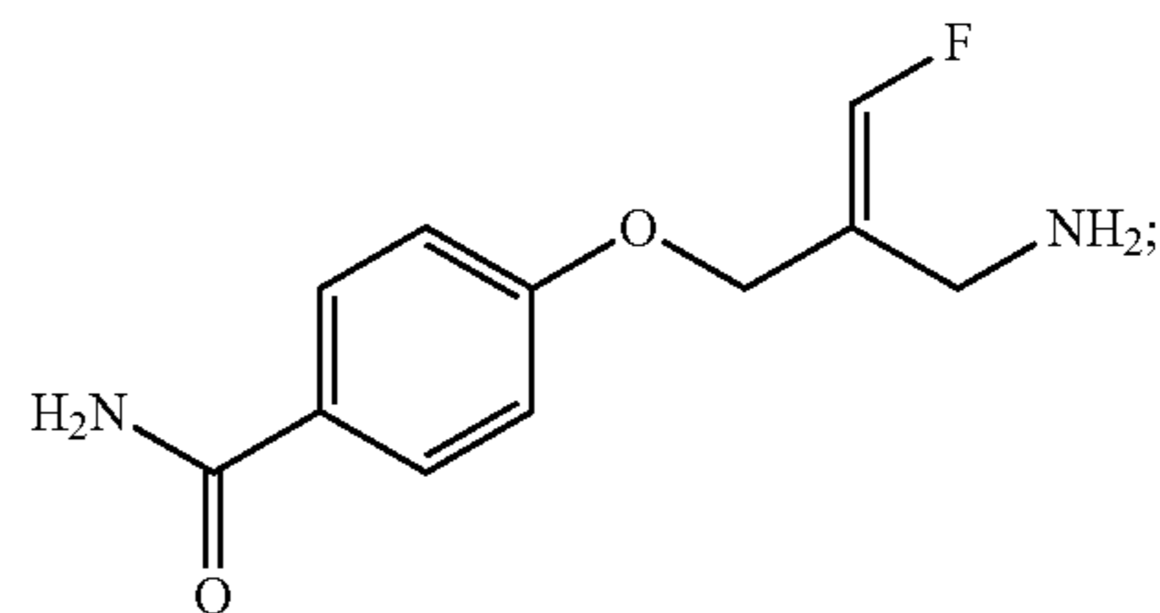
(E)-4-(2-(Aminomethyl)-3-fluoroallyloxy)benzamide
