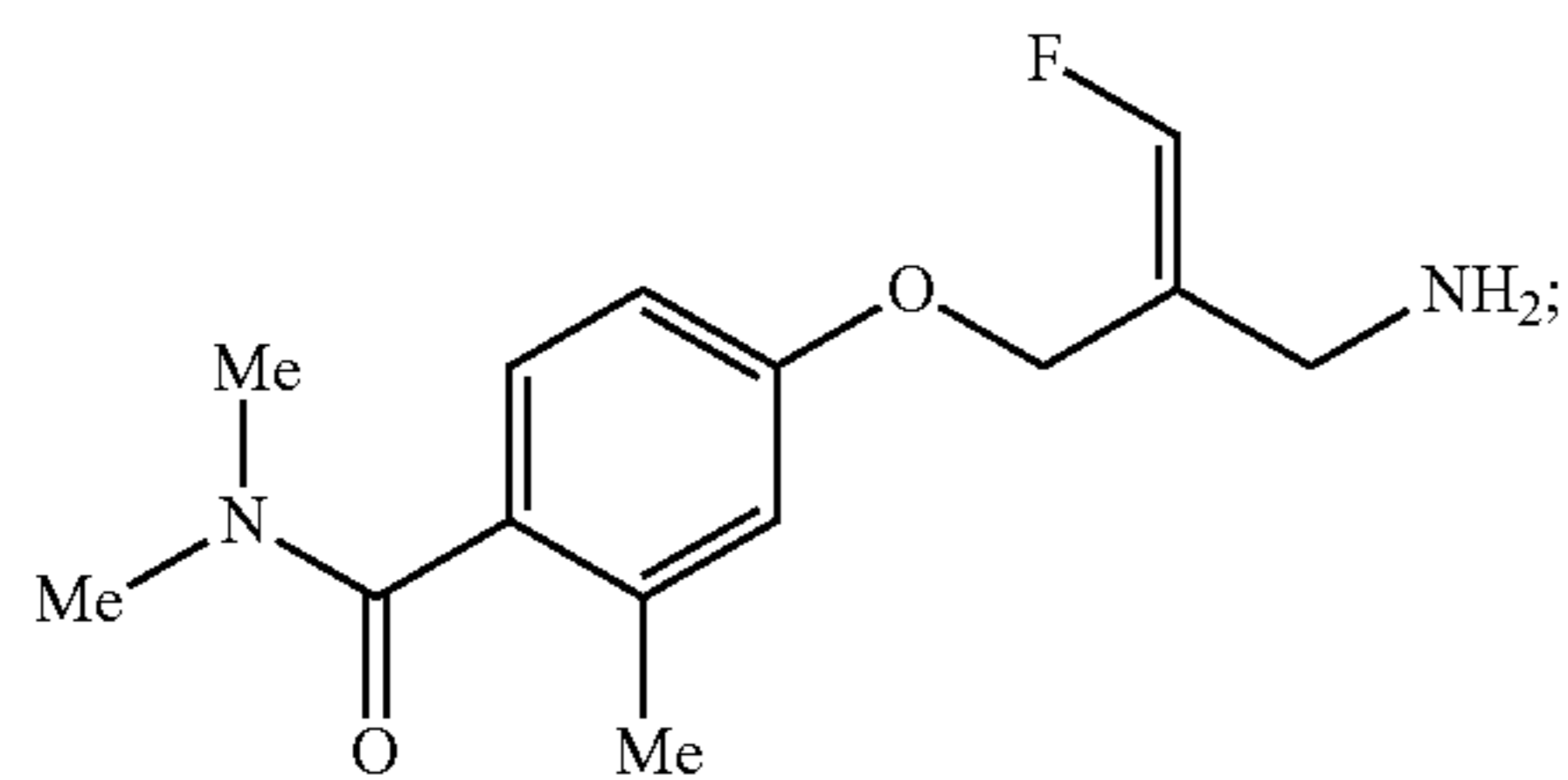
(Z)-4-(2-(Aminomethyl)-3-fluoroallyloxy)-N,N,2-trimethylbenzamide
