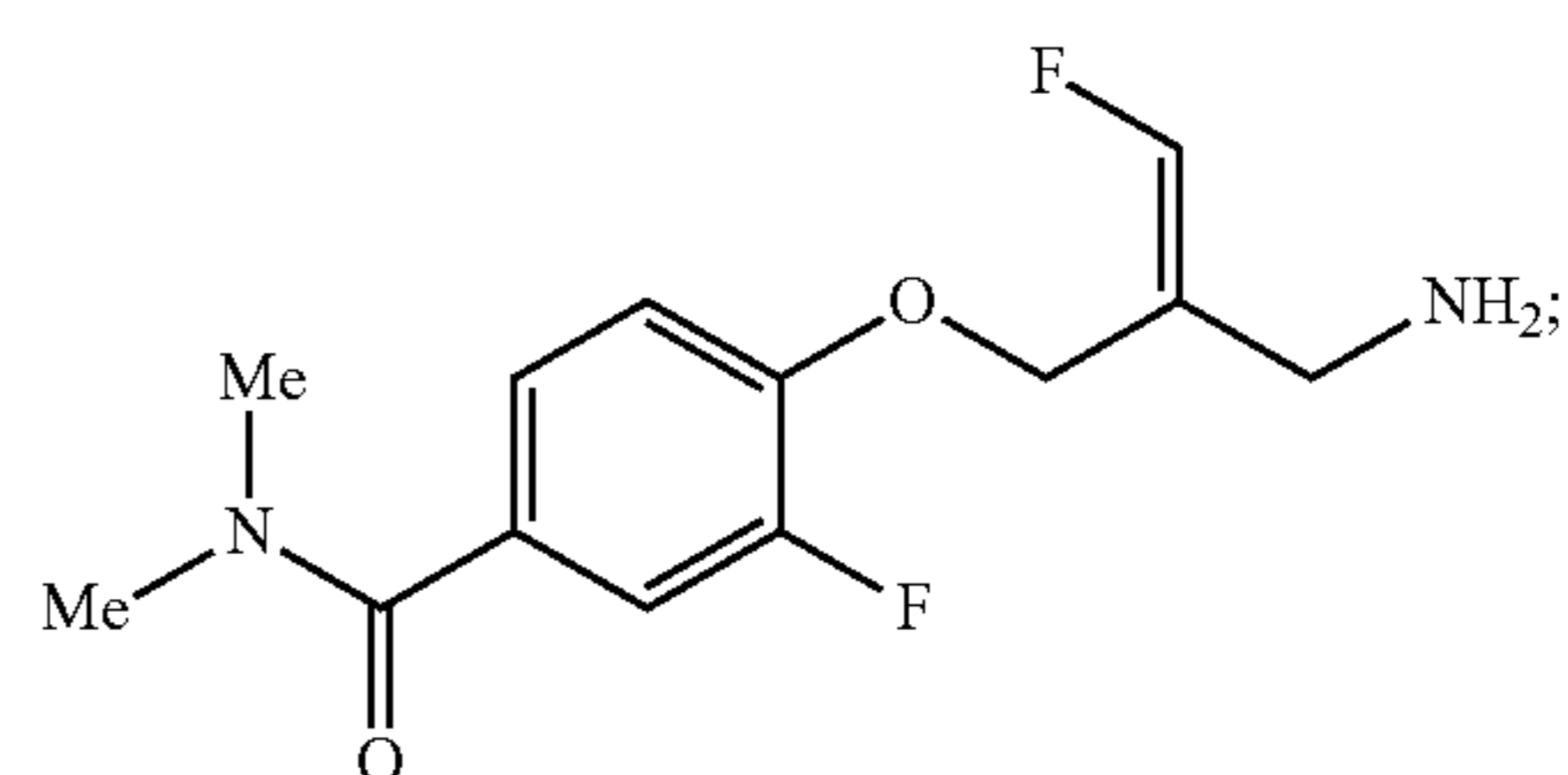
(Z)-4-(2-(Aminomethyl)-3-fluoroallyloxy)-3-fluoro-N,N-dimethylbenzamide
