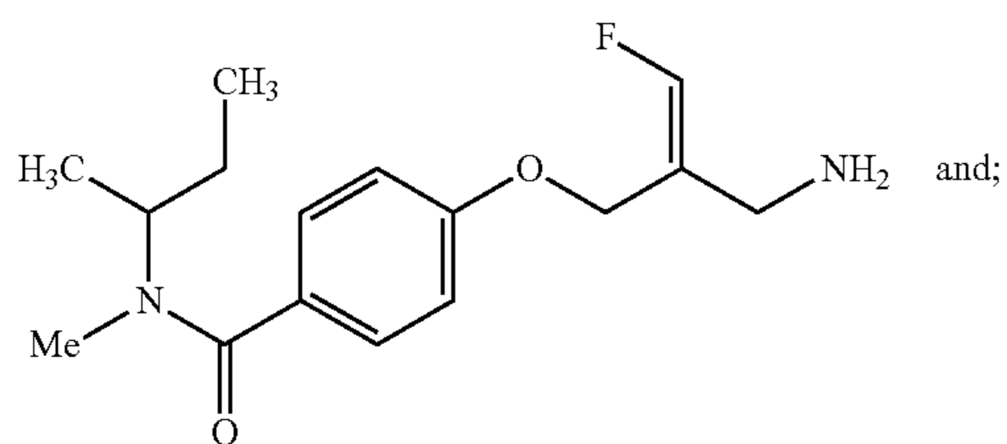
(Z)-4-(2-(Aminomethyl)-3-fluoroallyloxy)-N-sec-butyl-N-methylbenzamide
