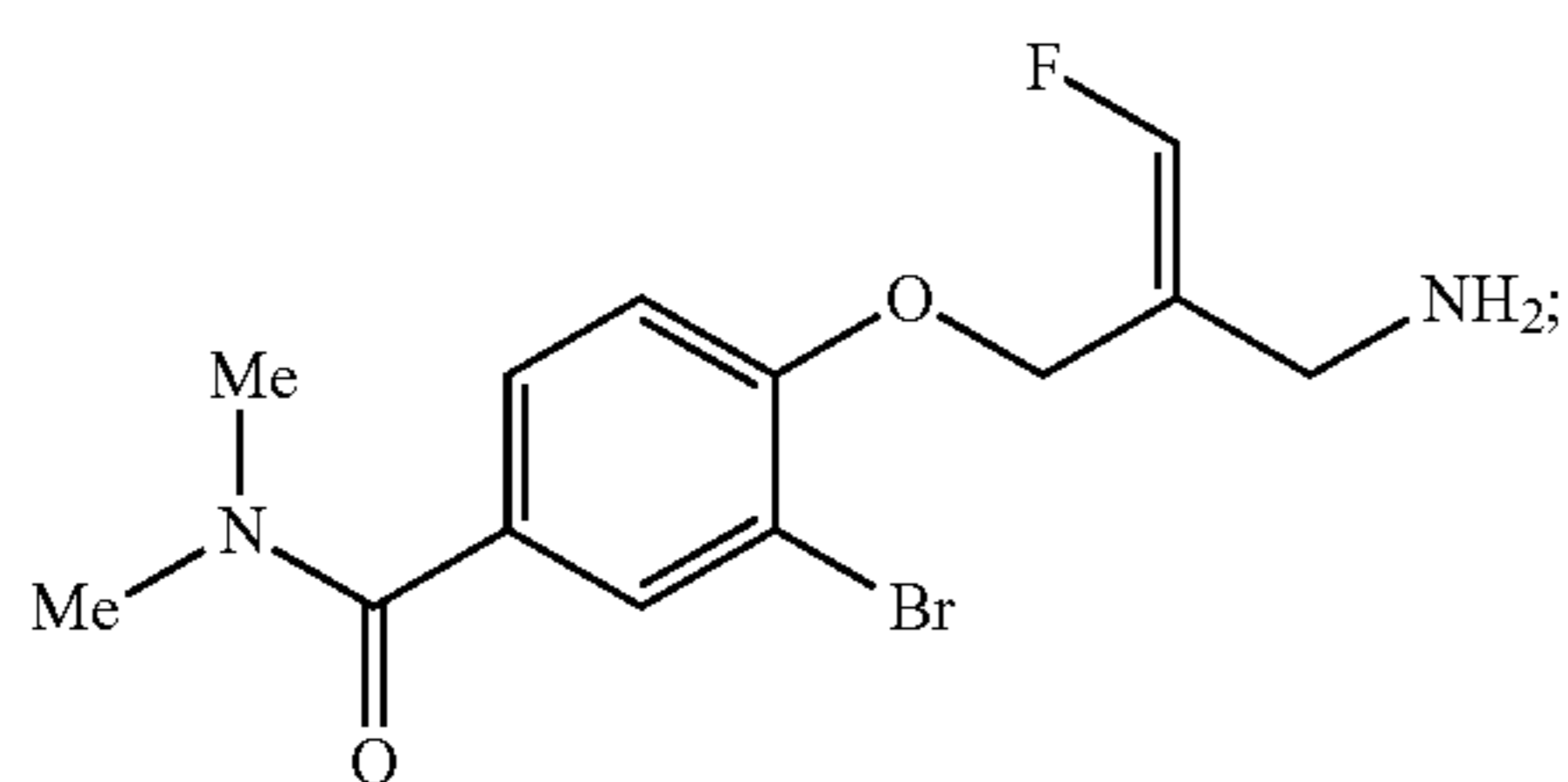
(Z)-4-(2-(Aminomethyl)-3-fluoroallyloxy)-3-bromo-N,N-dimethylbenzamide
