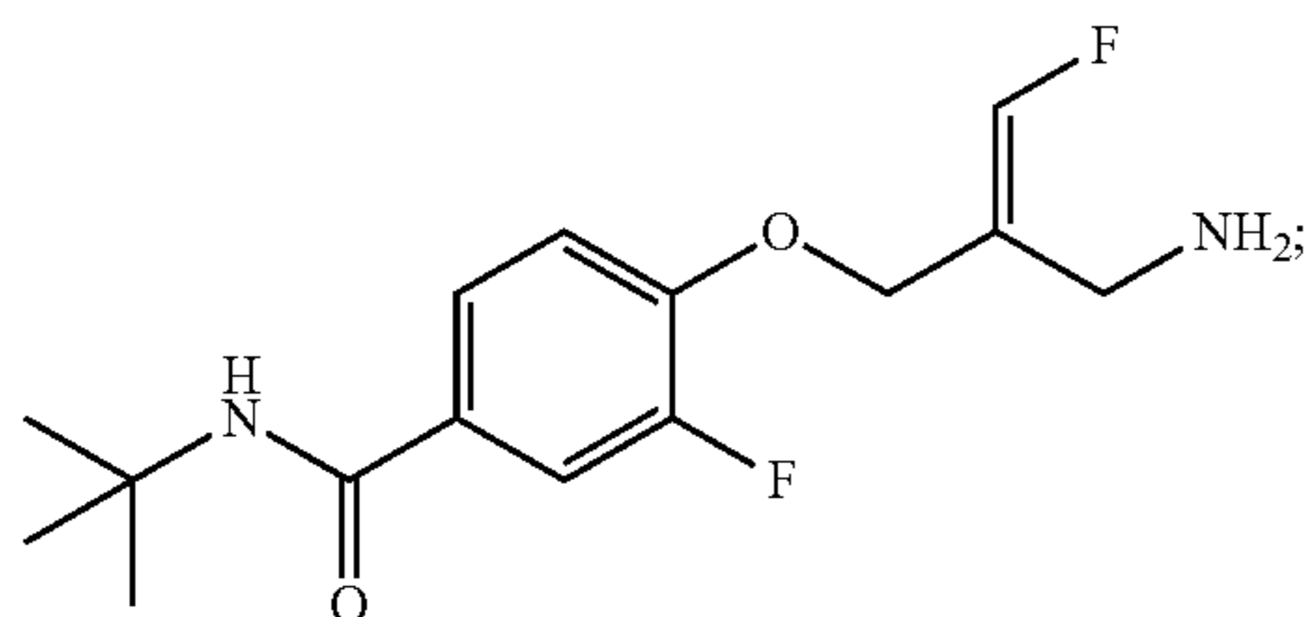
(E)-4-(2-(Aminomethyl)-3-fluoroallyloxy)-N-tert-butyl-3-fluorobenzamide
