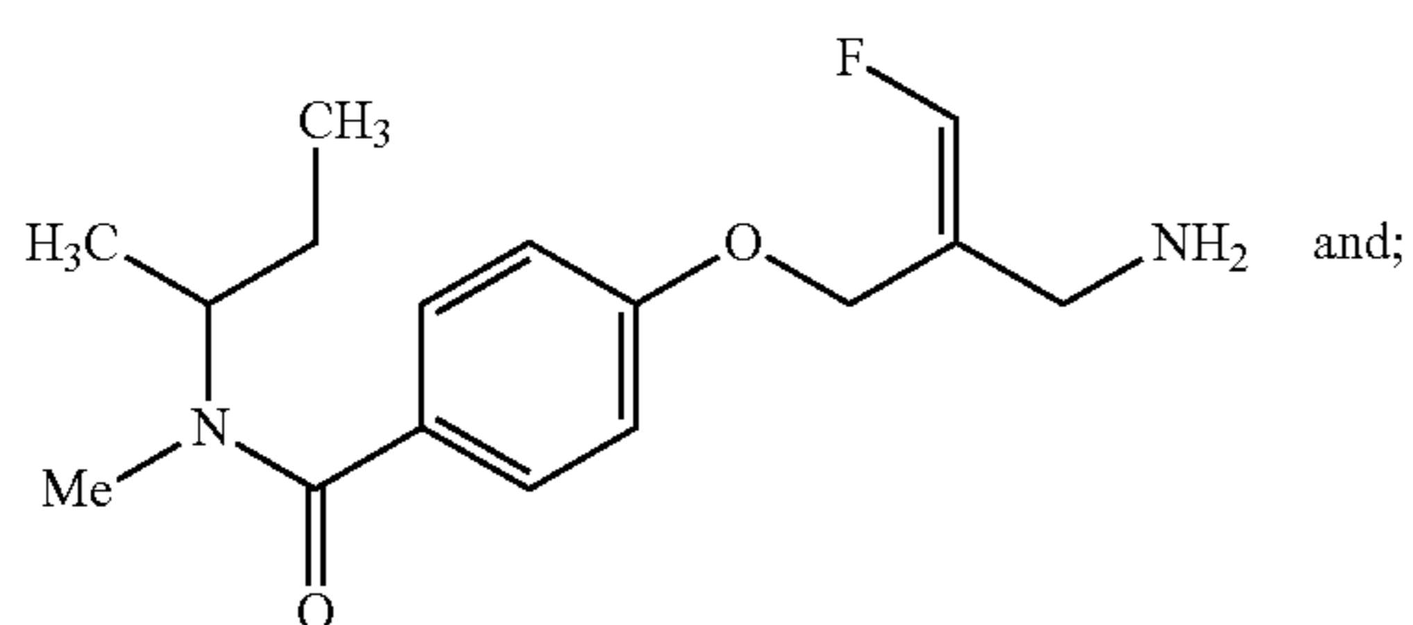
(Z)-4-(2-(Aminomethyl)-3-fluoroallyloxy)-N-sec-butyl-N-methylbenzamide
