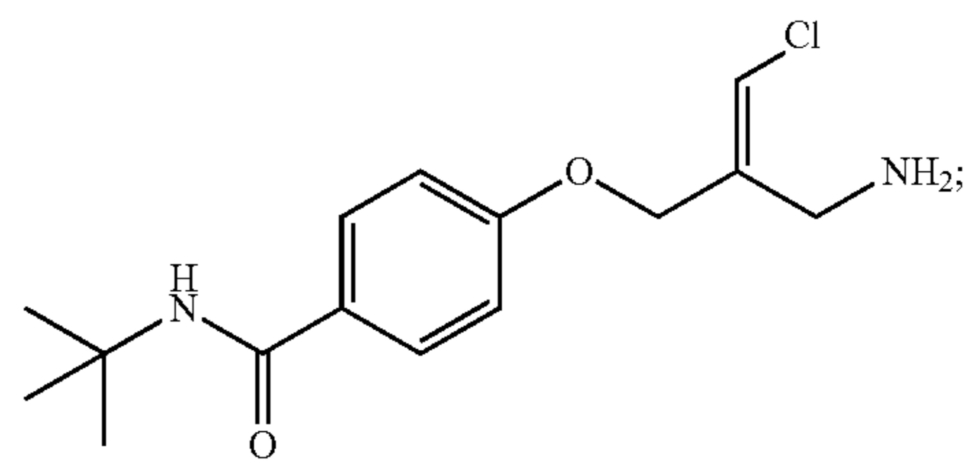
(E)-4-(2-(Aminomethyl)-3-chloroallyloxy)-N-tert-butylbenzamide
