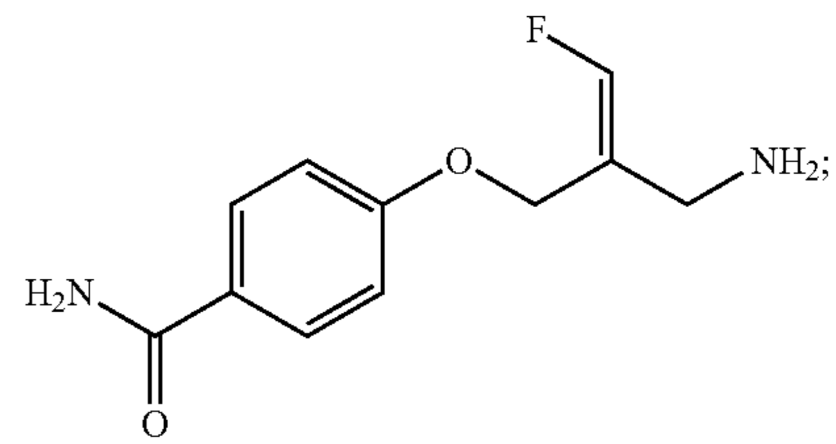
(Z)-4-(2-(Aminomethyl)-3-fluoroallyloxy)benzamide
