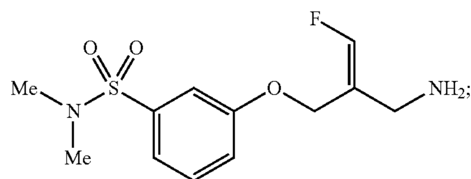
(Z)-3-(2-(Aminomethyl)-3-fluoroallyloxy)-N,N-dimethylbenzenesulfonamide
