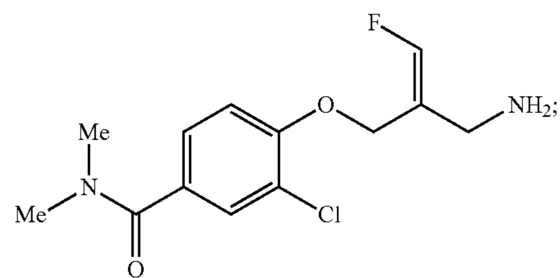
(Z)-4-(2-(Aminomethyl)-3-fluoroallyloxy)-3-chloro-N,N-dimethylbenzamide
