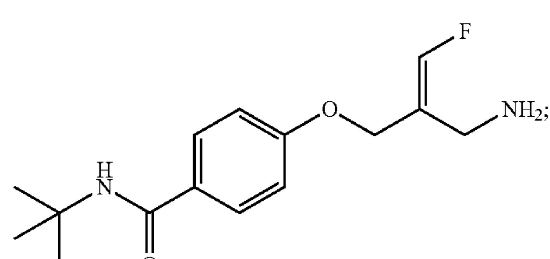
(E)-4-(2-(Aminomethyl)-3-fluoroallyloxy)-N-tert-butylbenzamide
