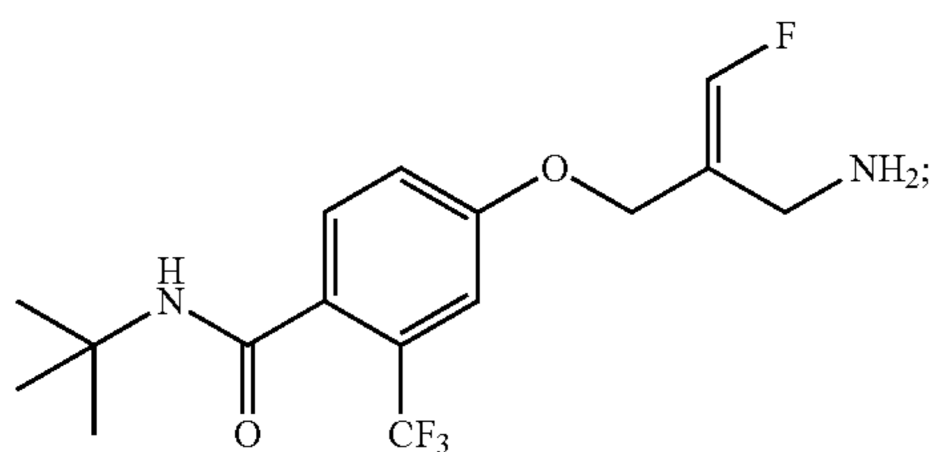
(E)-4-(2-(Aminomethyl)-3-fluoroallyloxy)-N-tert-butyl-2-(trifluoromethyl)benzamide
