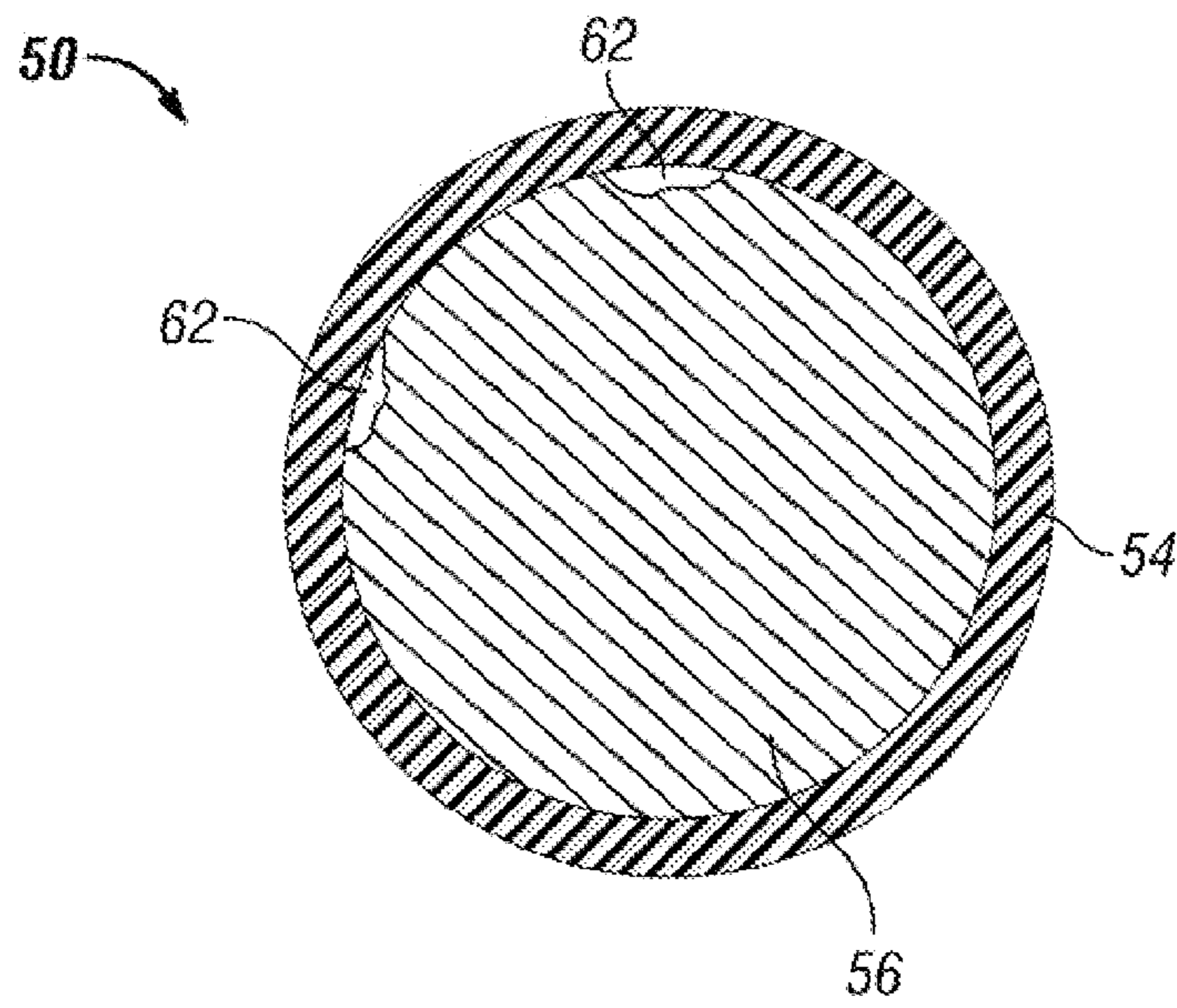
FIG. 1B
