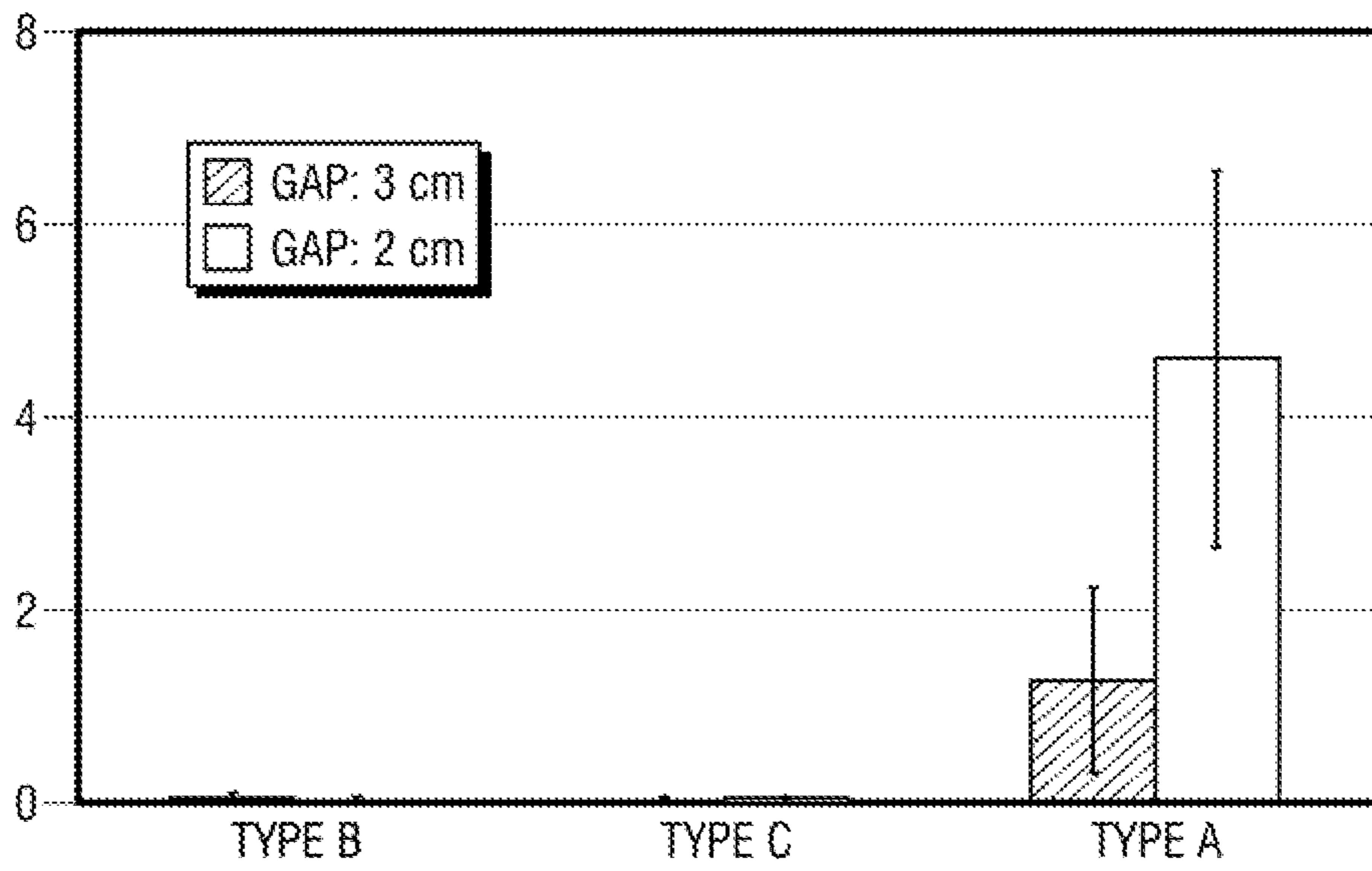
FIG. 12
