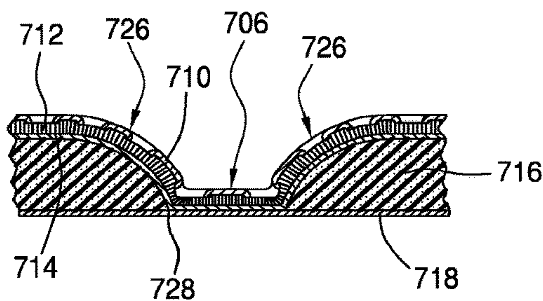
FIG. 32L
