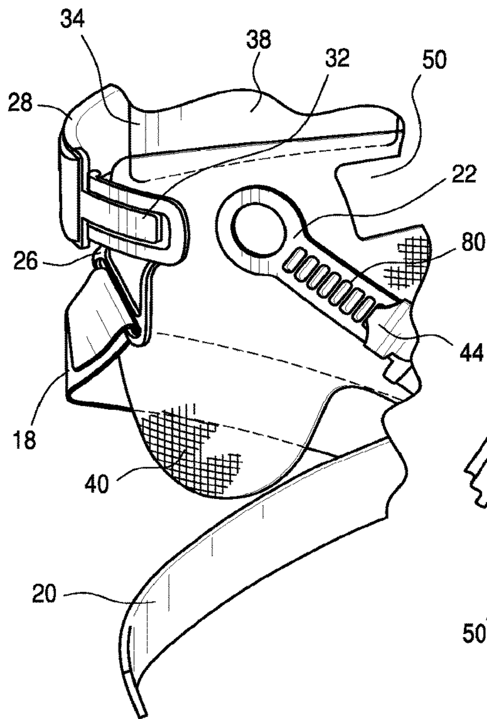
FIG. 20
