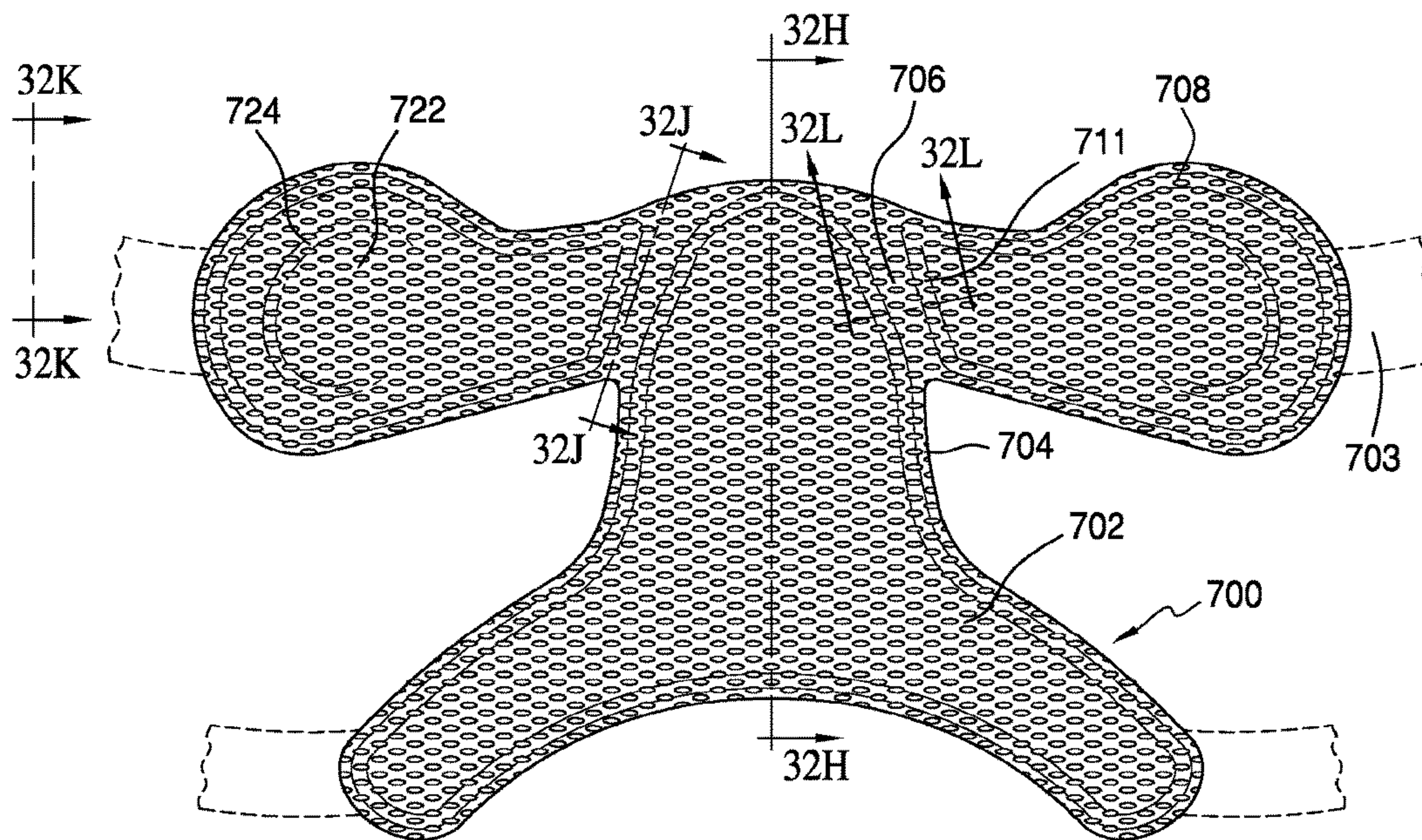
FIG. 32G
