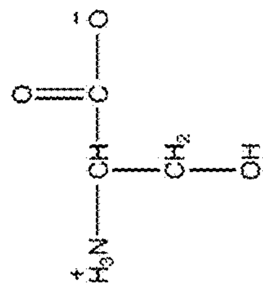
Serine (ser)
