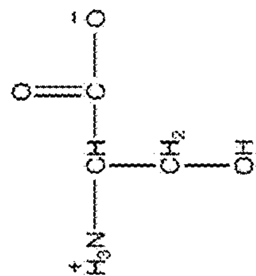
Serine (ser)
