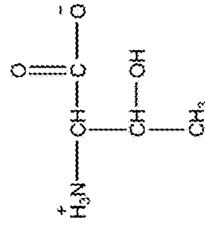
Threonine (thr)
