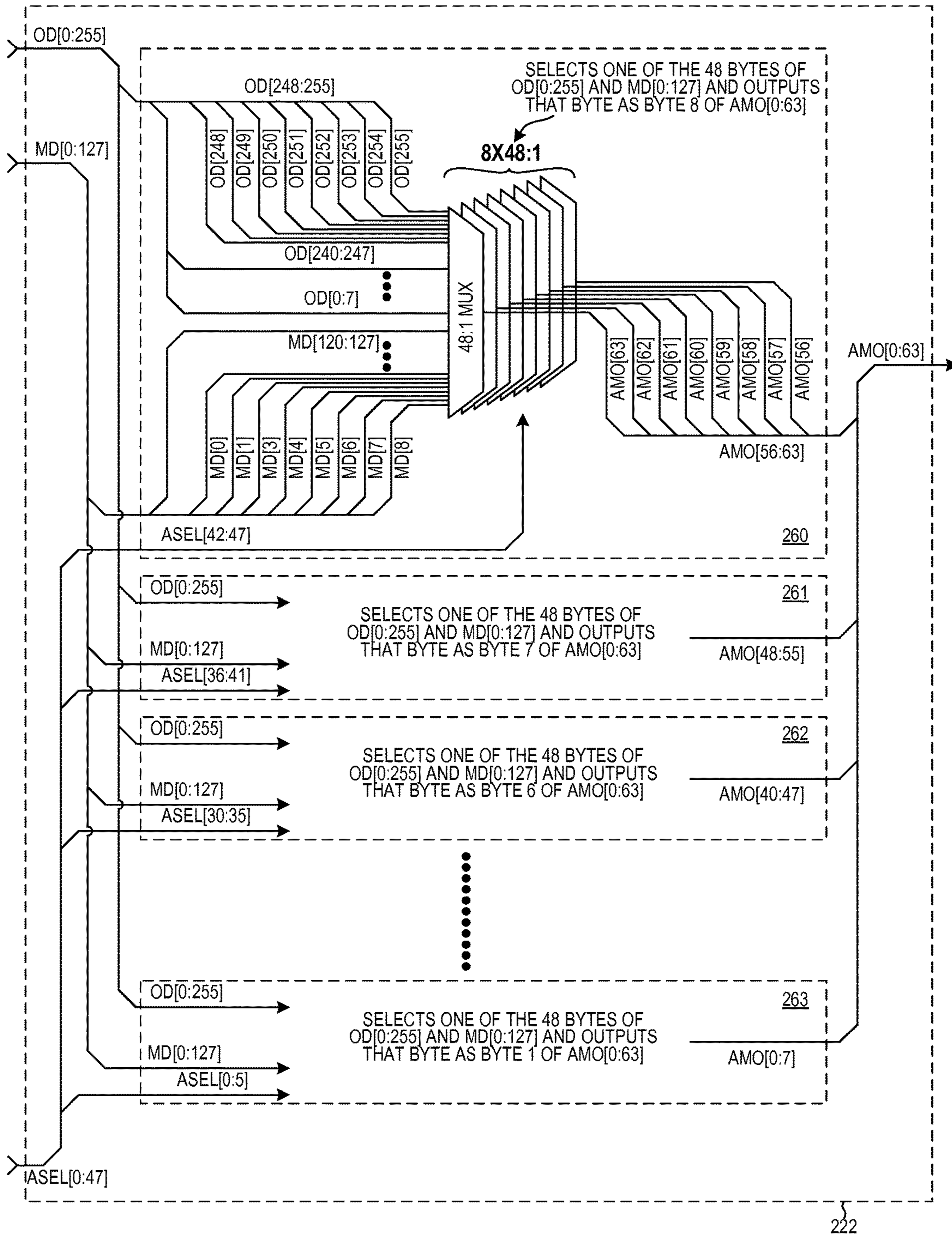
MUX A FIG. 11
