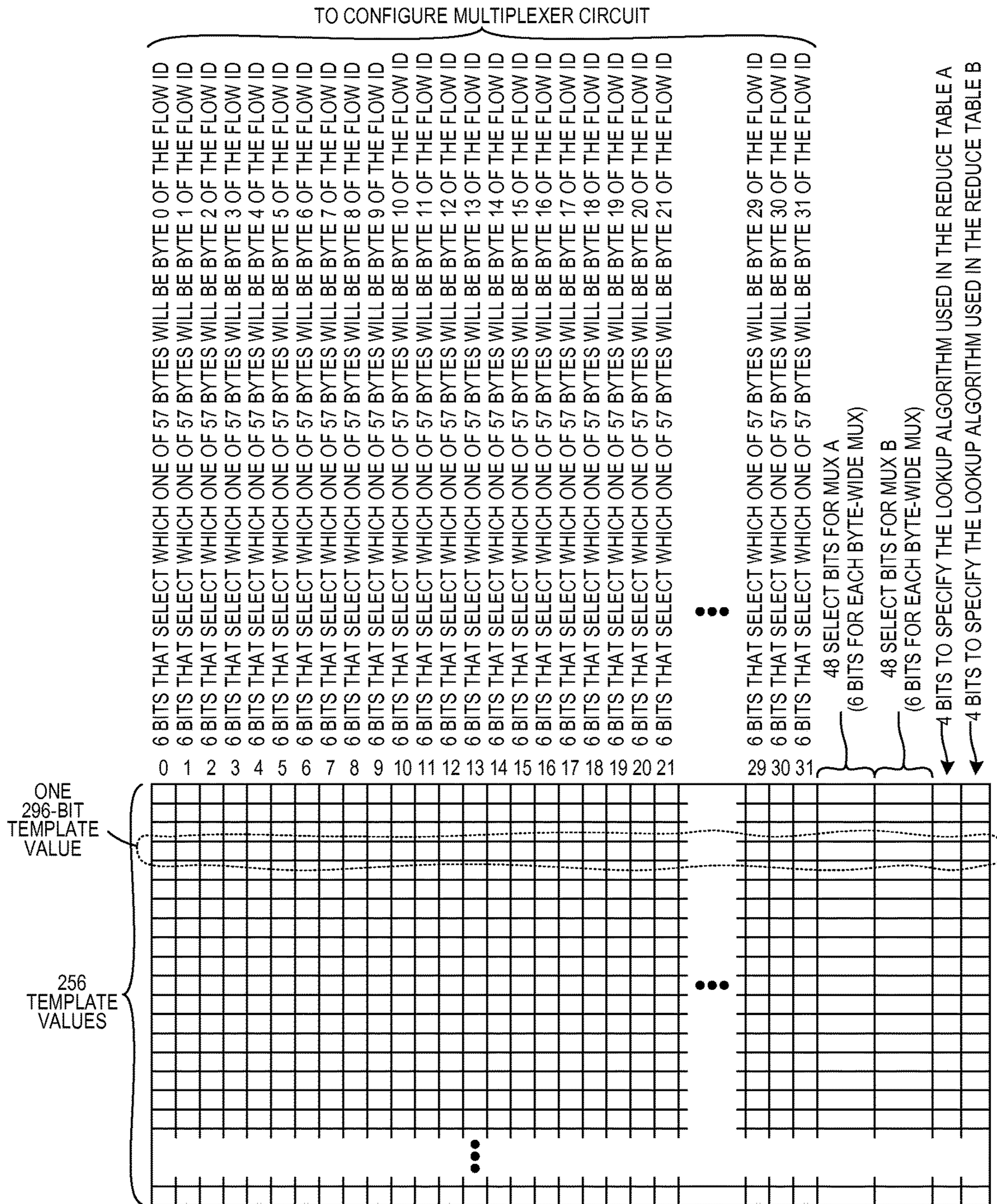
TEMPLATE RAM FIG. 10
