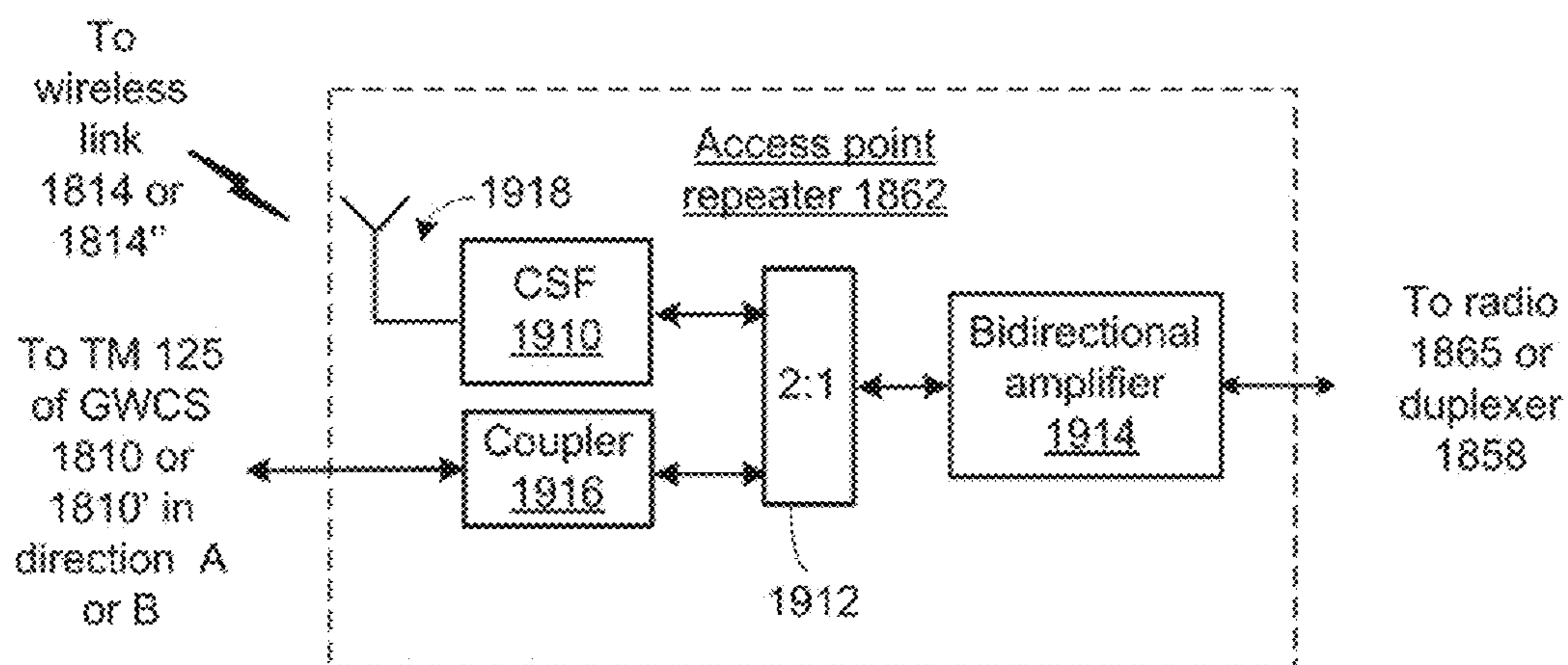
1900 FIG. 19A
