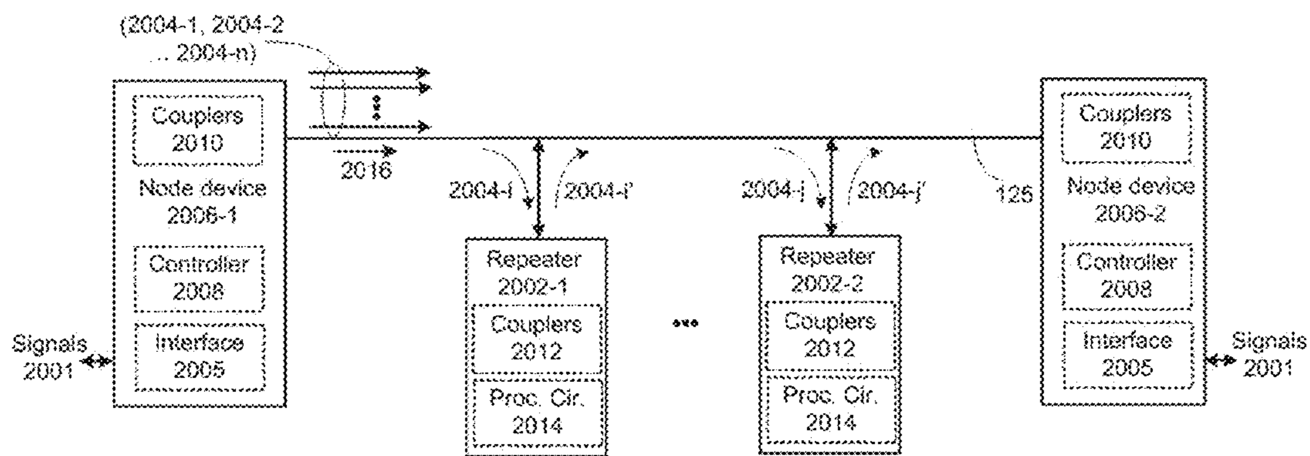
2000 FIG. 20A
