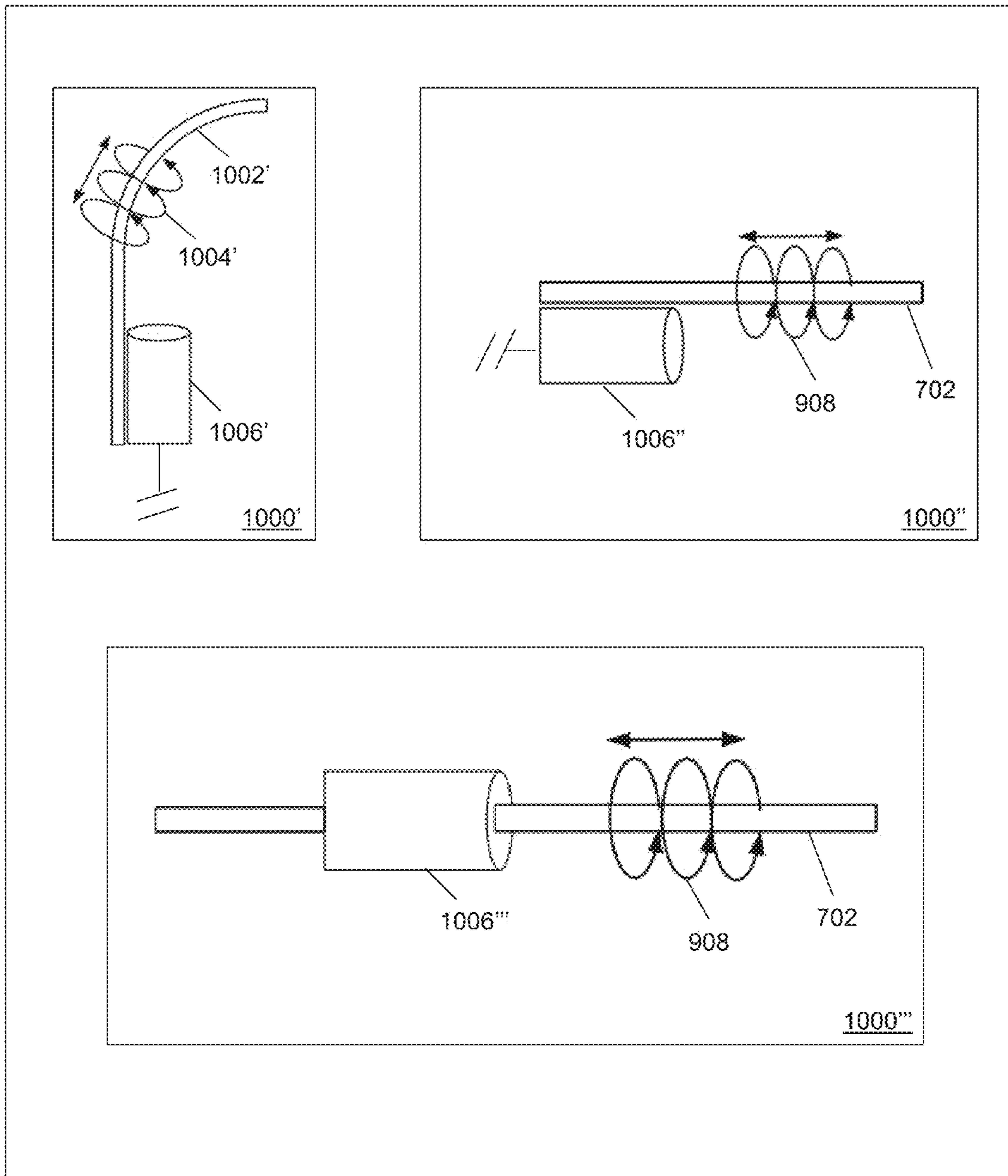
FIG. 10B
