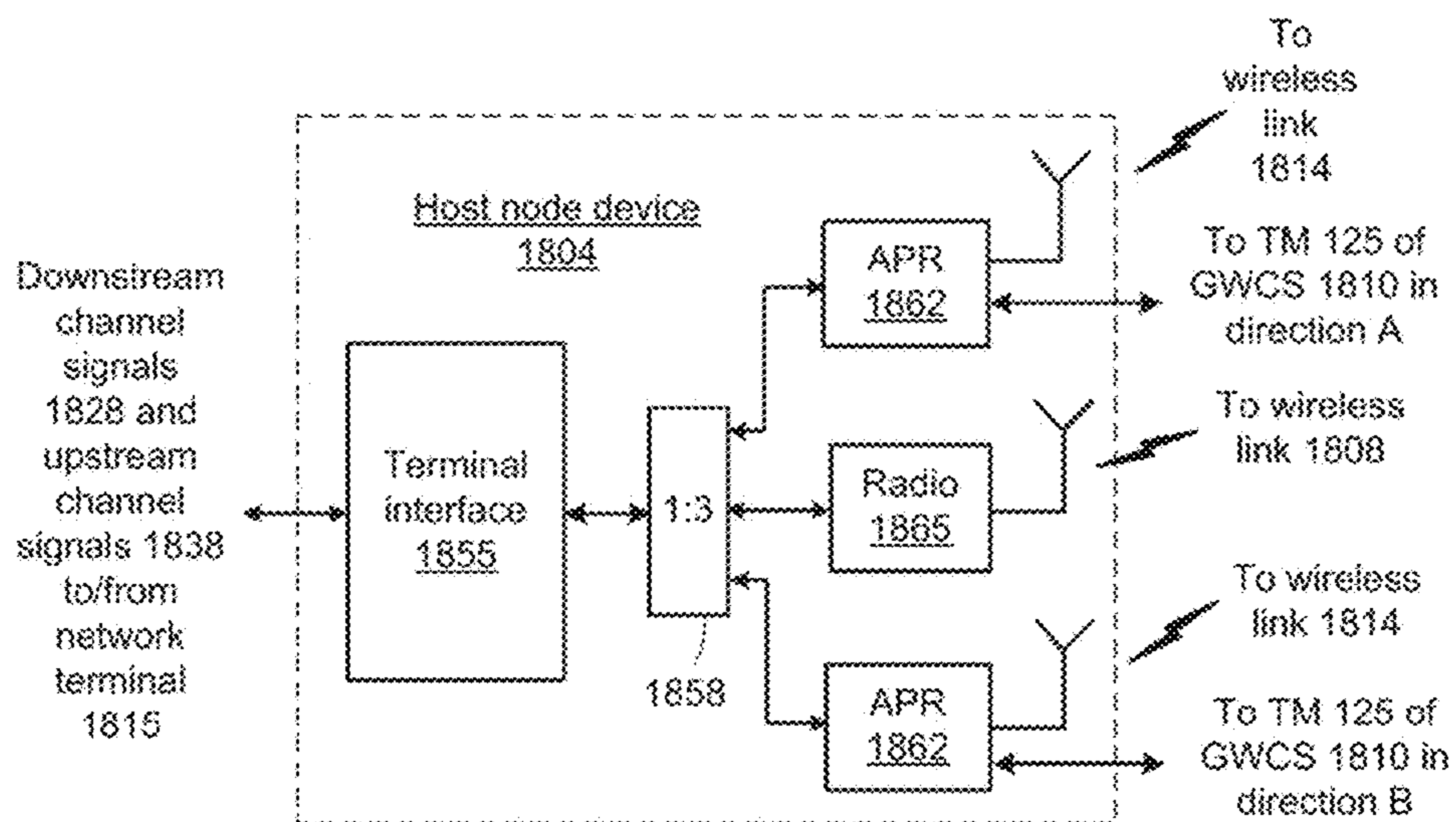
FIG. 18E
