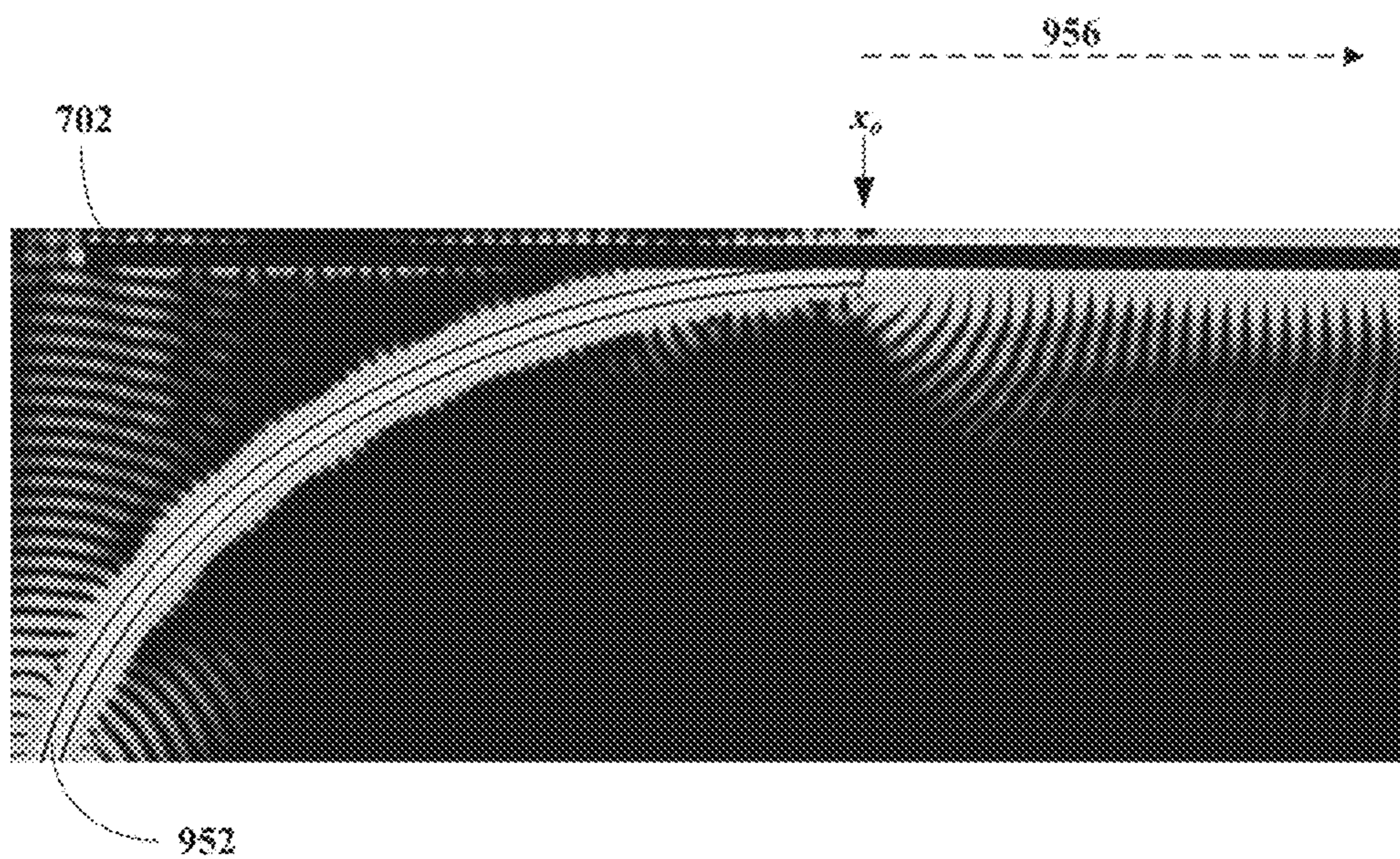
950 FIG. 9B
