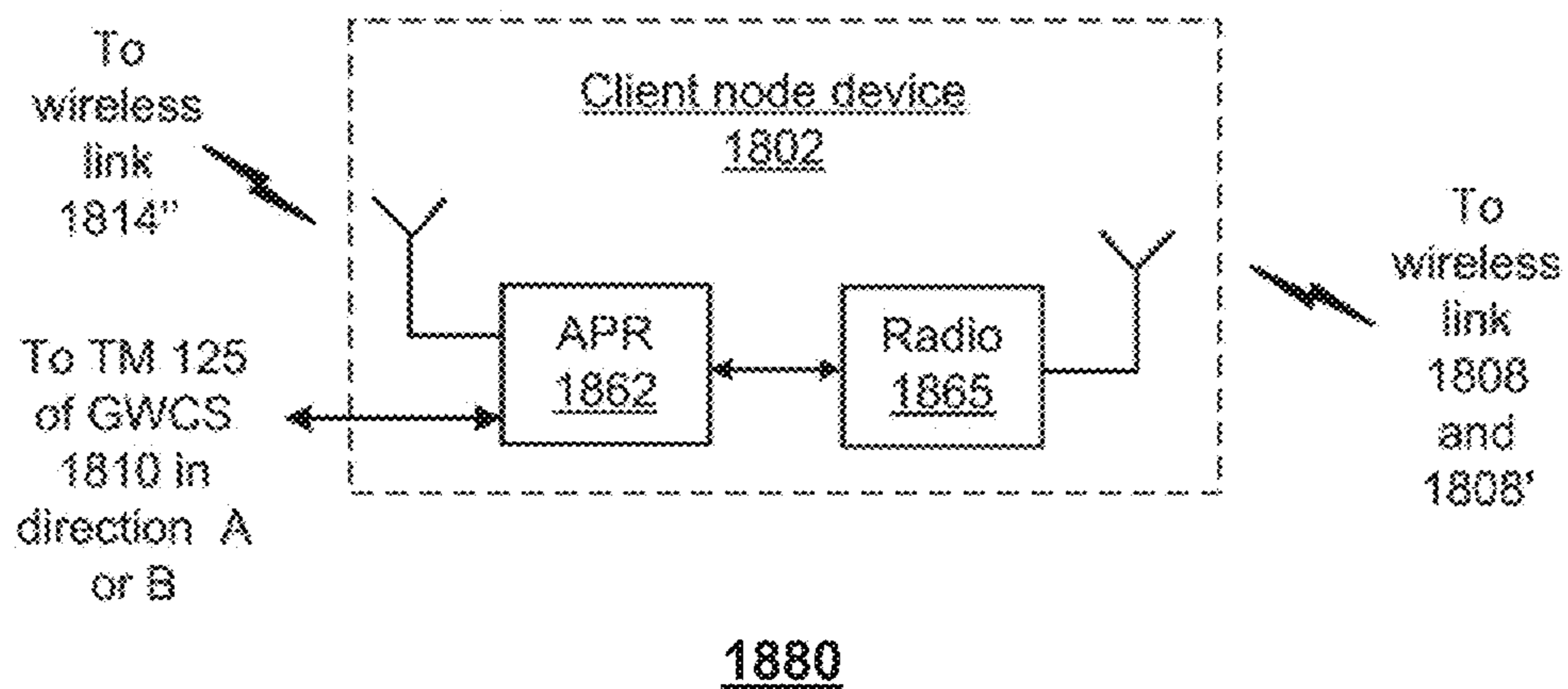
1880 FIG. 18H
