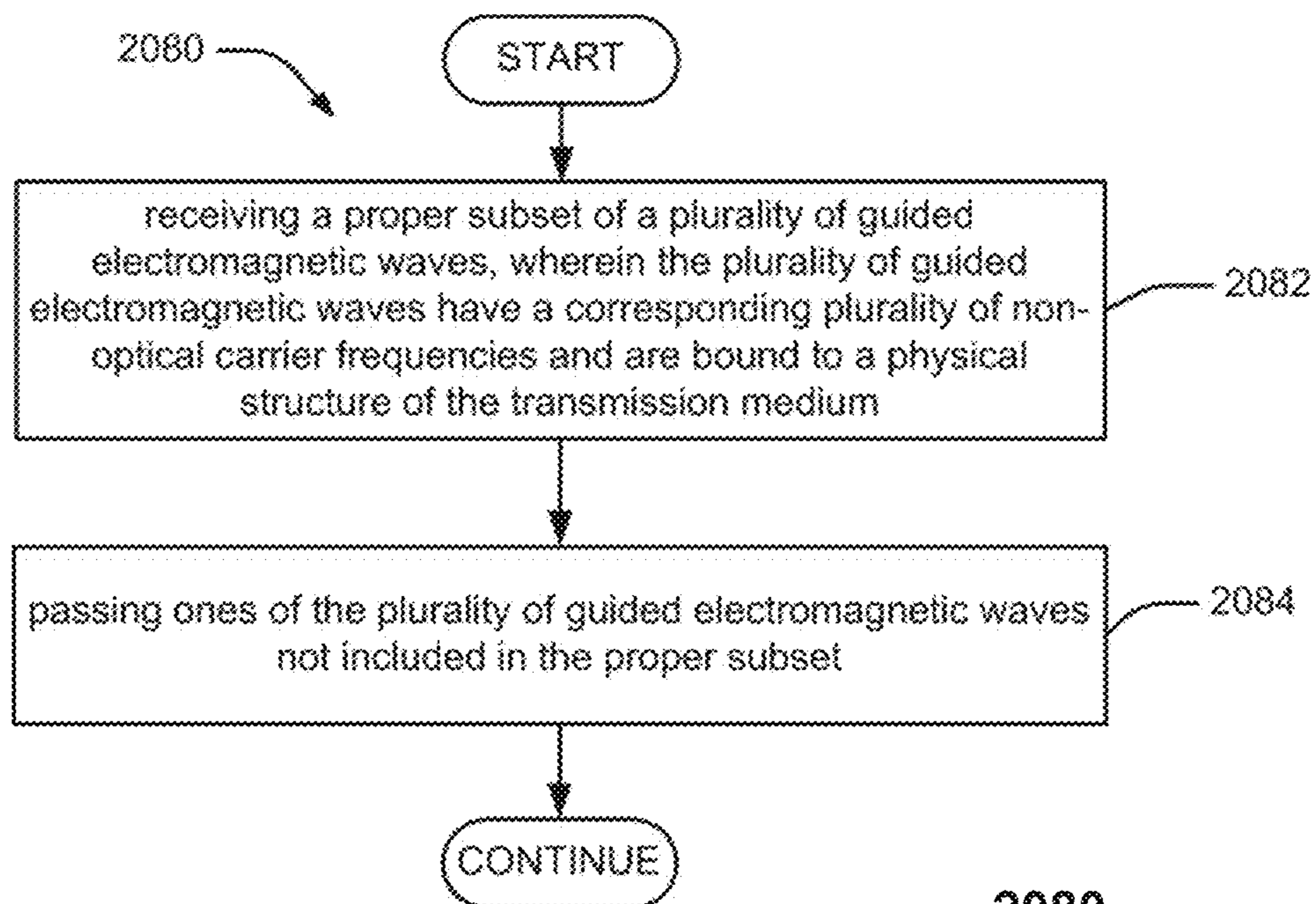
2080 FIG. 20H
