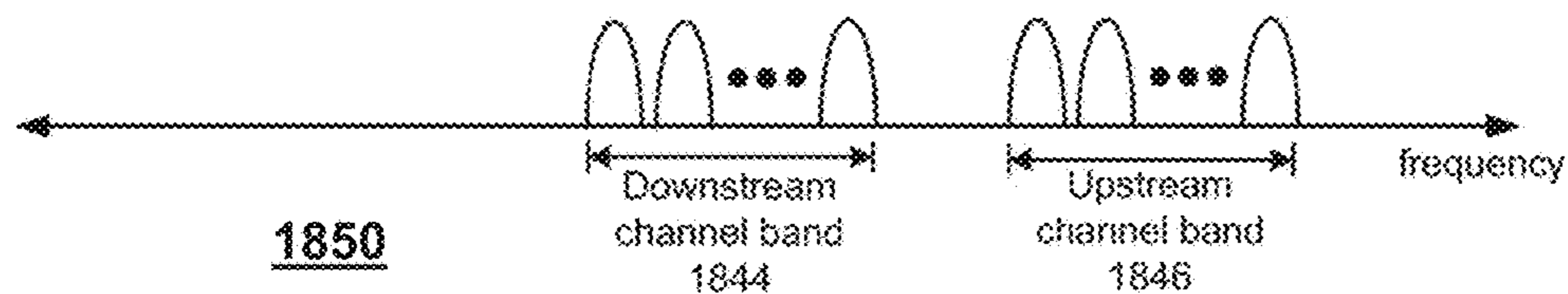
FIG. 18C
