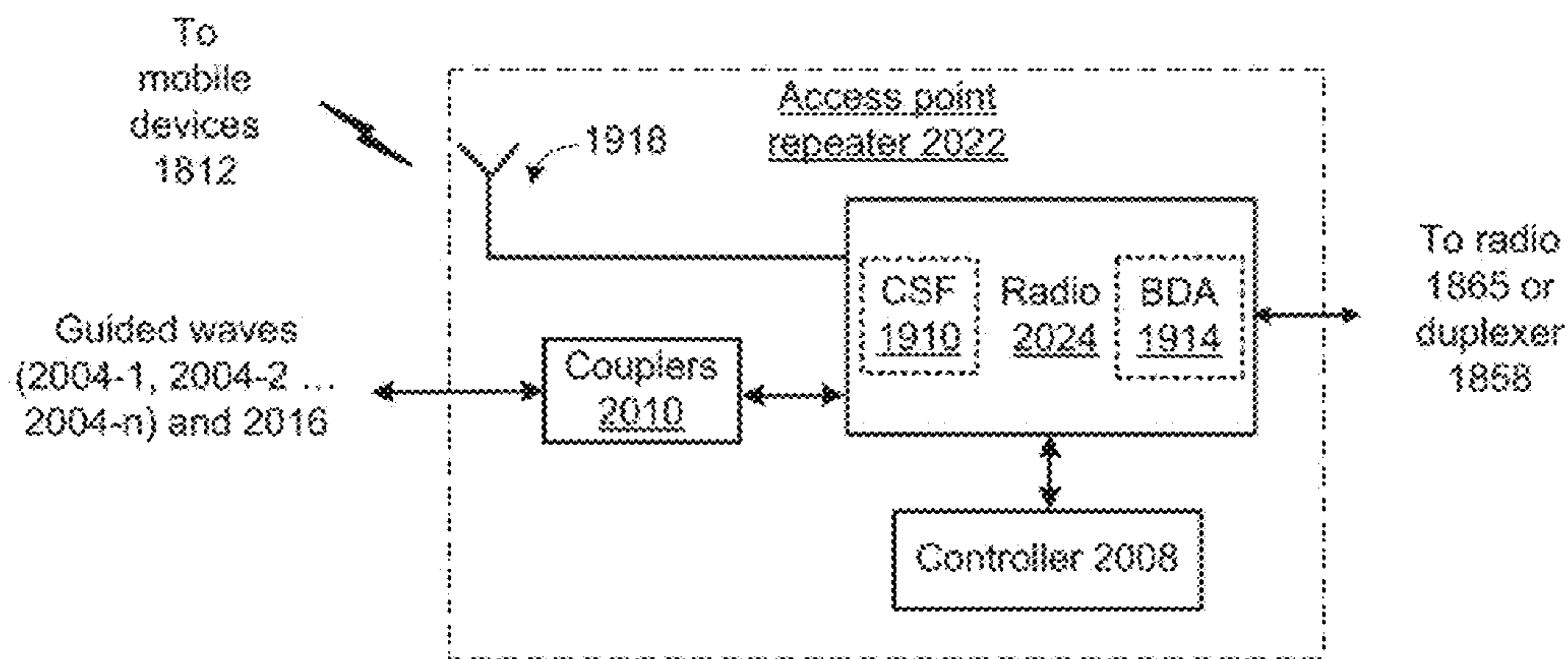
2020 FIG. 20C
