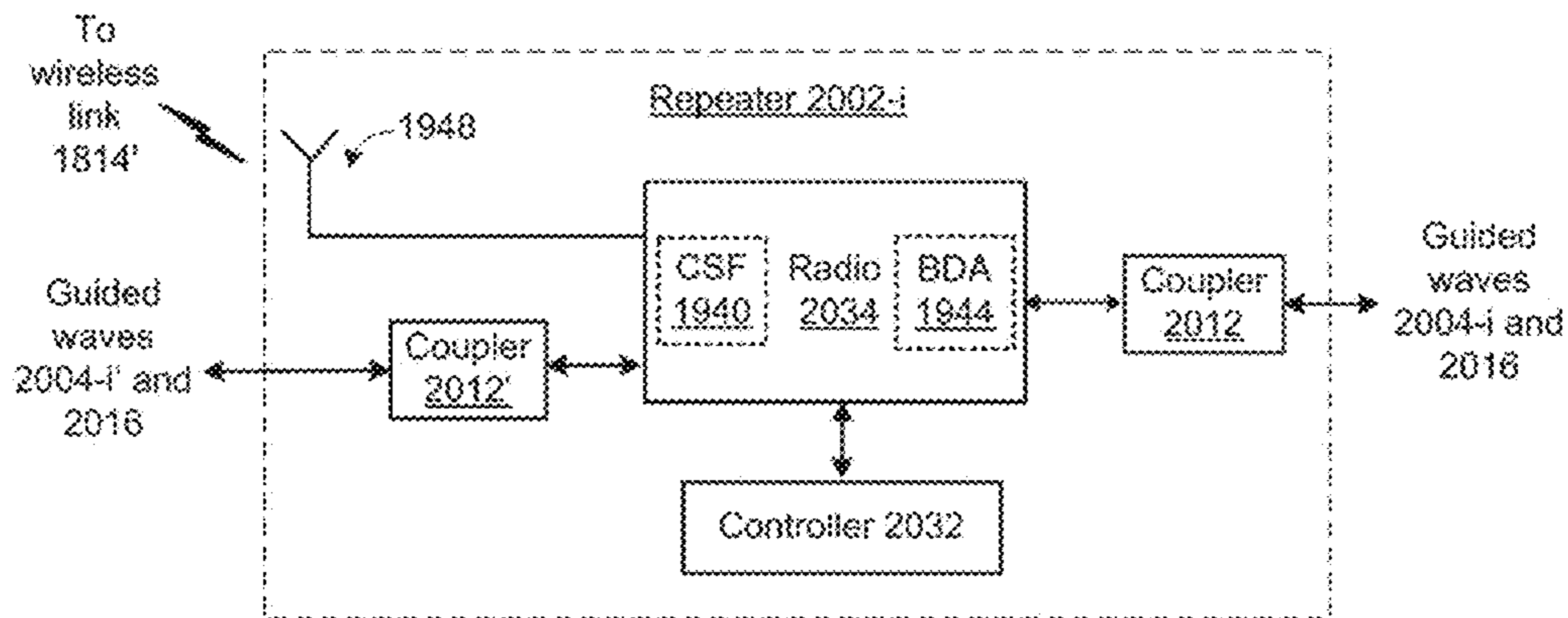
2030 FIG. 20D
