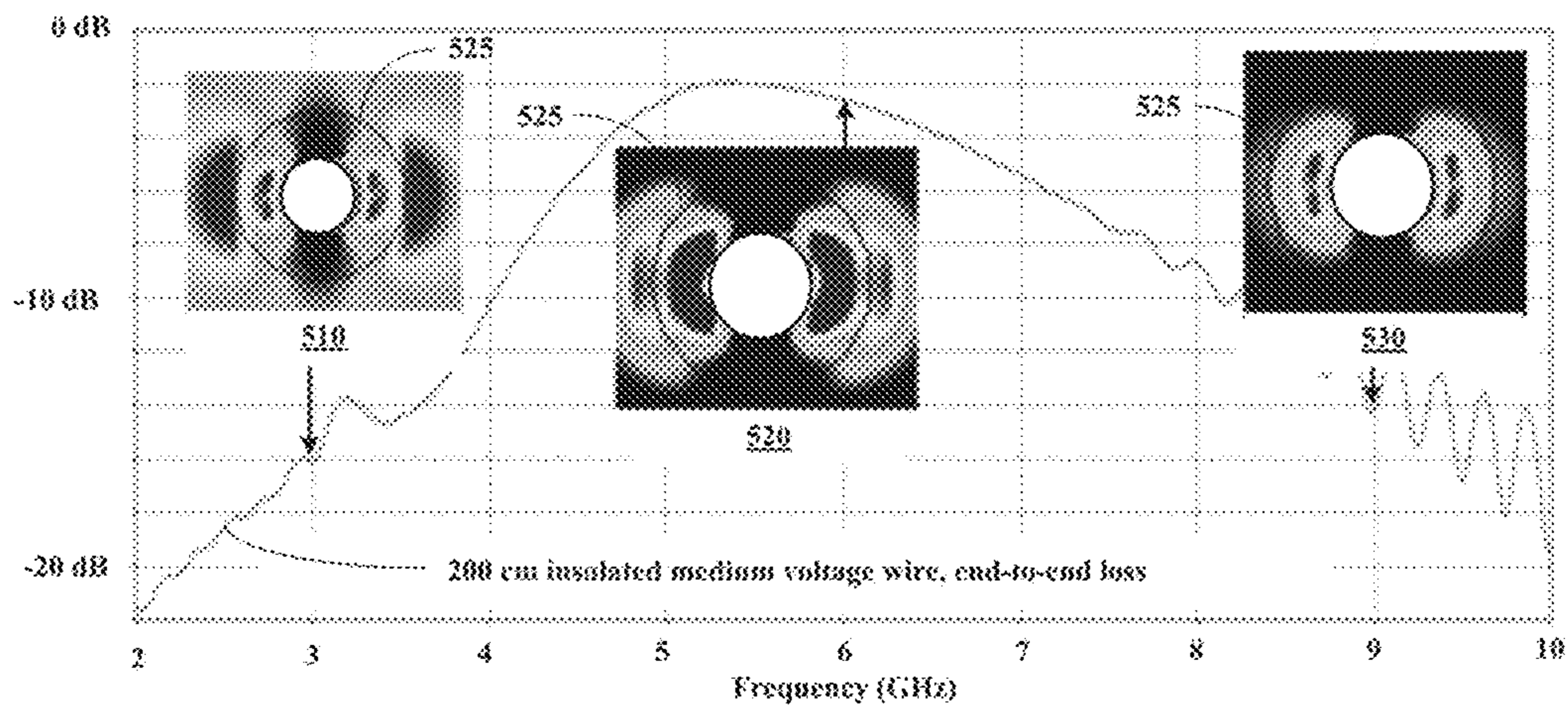
500 FIG. 5A
