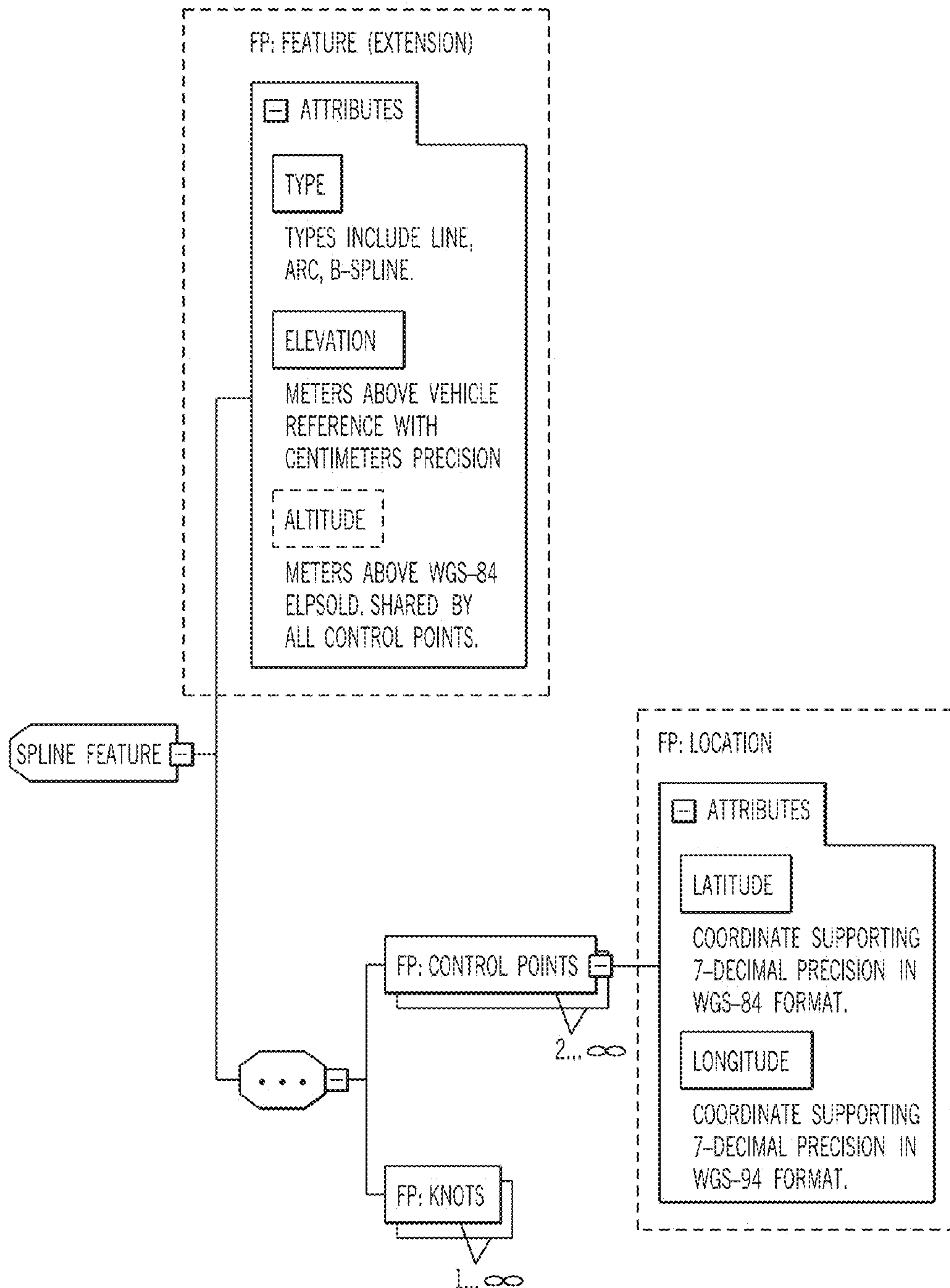
FIG. 5
