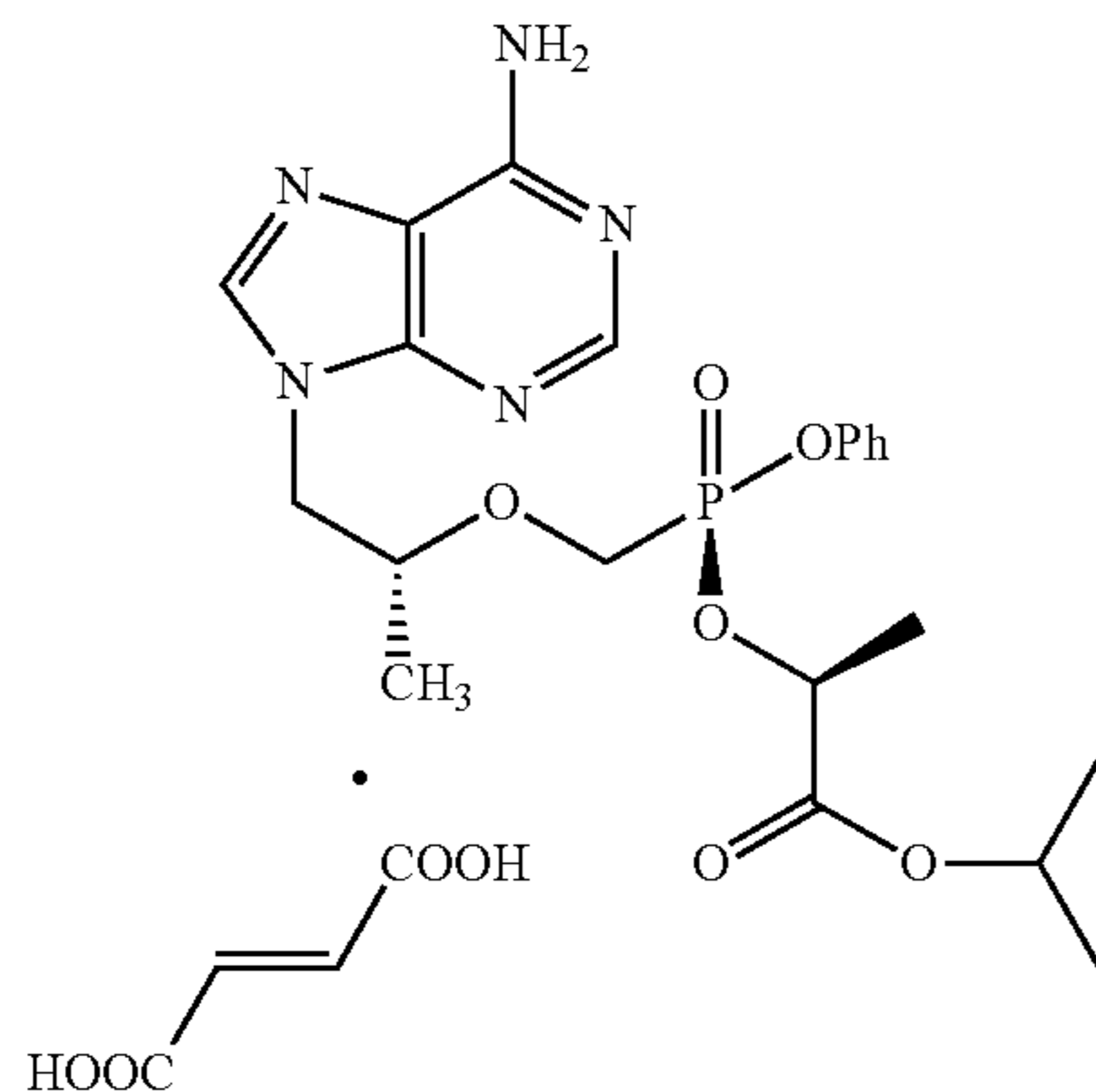
GS-7340
