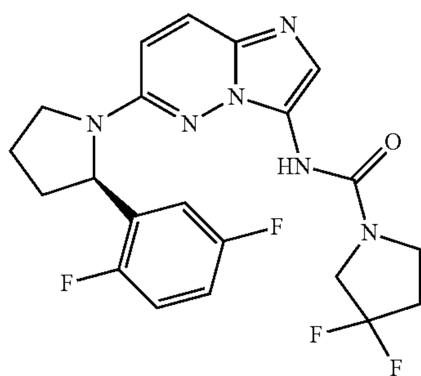
(R)-N-(6-(2-(2,5-difluorophenyl)pyrrolidin-1-yl)imidazo[1,2-b]pyridazin-3-yl)-3,3-difluoropyrrolidine-1-carboxamide
