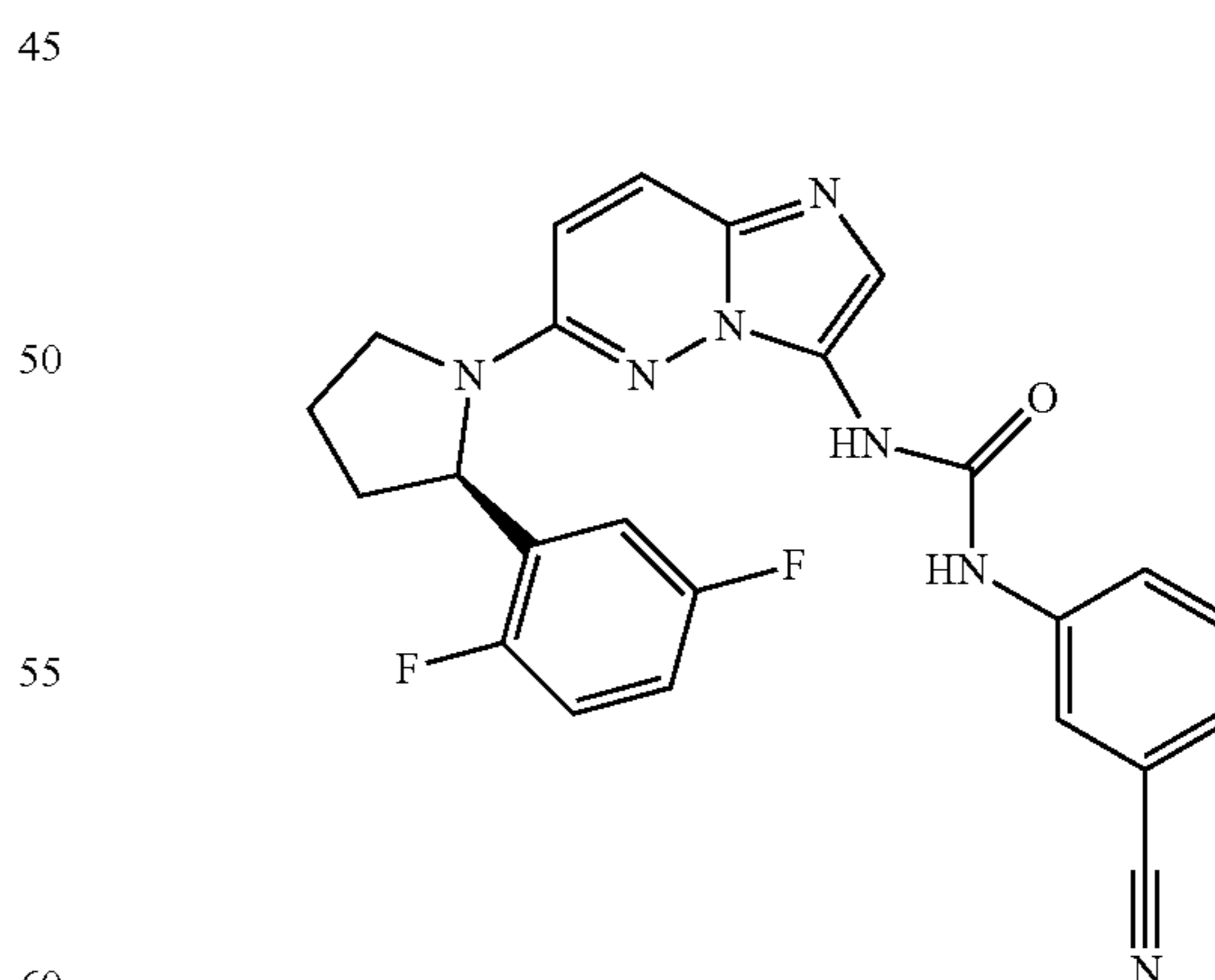
(R)-1-(3-cyanophenyl)-3-(6-(2-(2,5-difluorophenyl)pyrrolidin-1-yl)imidazo[1,2-b]pyridazin-3-yl)urea
