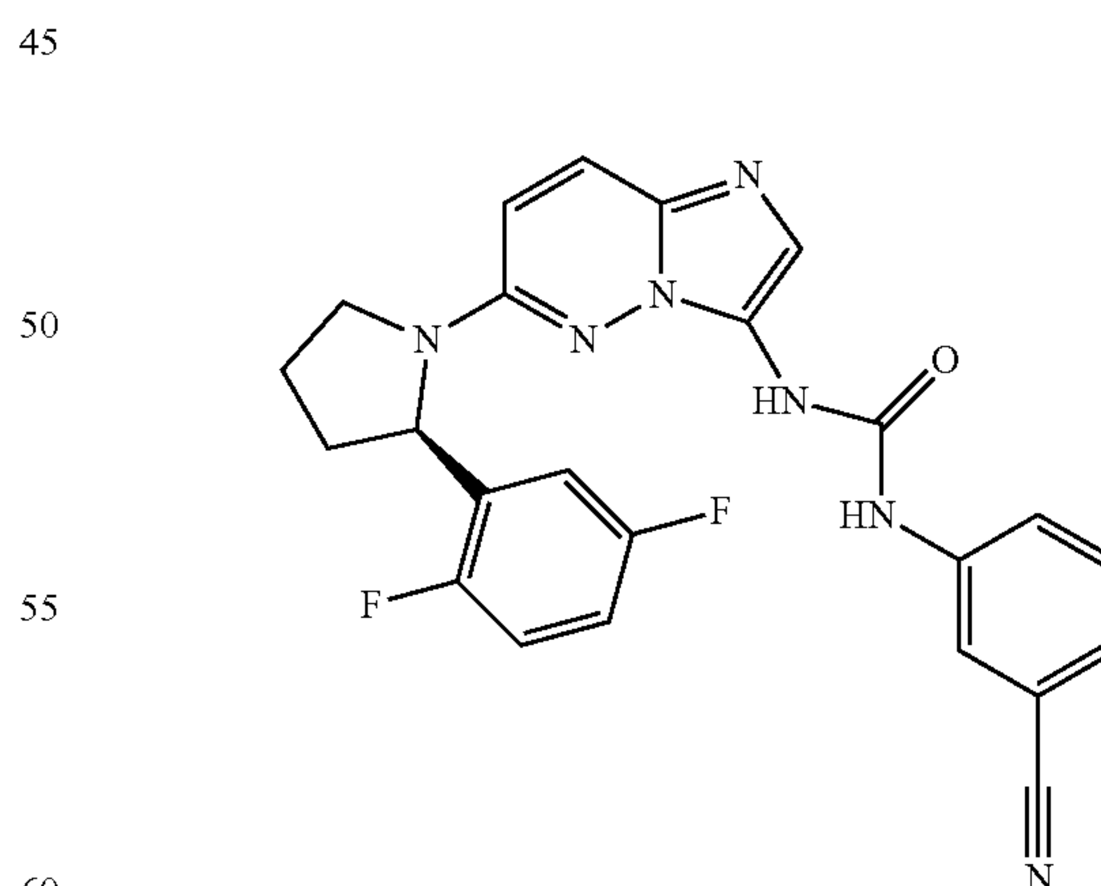
(R)-1-(3-cyanophenyl)-3-(6-(2-(2,5-difluorophenyl)pyrrolidin-1-yl)imidazo[1,2-b]pyridazin-3-yl)urea
