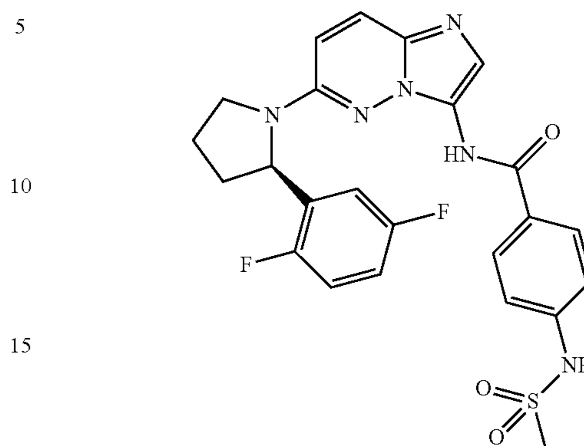
(R)—N-(6-(2-(2,5-difluorophenyl)pyrrolidin-1-yl)imidazo[1,2-b]pyridazin-3-yl)-4-(methylsulfonylamido)benzamide
