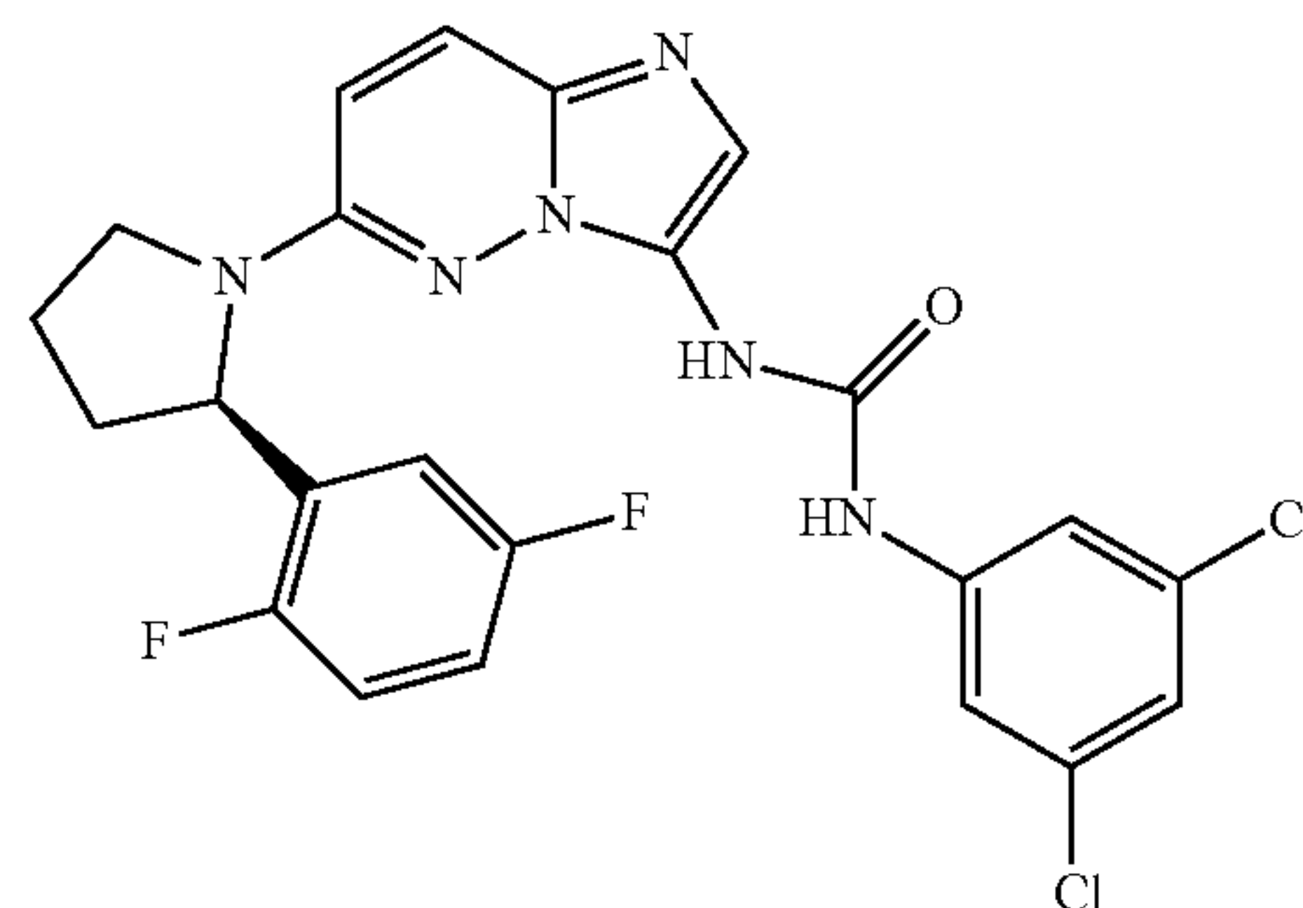
(R)-1-(3,5-dichlorophenyl)-3-(6-(2-(2,5-difluorophenyl)pyrrolidin-1-yl)imidazo[1,2-b]pyridazin-3-yl)urea
