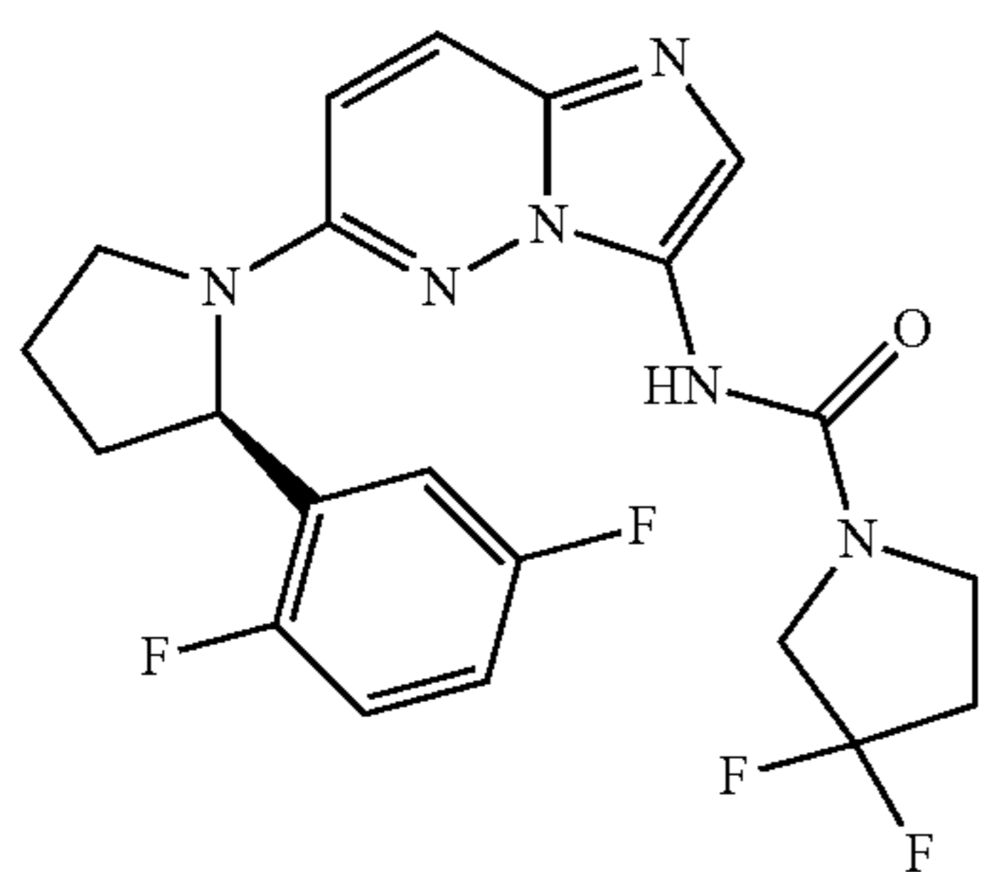
(R)-N-(6-(2-(2,5-difluorophenyl)pyrrolidin-1-yl)imidazo[1,2-b]pyridazin-3-yl)-3,3-difluoropyrrolidine-1-carboxamide
