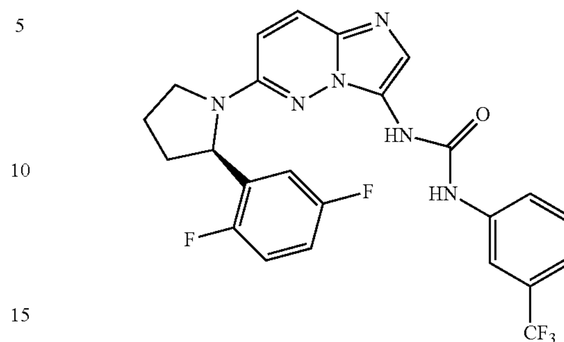
(R)-1-(6-(2-(2,5-difluorophenyl)pyrrolidin-1-yl)imidazo[1,2-b]pyridazin-3-yl)-3-(3-(trifluoromethyl)phenyl)urea
