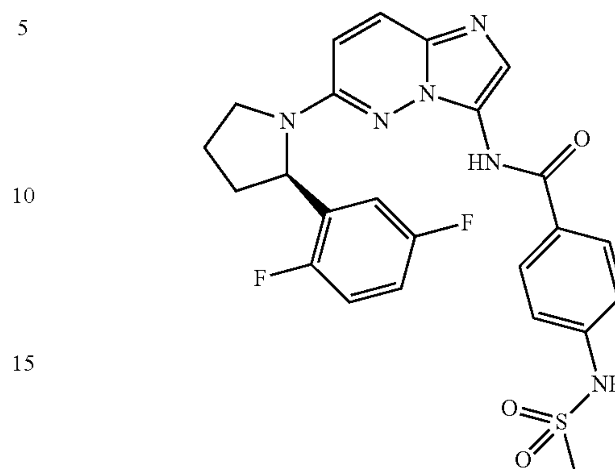
(R)—N-(6-(2-(2,5-difluorophenyl)pyrrolidin-1-yl)imidazo[1,2-b]pyridazin-3-yl)-4-(methylsulfonylamido)benzamide
