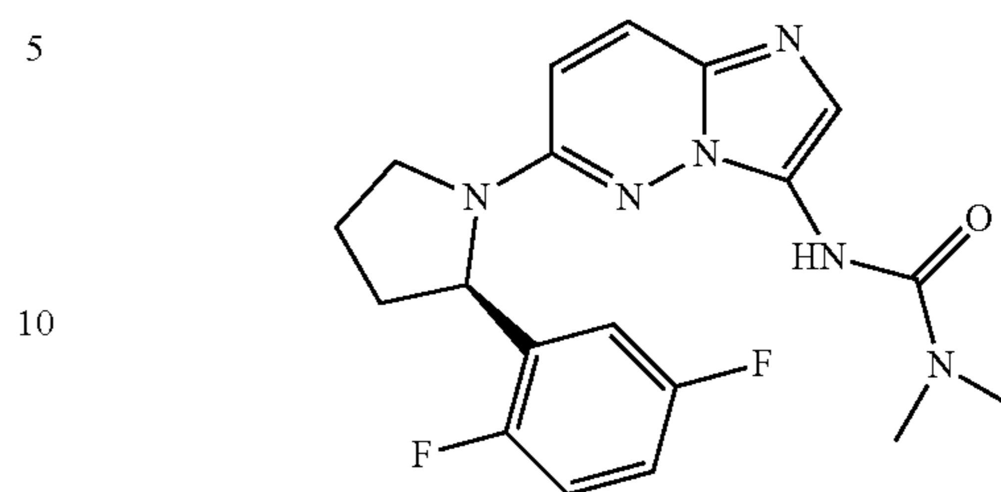
(R)-3-(6-(2-(2,5-difluorophenyl)pyrrolidin-1-yl)imidazo[1,2-b]pyridazin-3-yl)-1,1-dimethylurea
