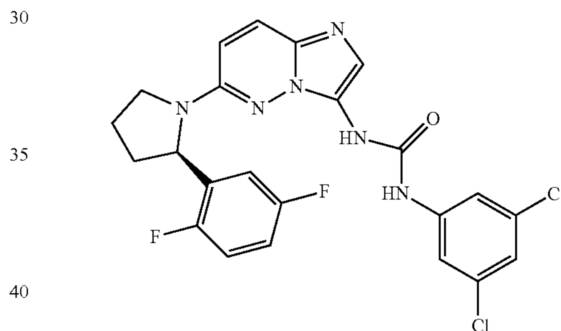
(R)-1-(3,5-dichlorophenyl)-3-(6-(2-(2,5-difluorophenyl)pyrrolidin-1-yl)imidazo[1,2-b]pyridazin-3-yl)urea
