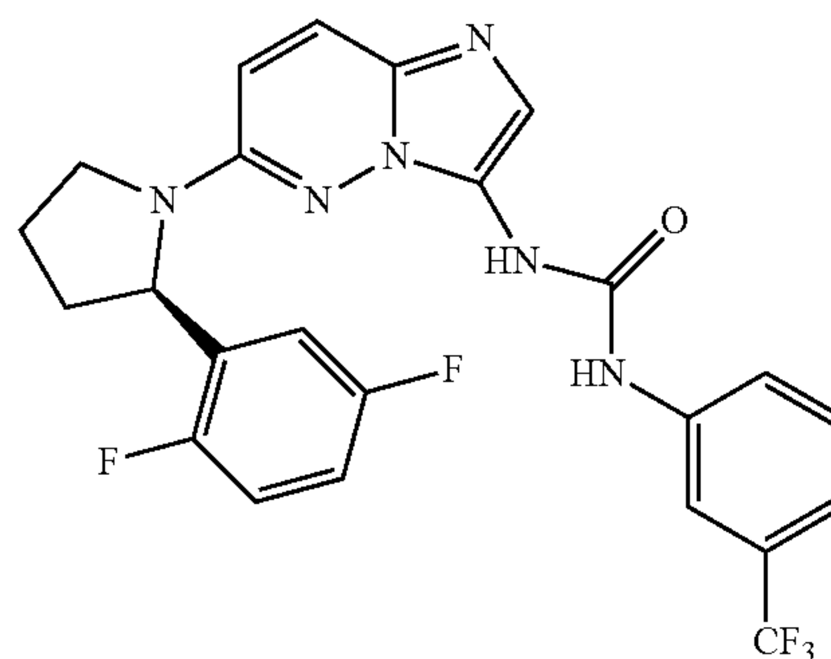
(R)-1-(6-(2-(2,5-difluorophenyl)pyrrolidin-1-yl)imidazo[1,2-b]pyridazin-3-yl)-3-(3-(trifluoromethyl)phenyl)urea
