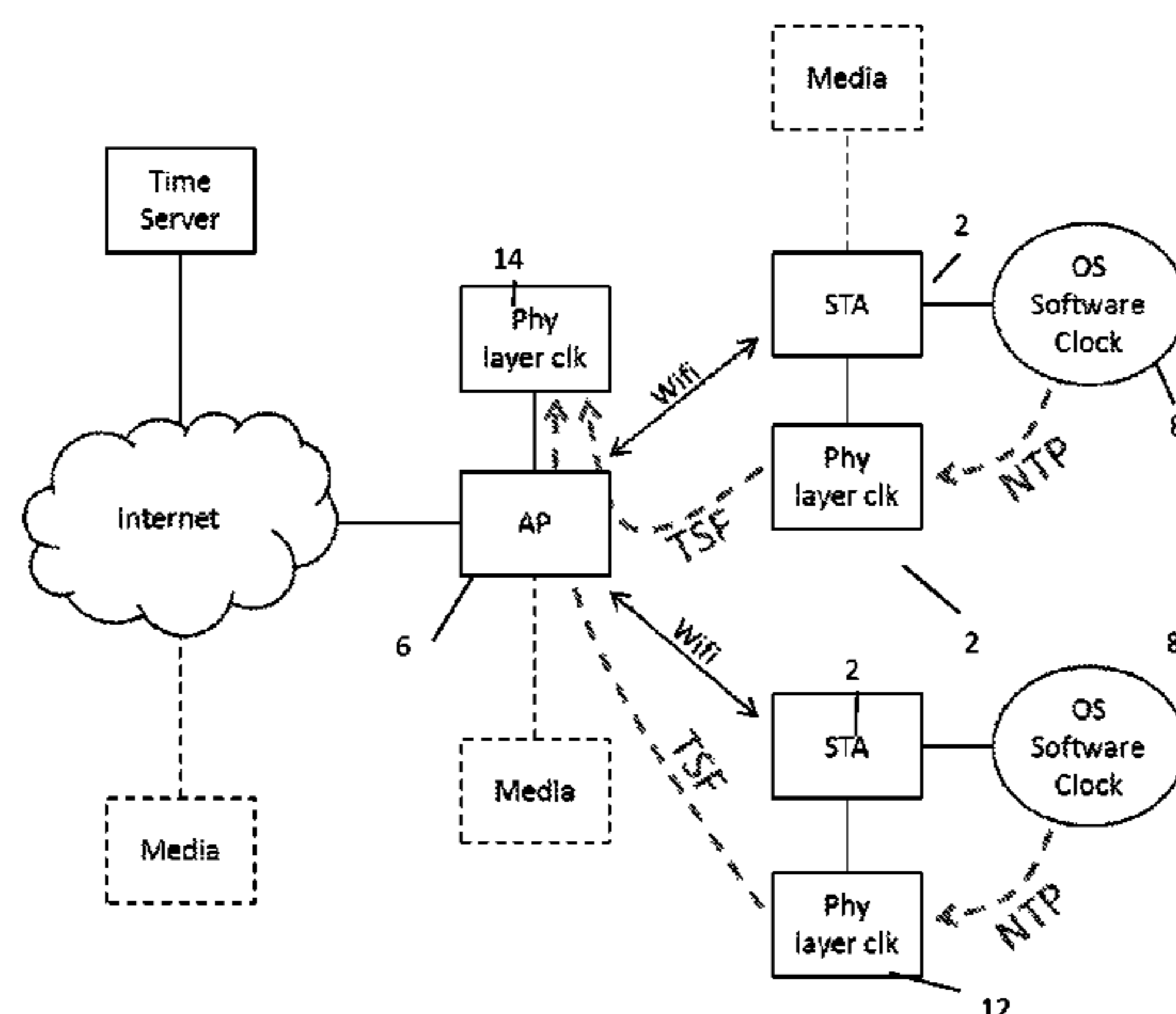
Multiple-protocol layer synchronisation technique
