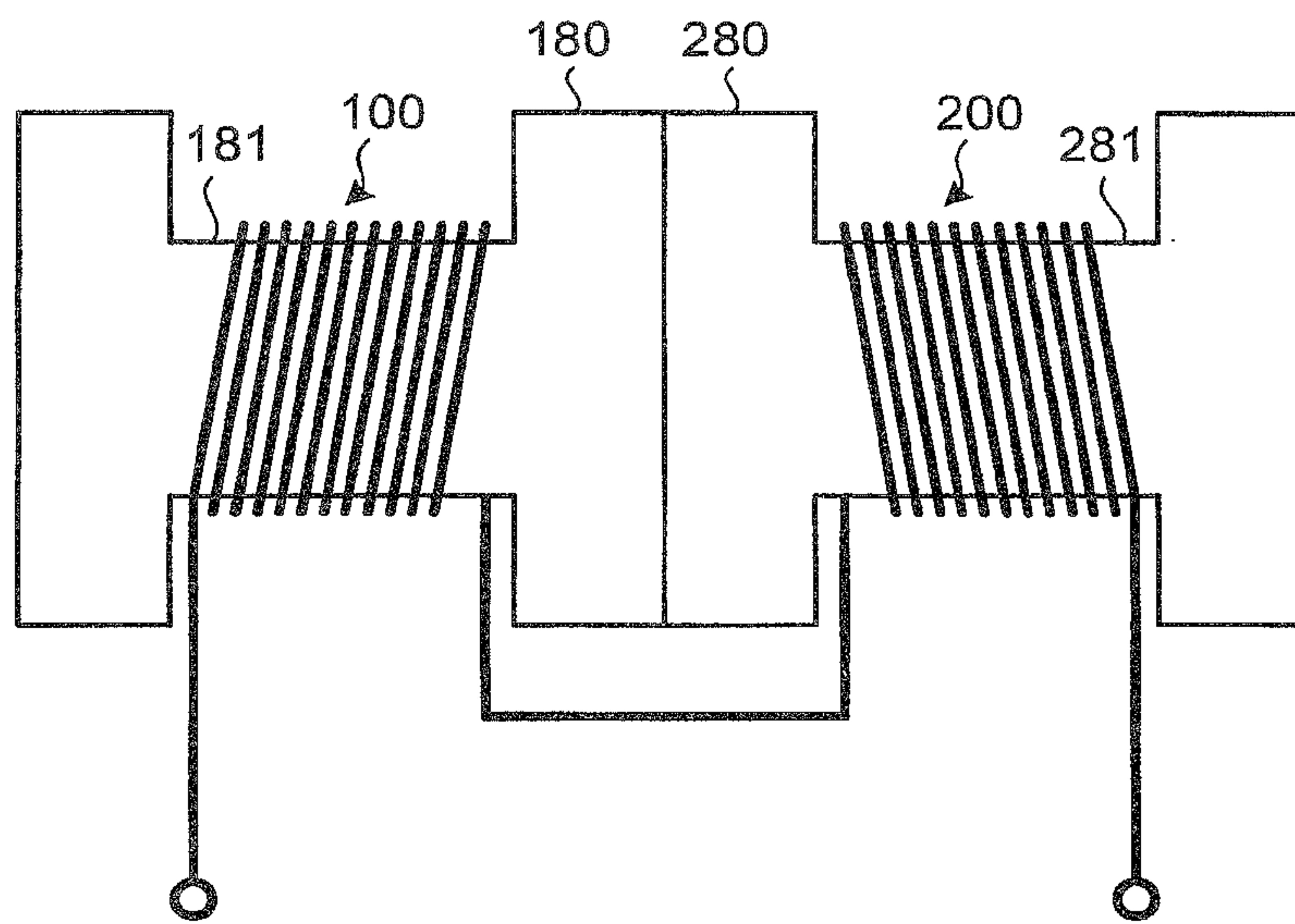
FIG. 1A
