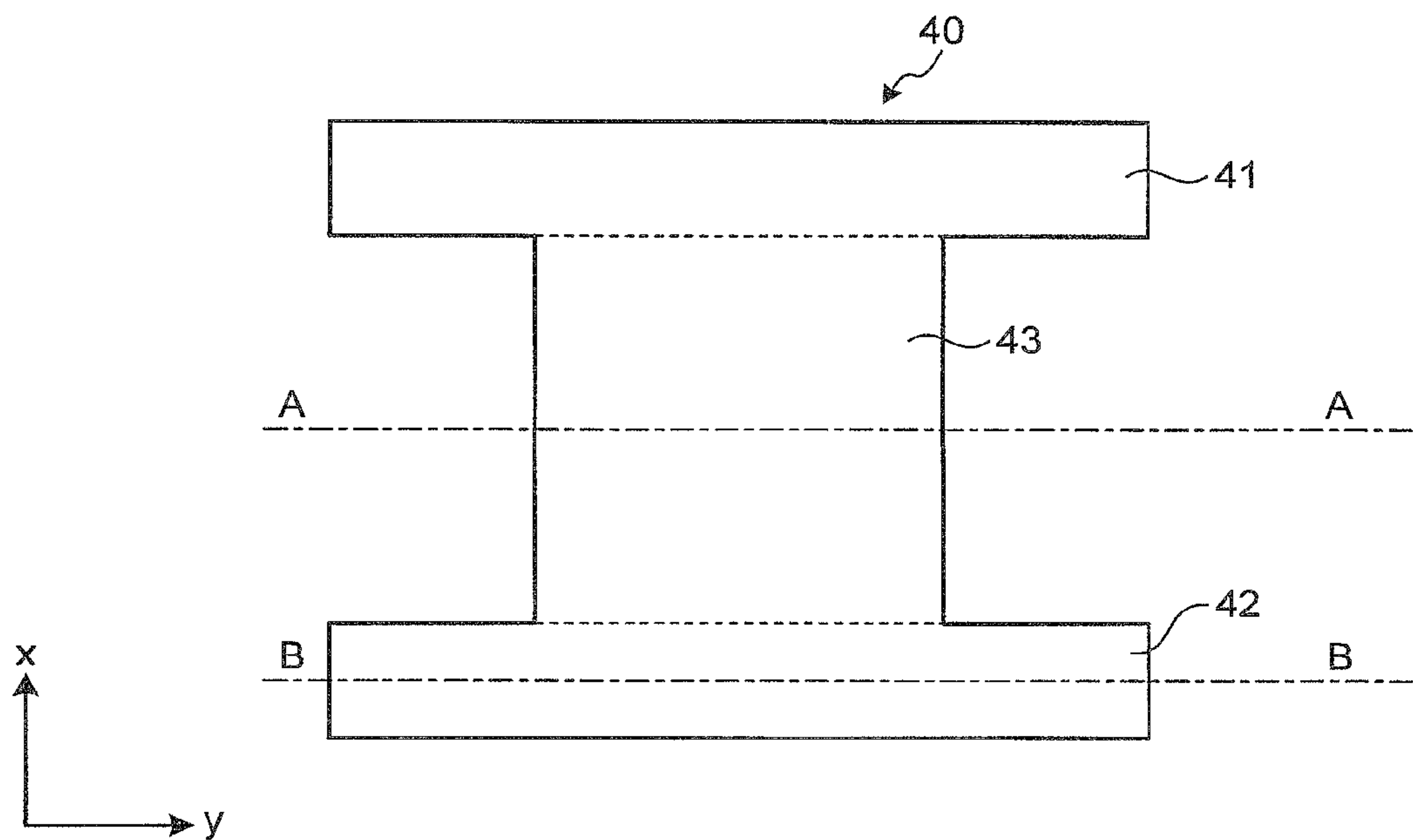
FIG. 20D
