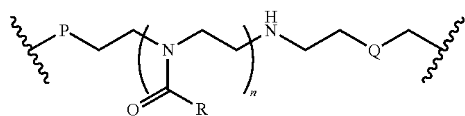
poly(oxazoline)
