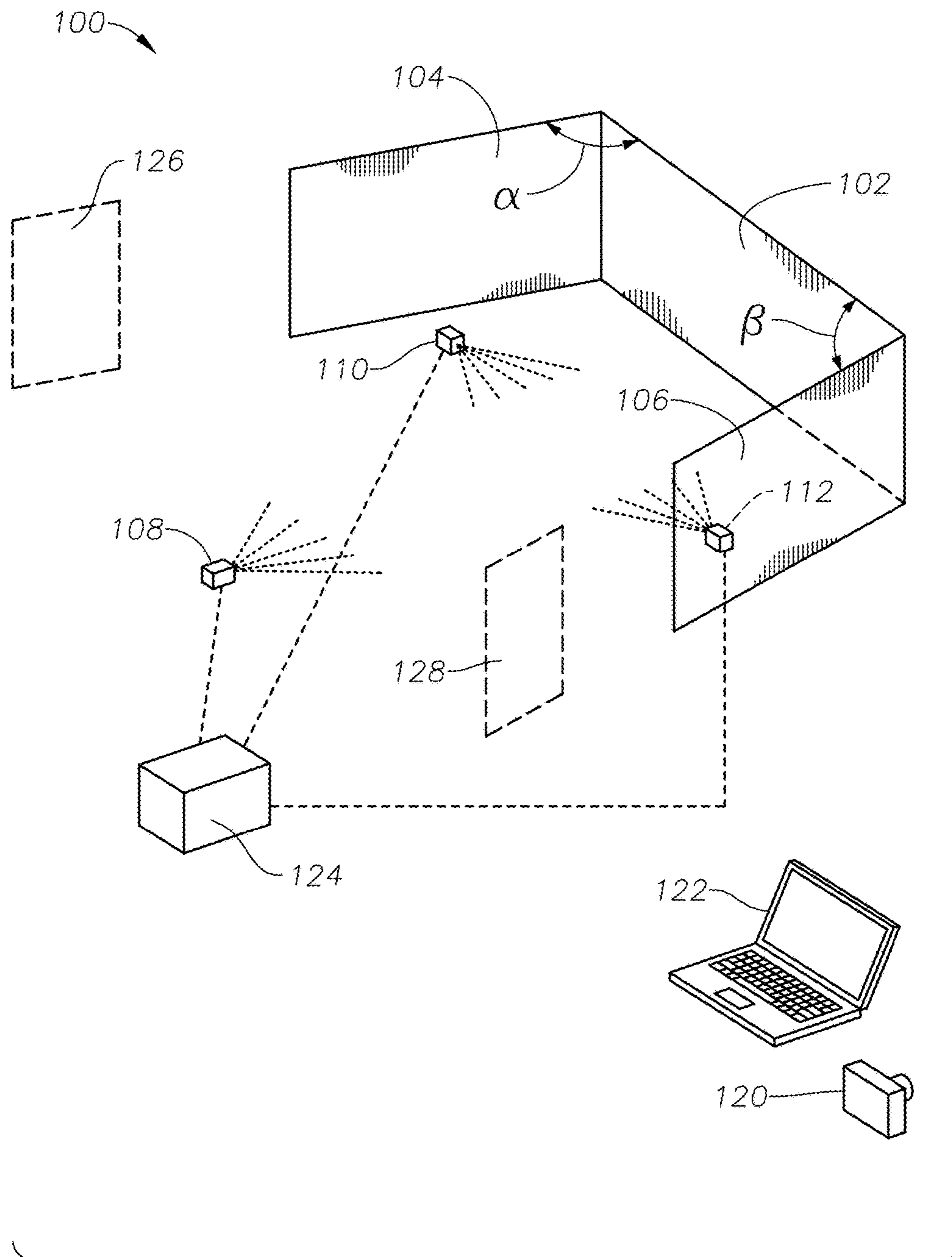
FIG. 16
