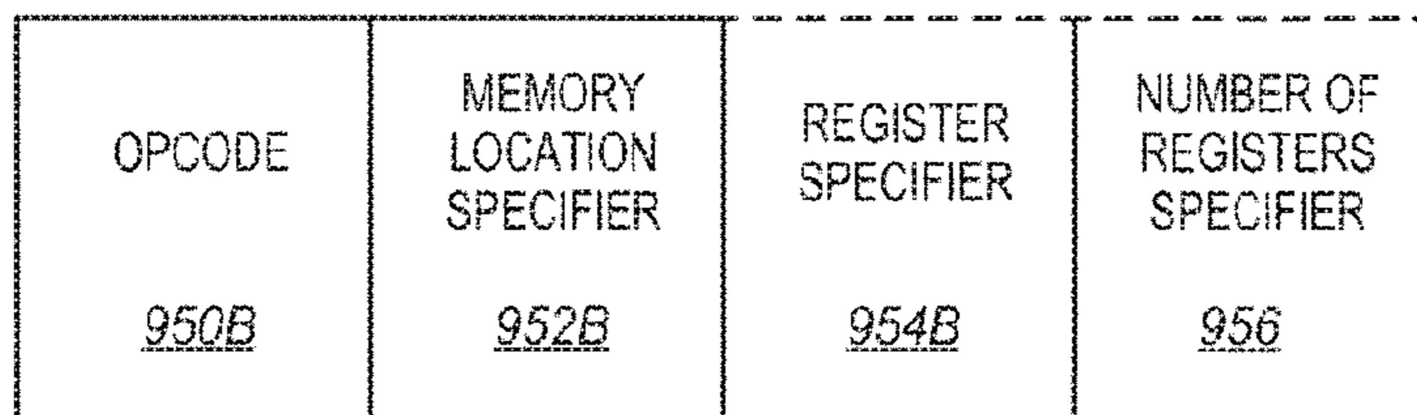
FIG. 9B
