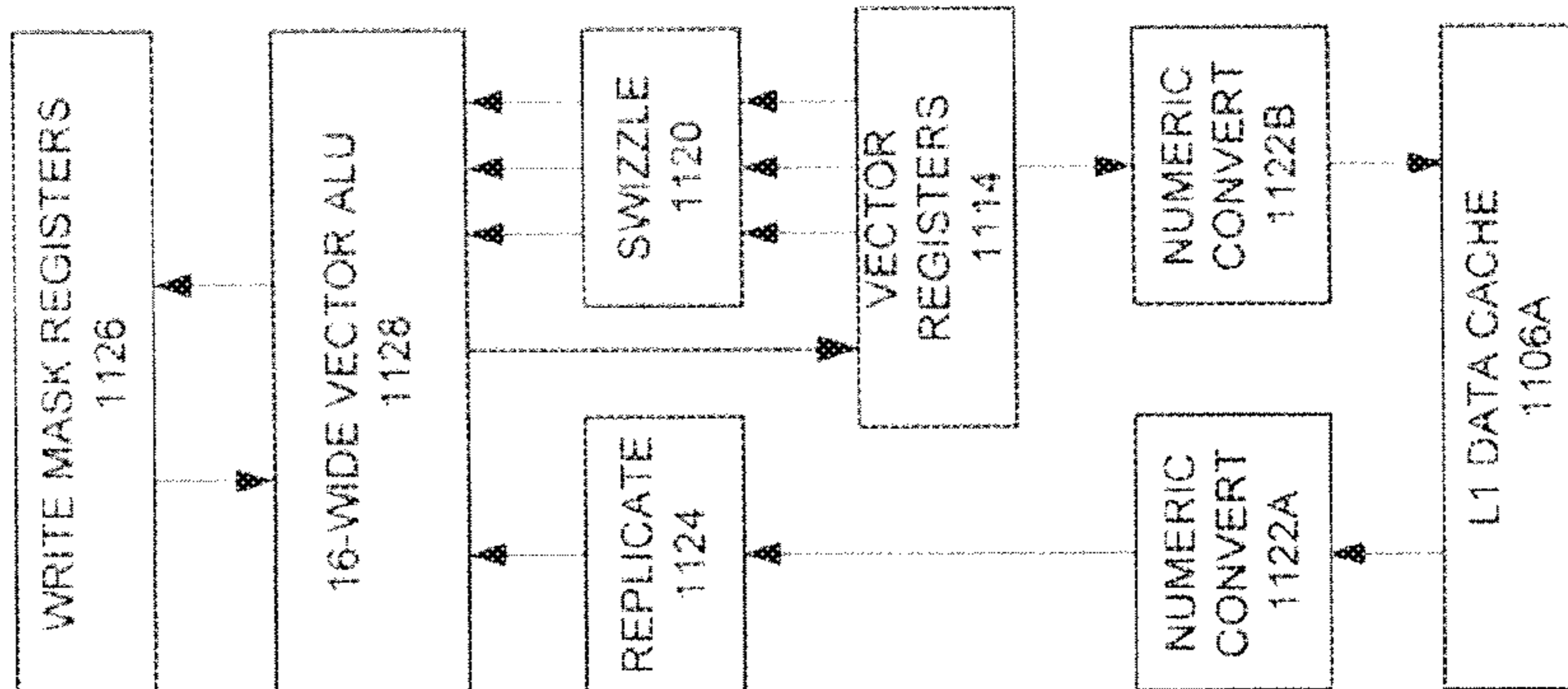
FIG. 11B
