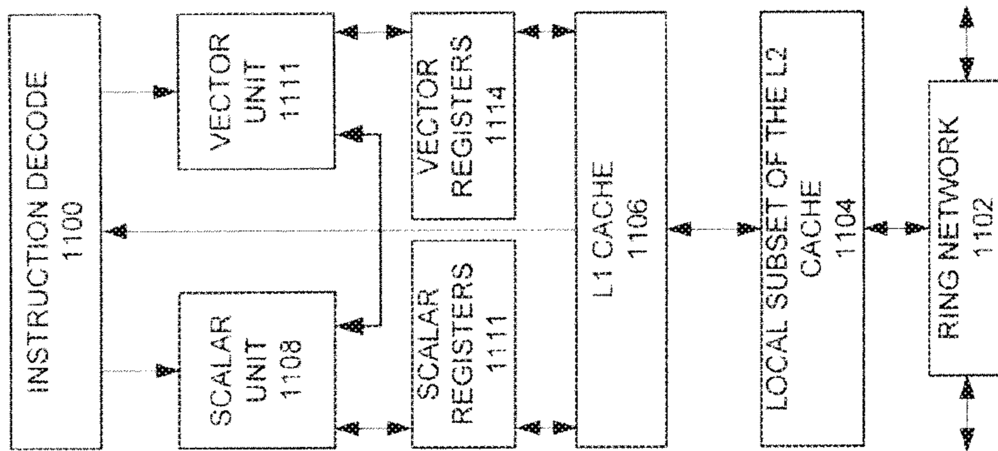
FIG. 11A
