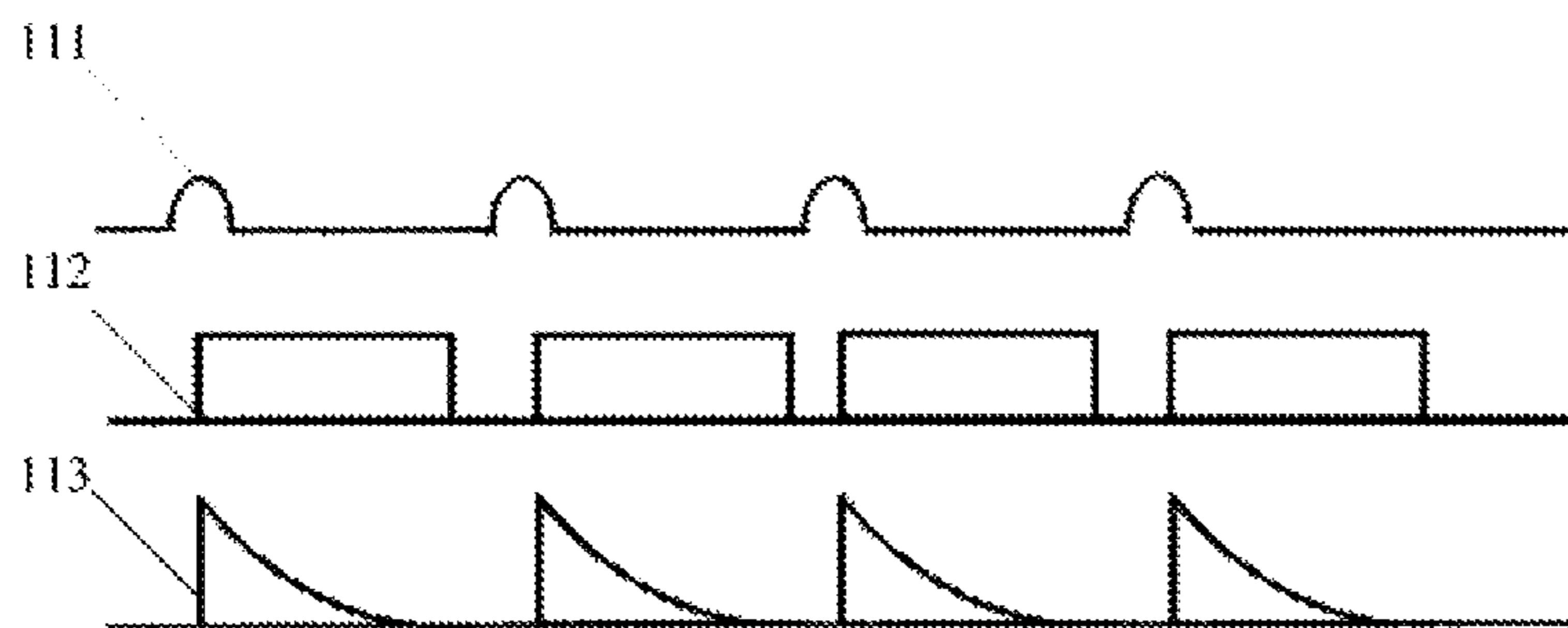
FIG. 3
