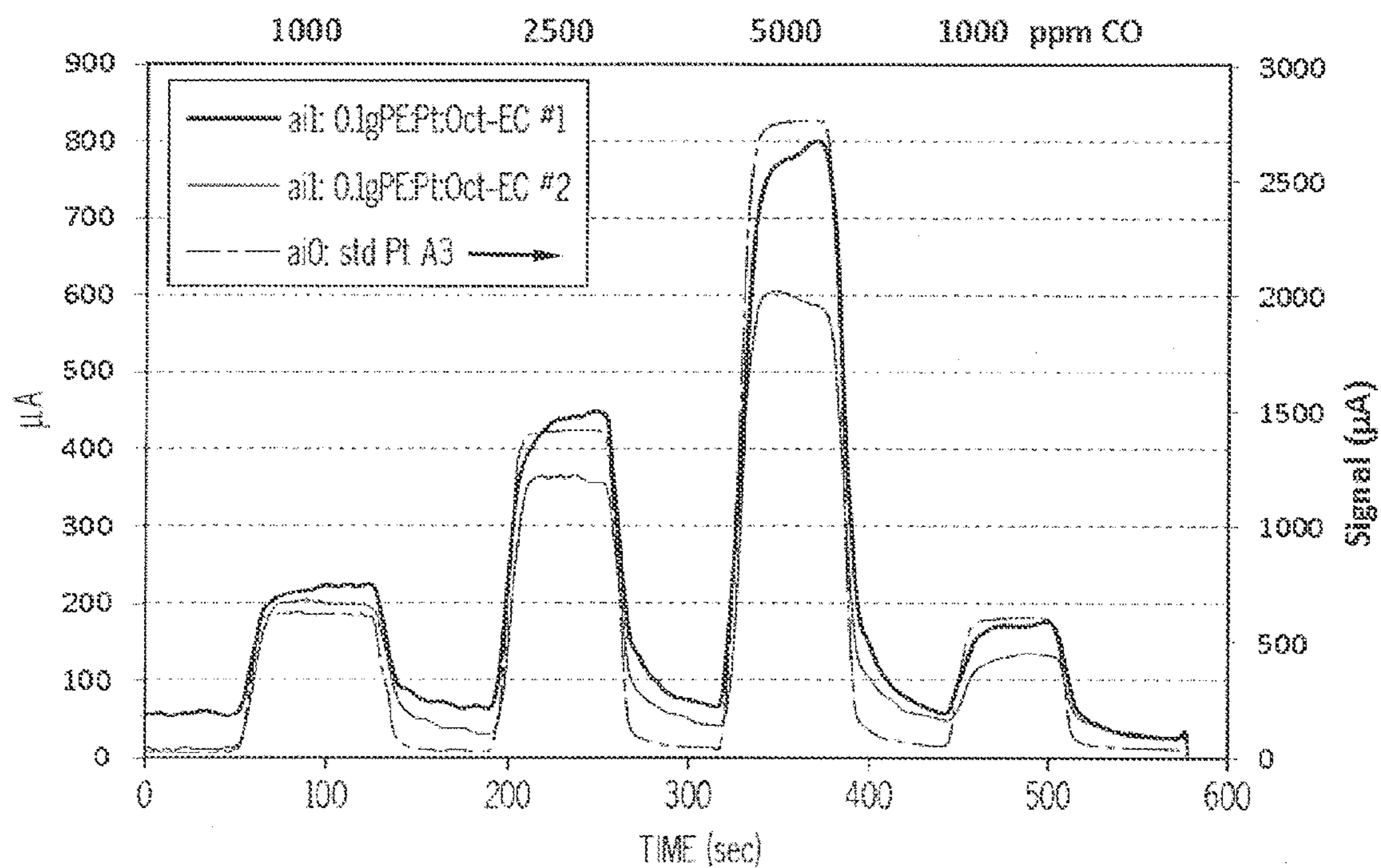
FIG. 16
