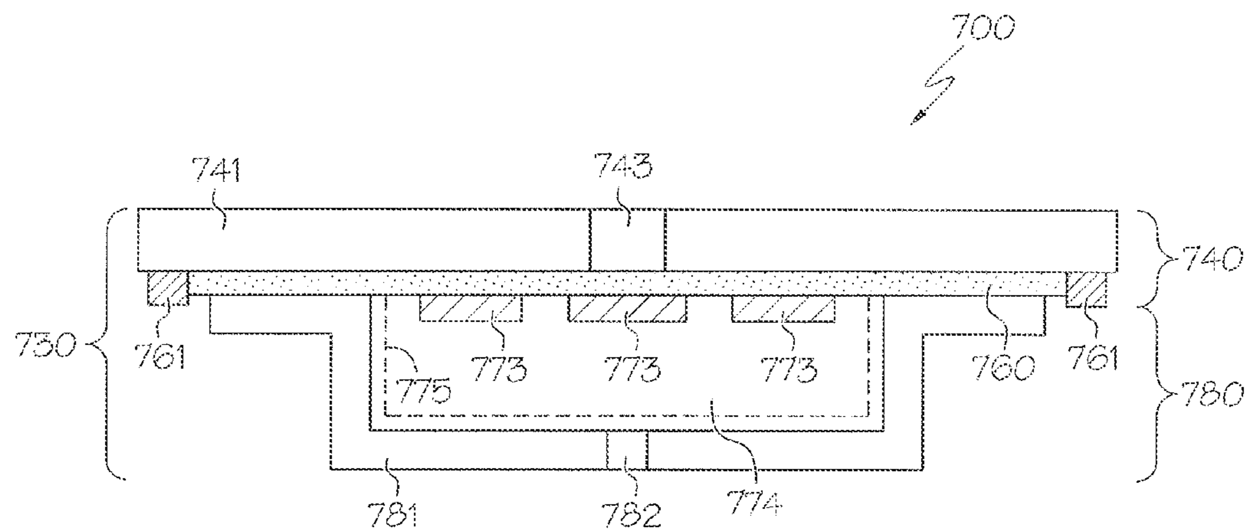
FIG. 12
