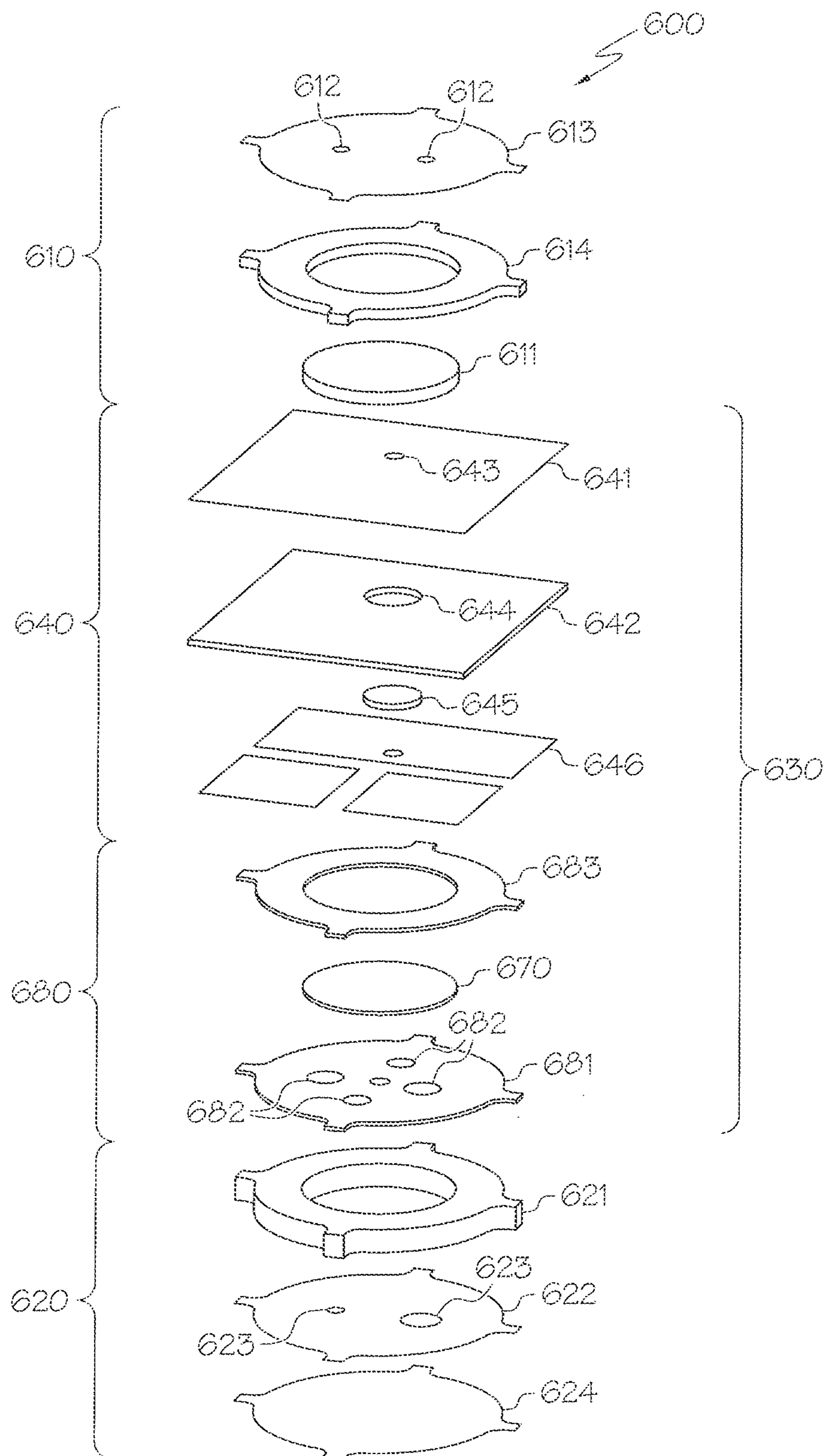
FIG. 11A
