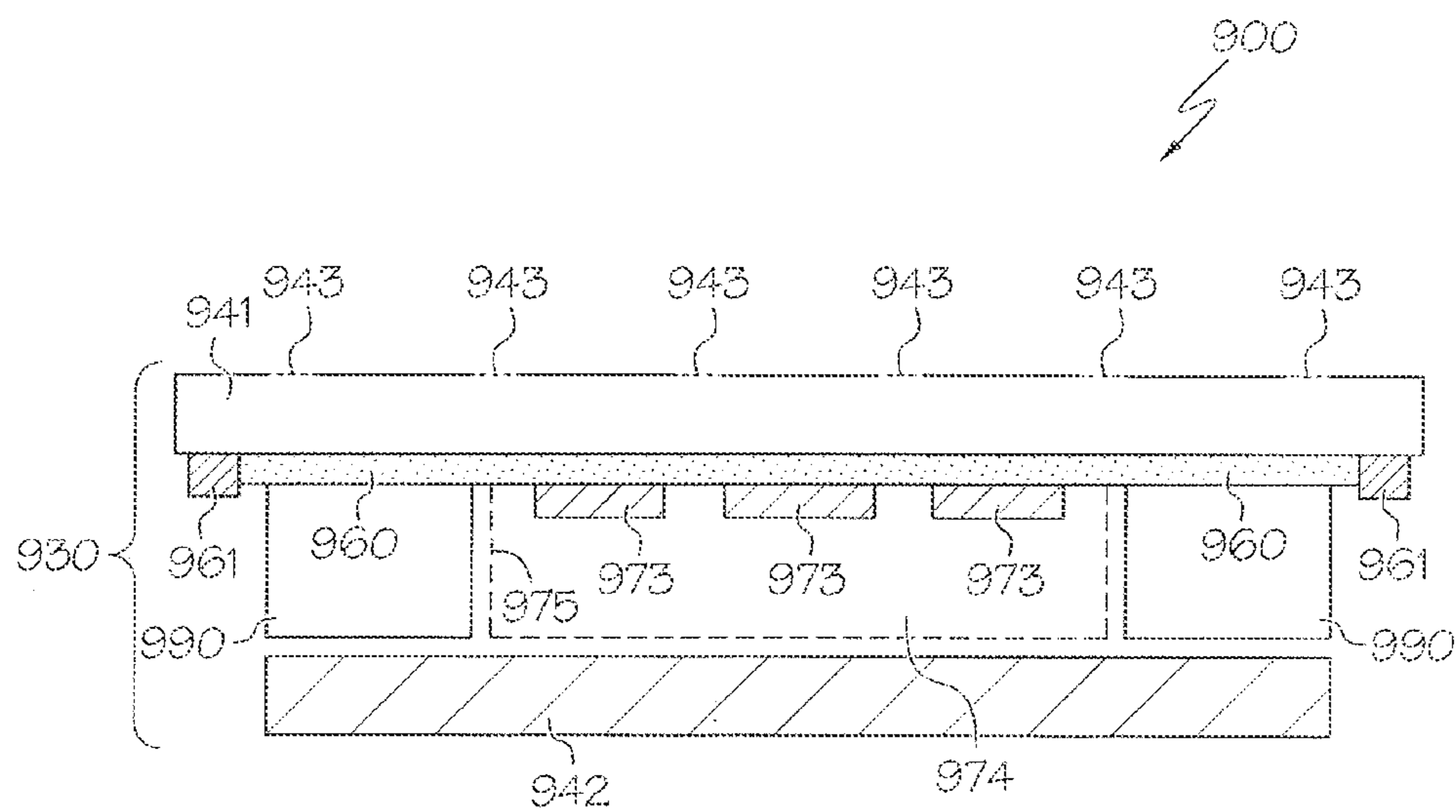
FIG. 13
