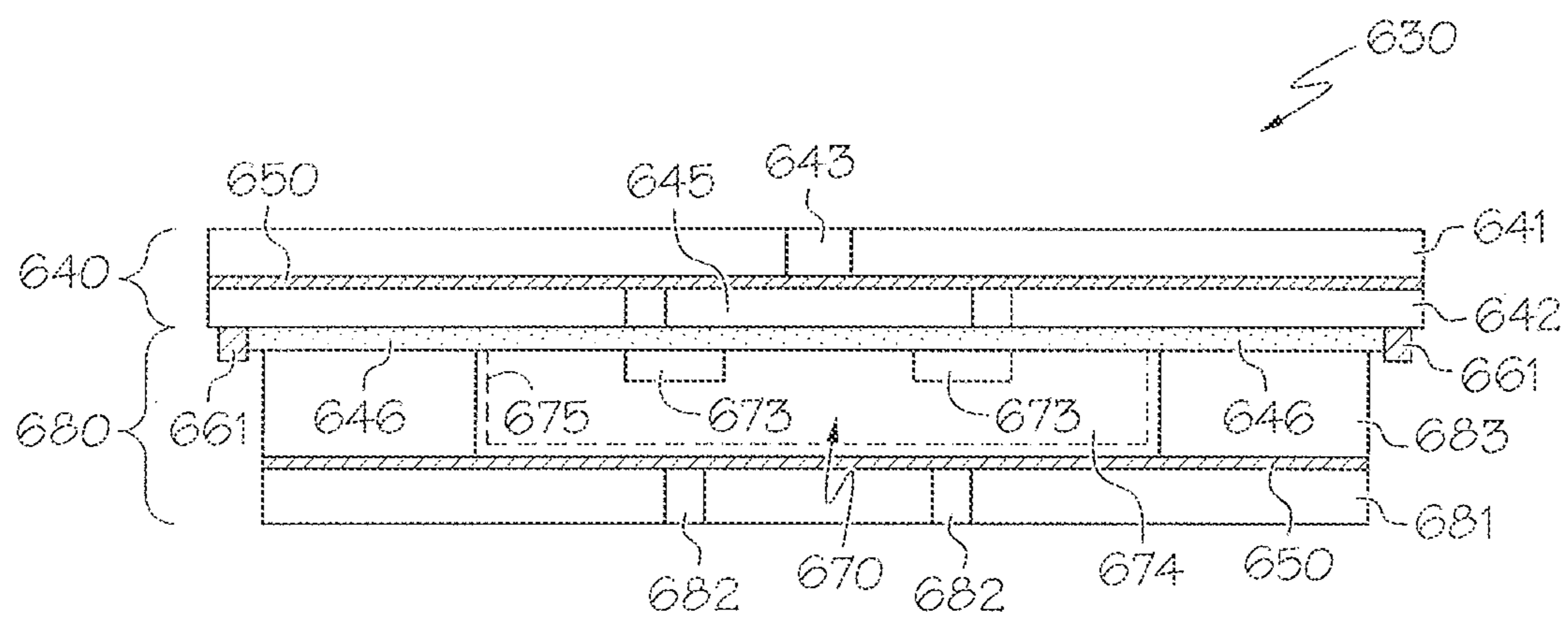
FIG. 10
