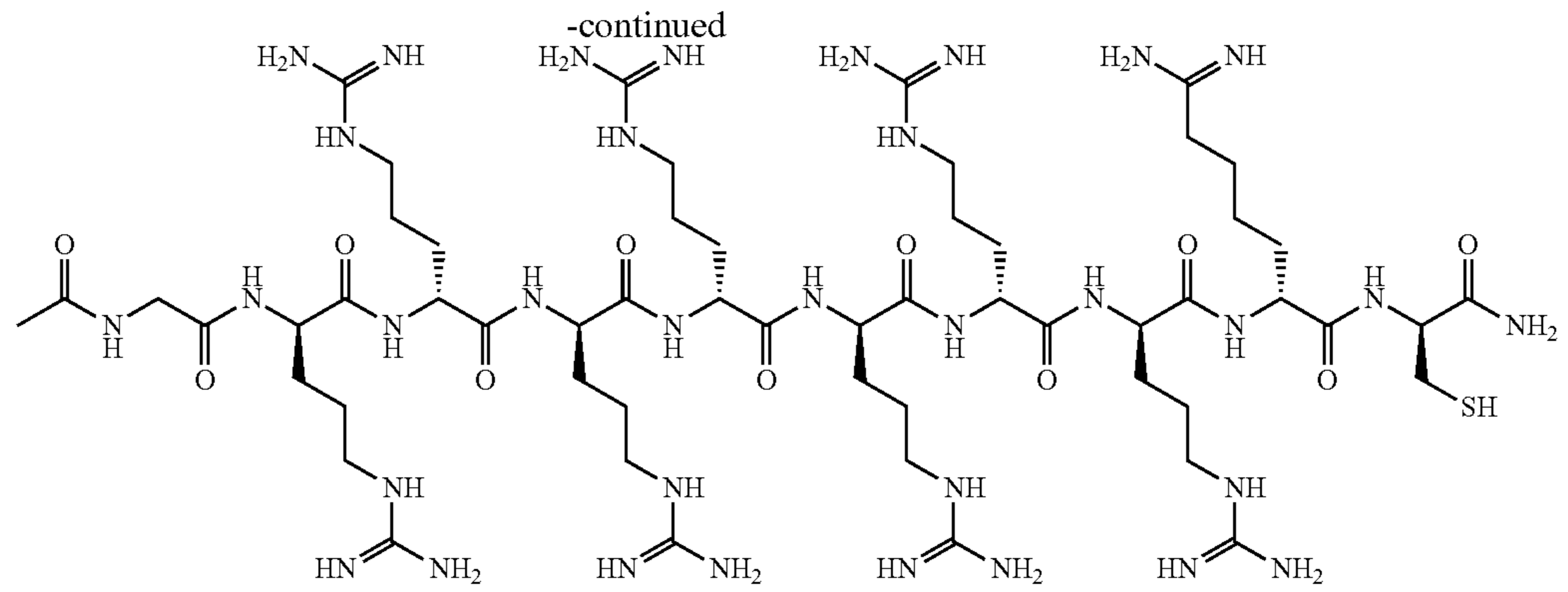
Peptide P-2
