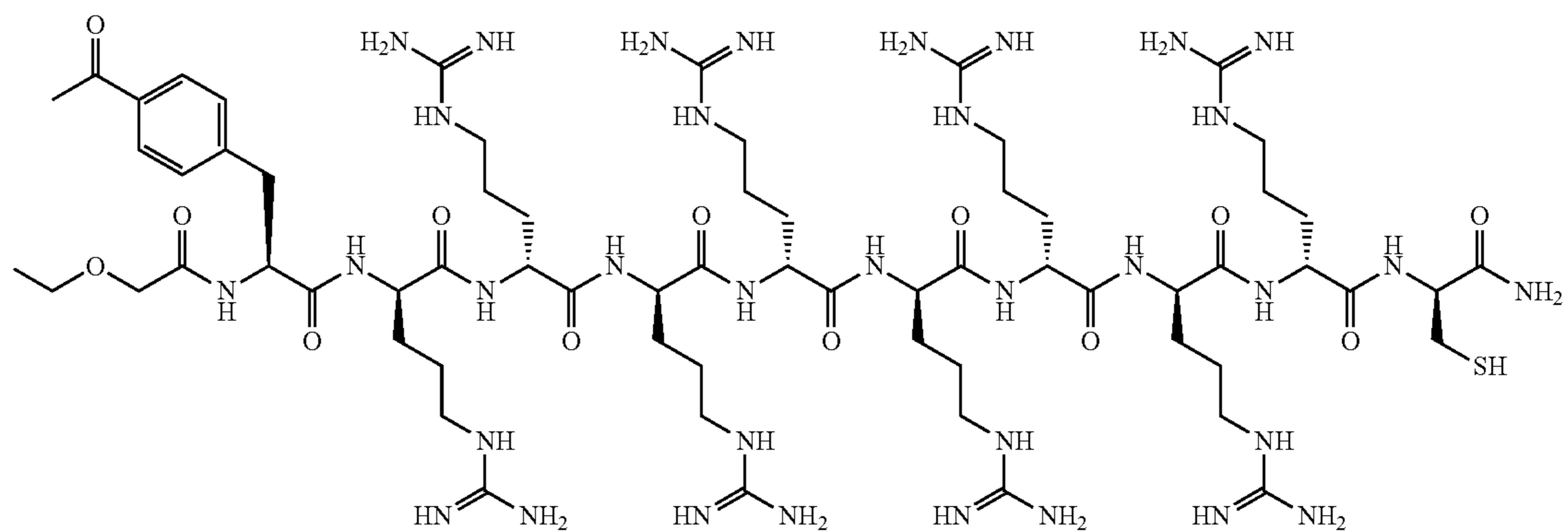
Peptide P-6
