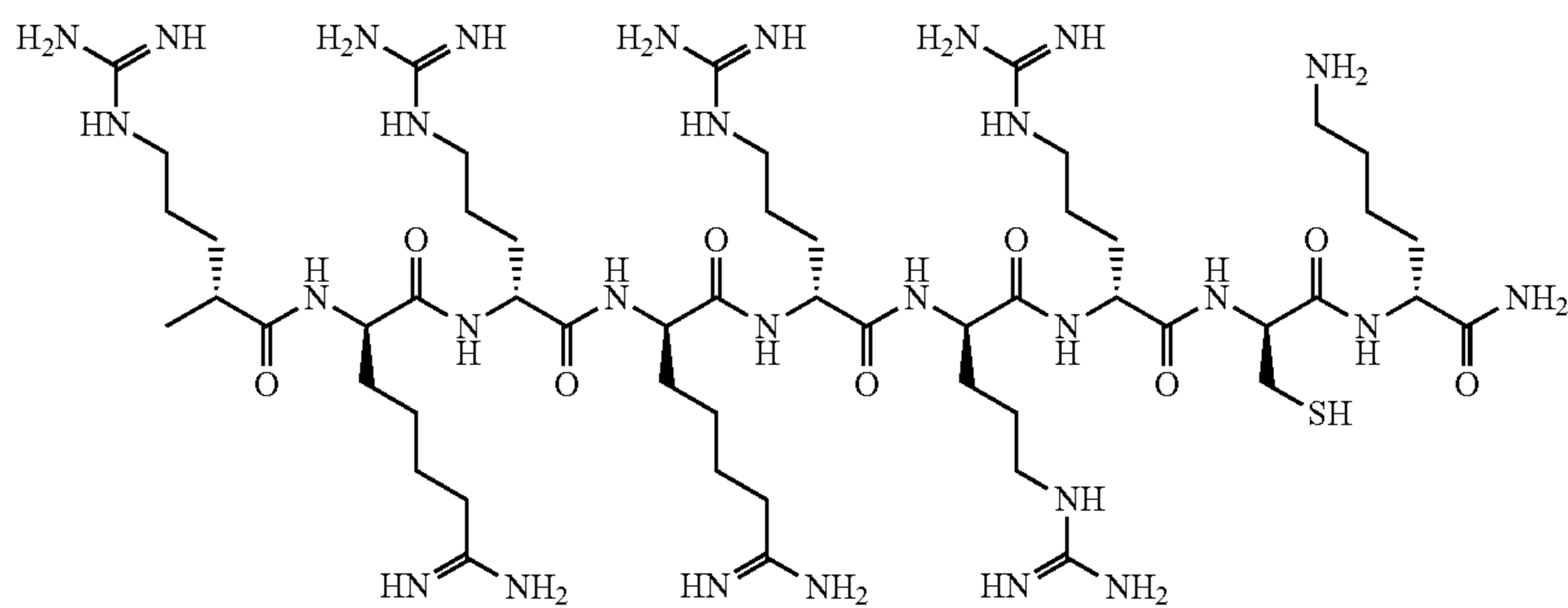
Peptide P-5
