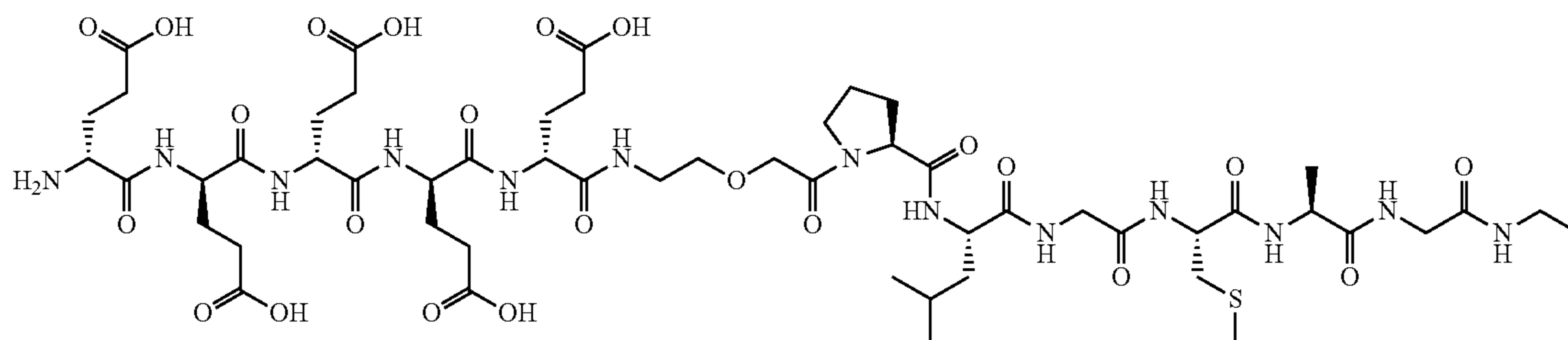
Peptide P-5
