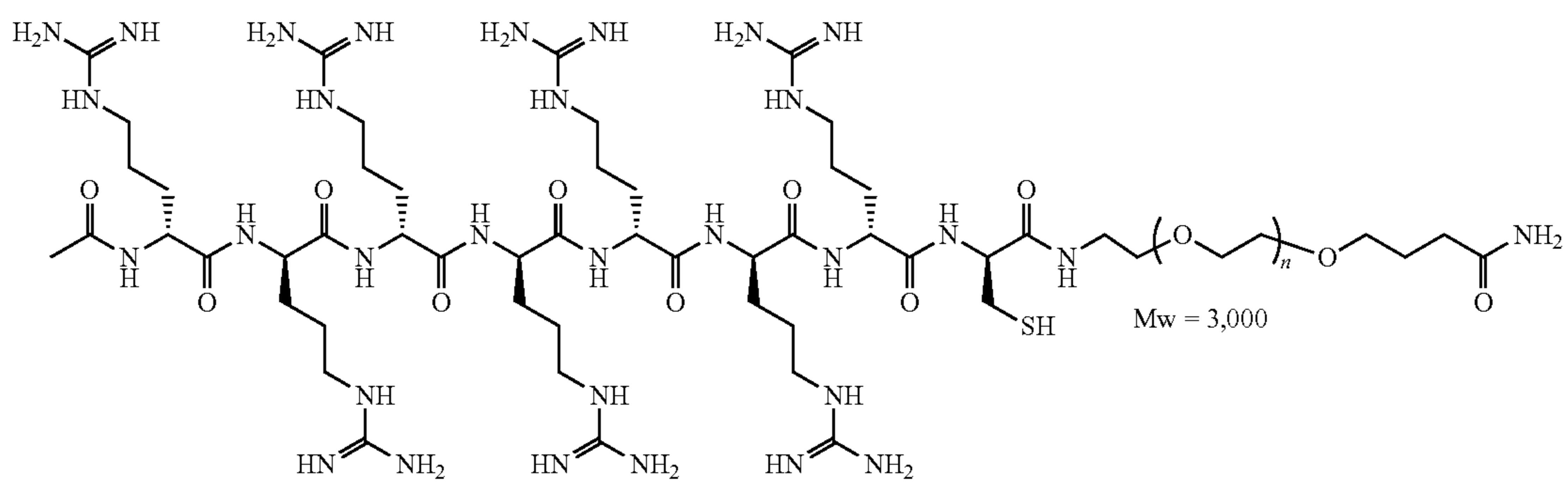
Peptide P-10
