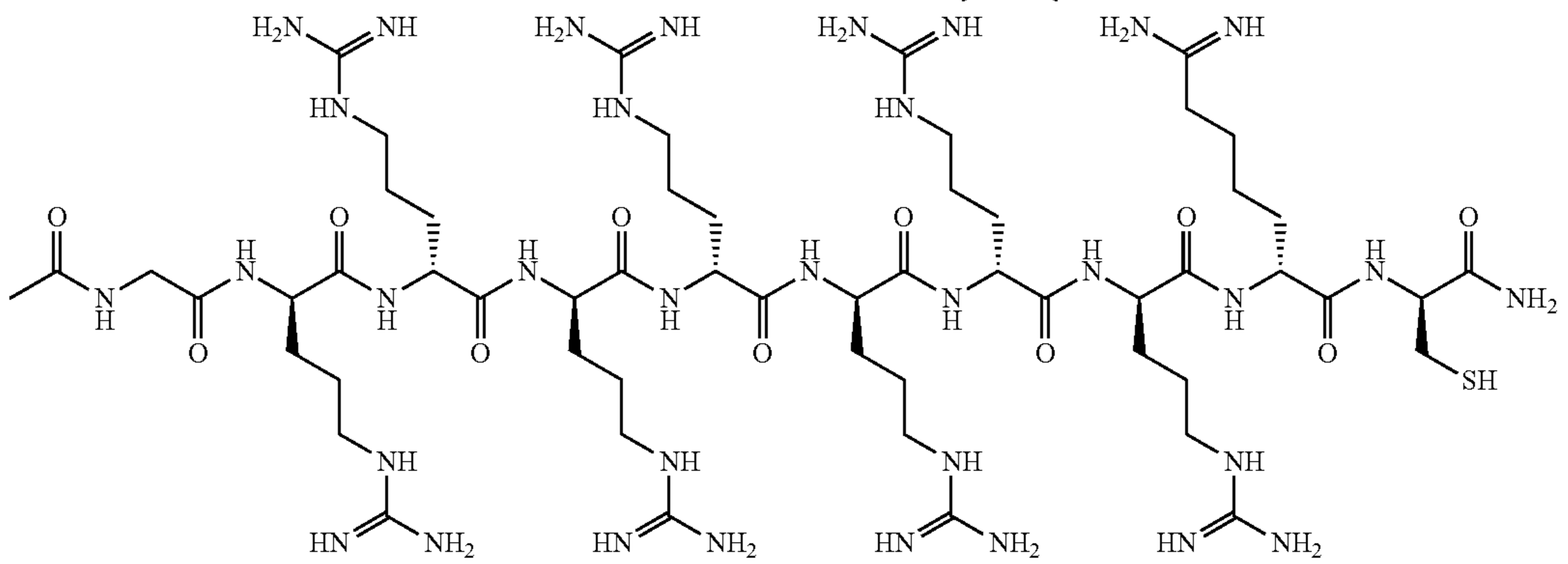
Peptide P-3
