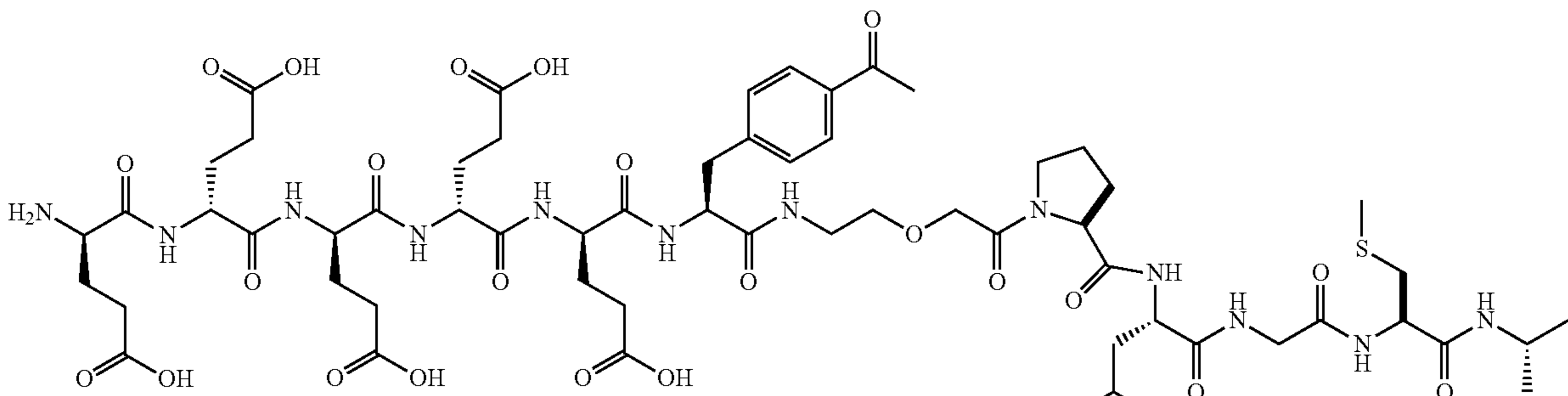
Peptide P-2
