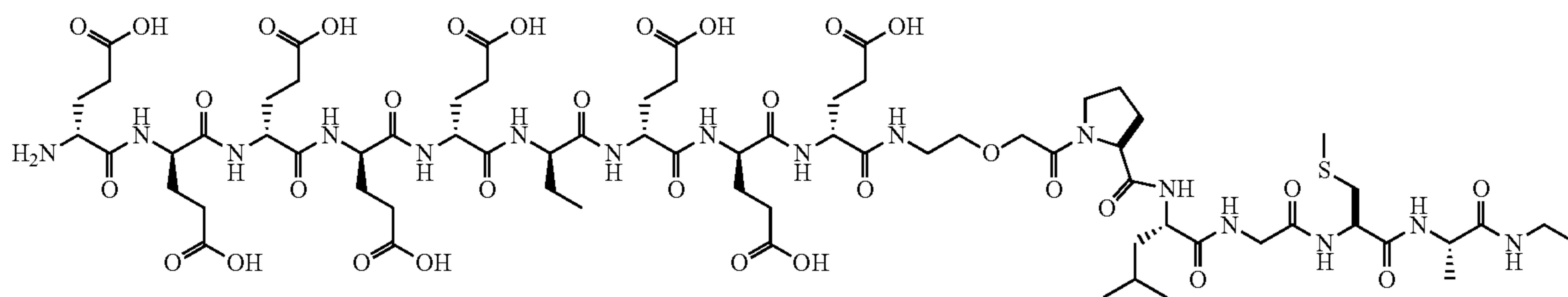
Peptide P-6
