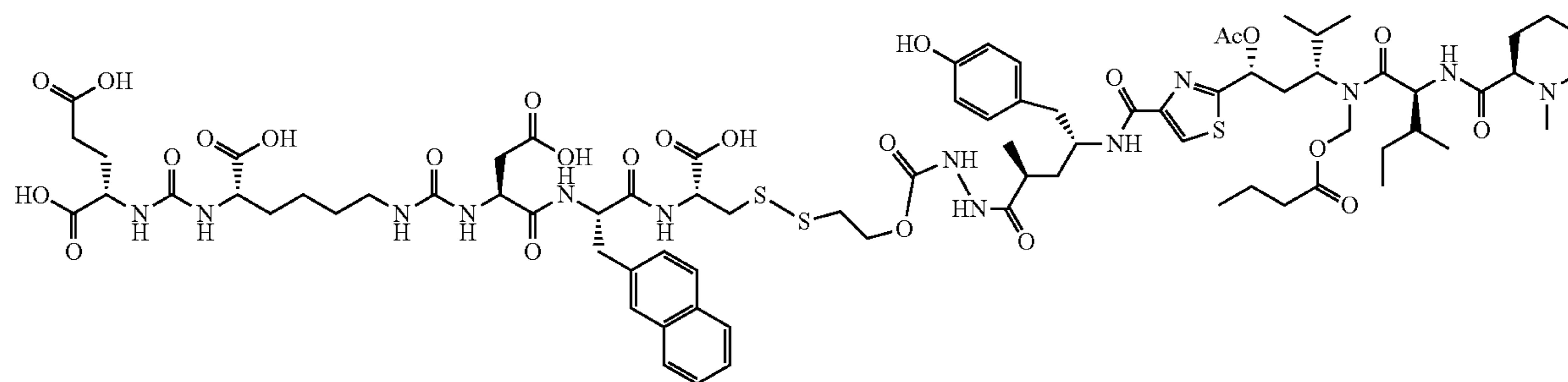
EC1387 Exact Mass: 1723.68 Mol. Wt.: 1724.97
