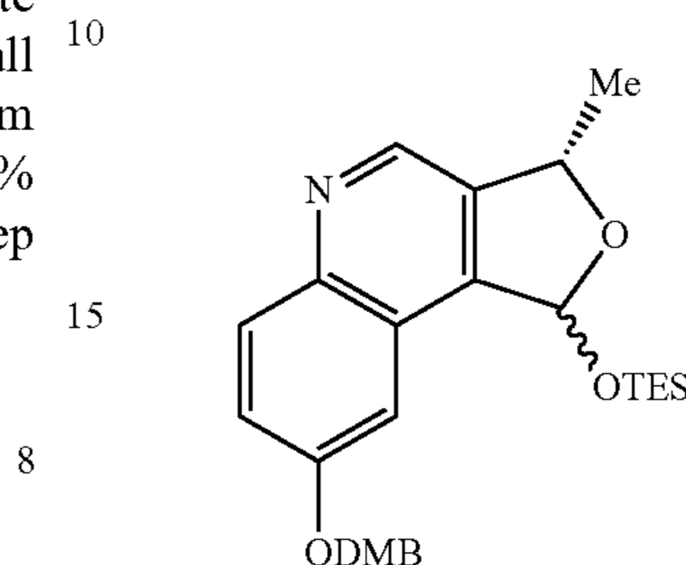
TES Lactol 10.
