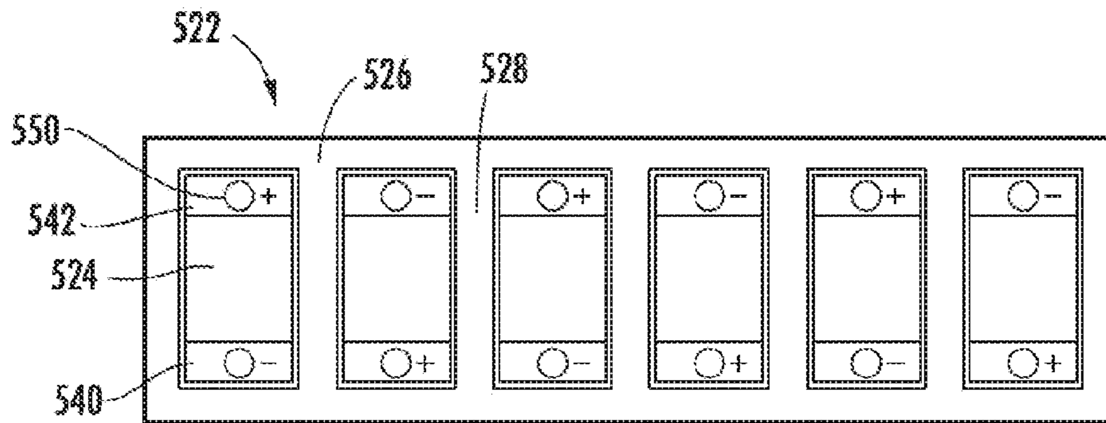
FIG. 10
