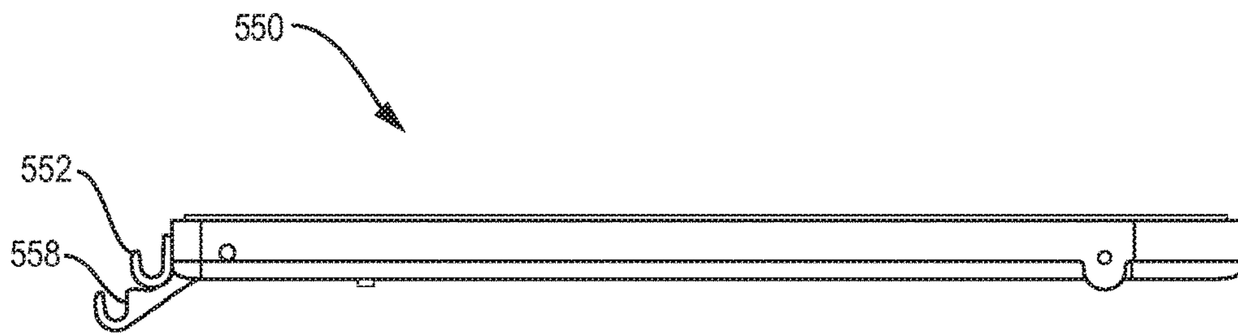
FIG. 24D
