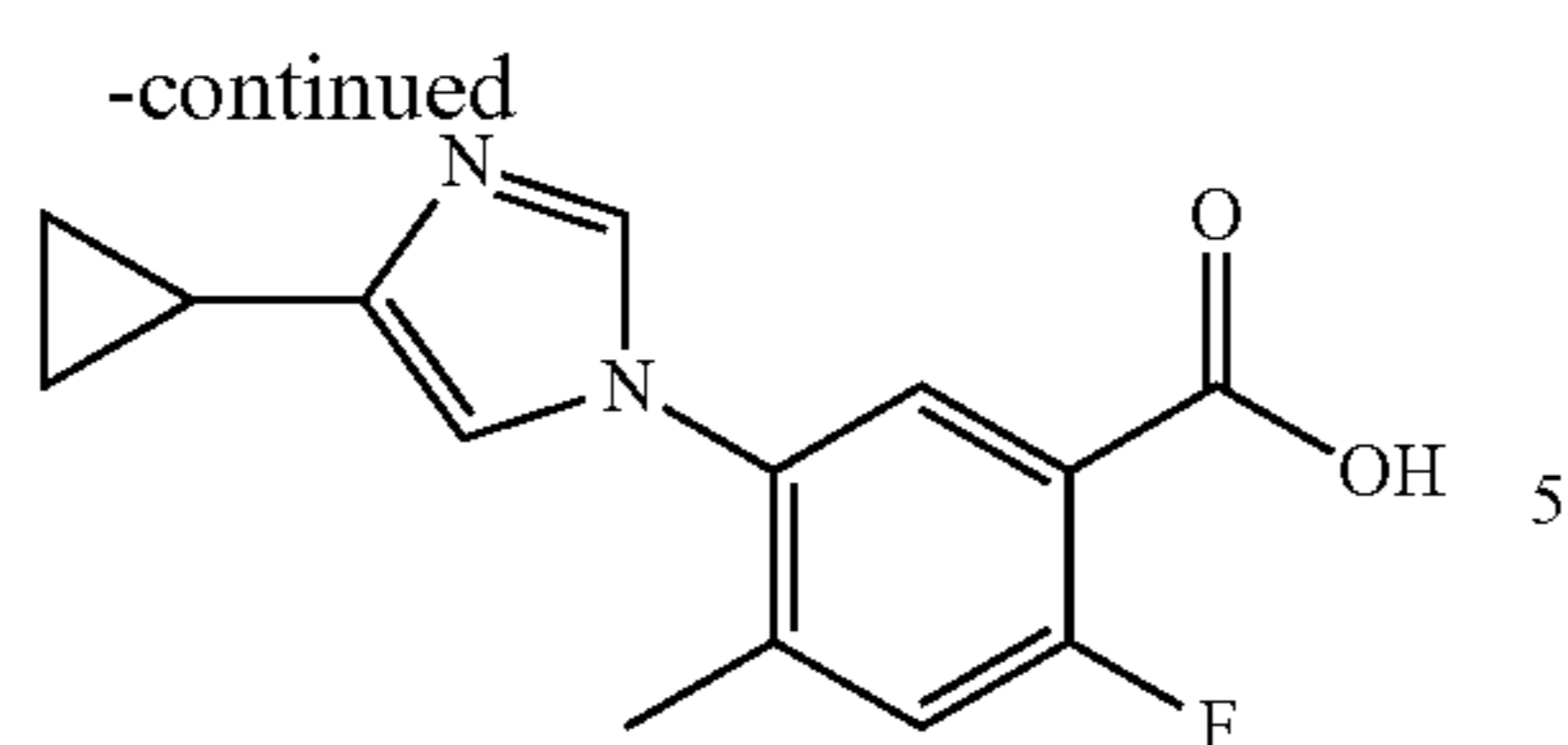
Compound (D)
