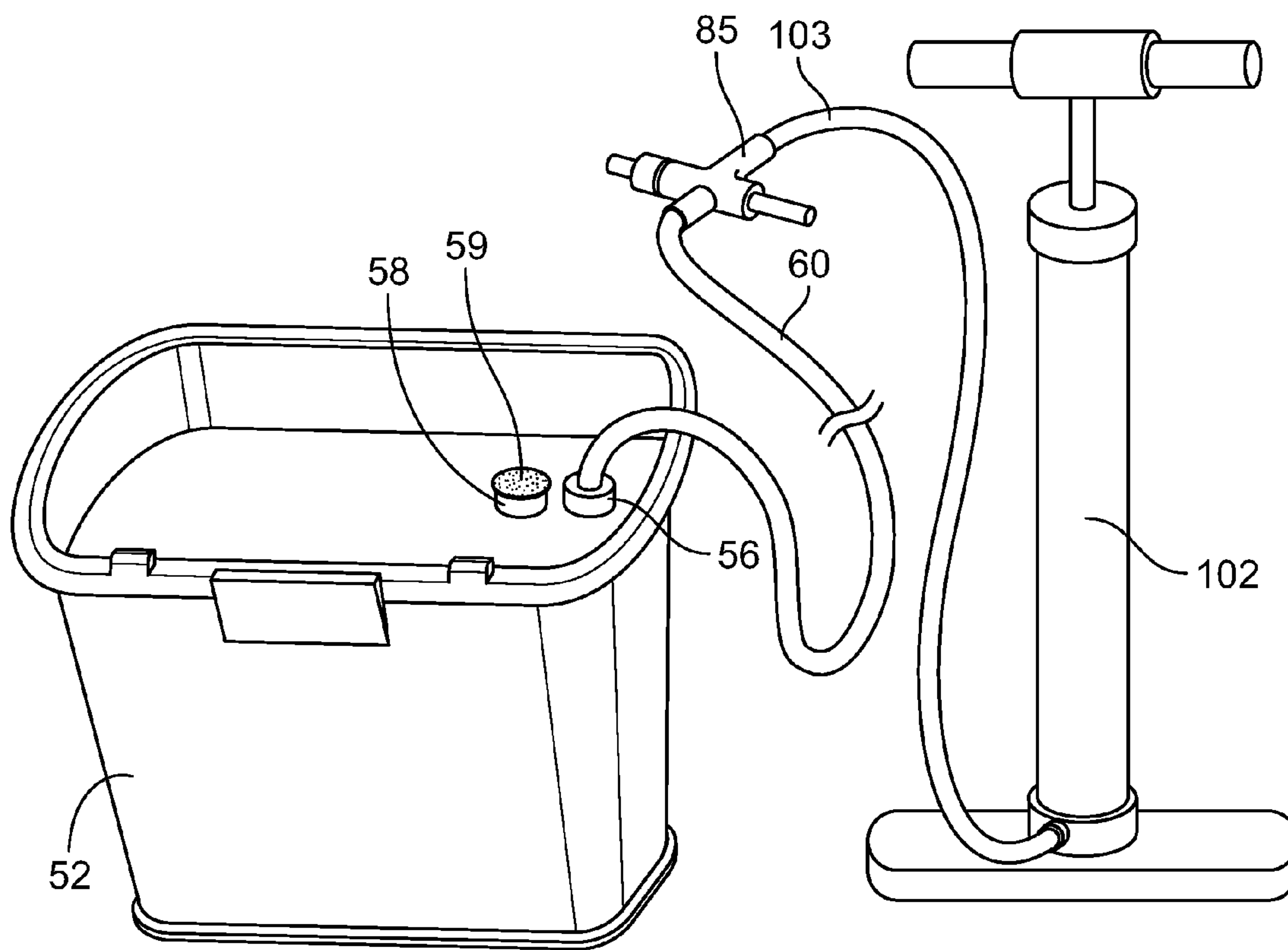
FIG. 13
