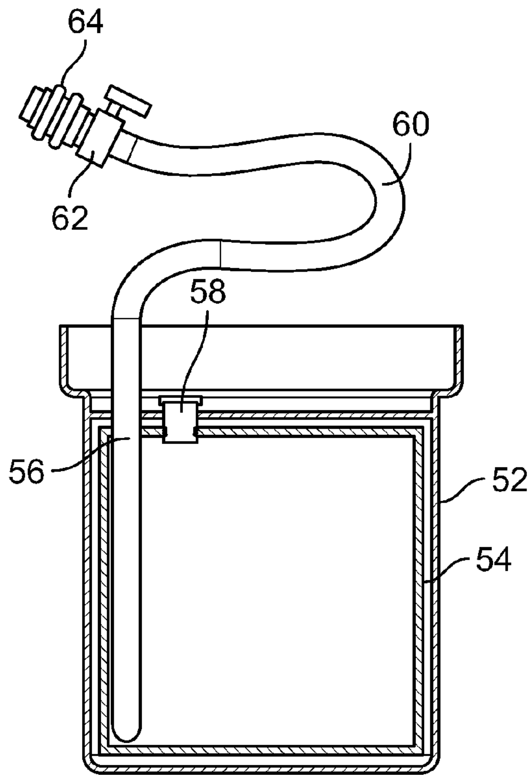
FIG. 9
