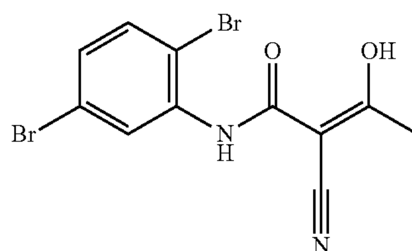
LFM-A13
