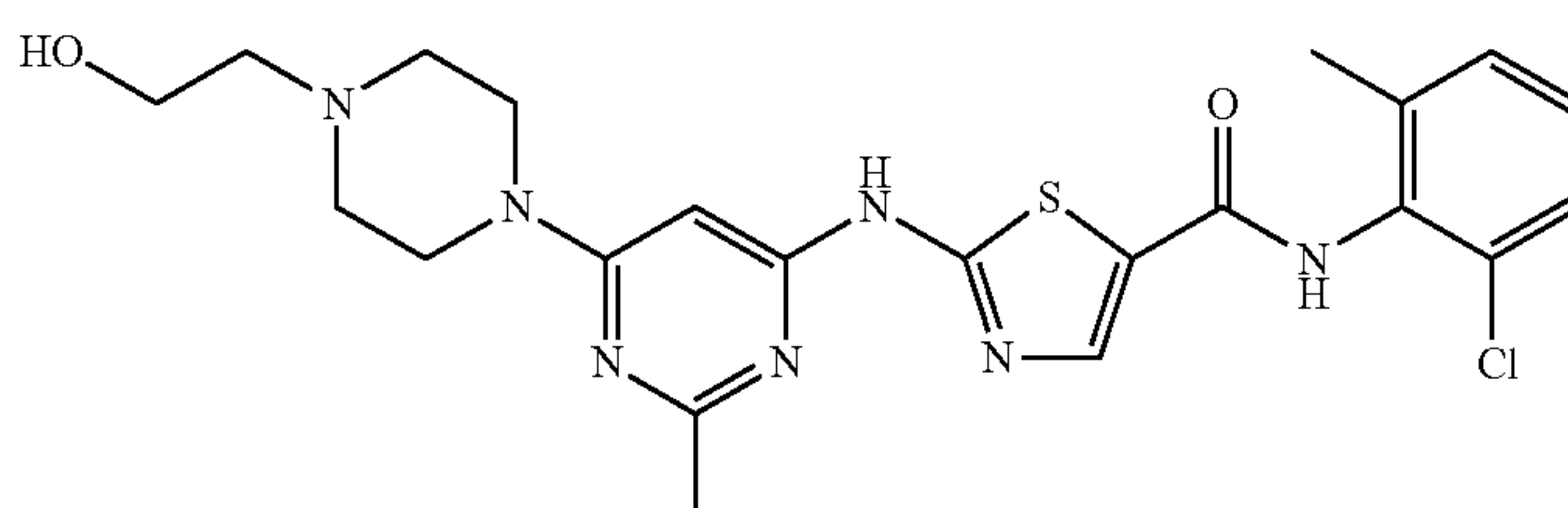
Dasatinib
