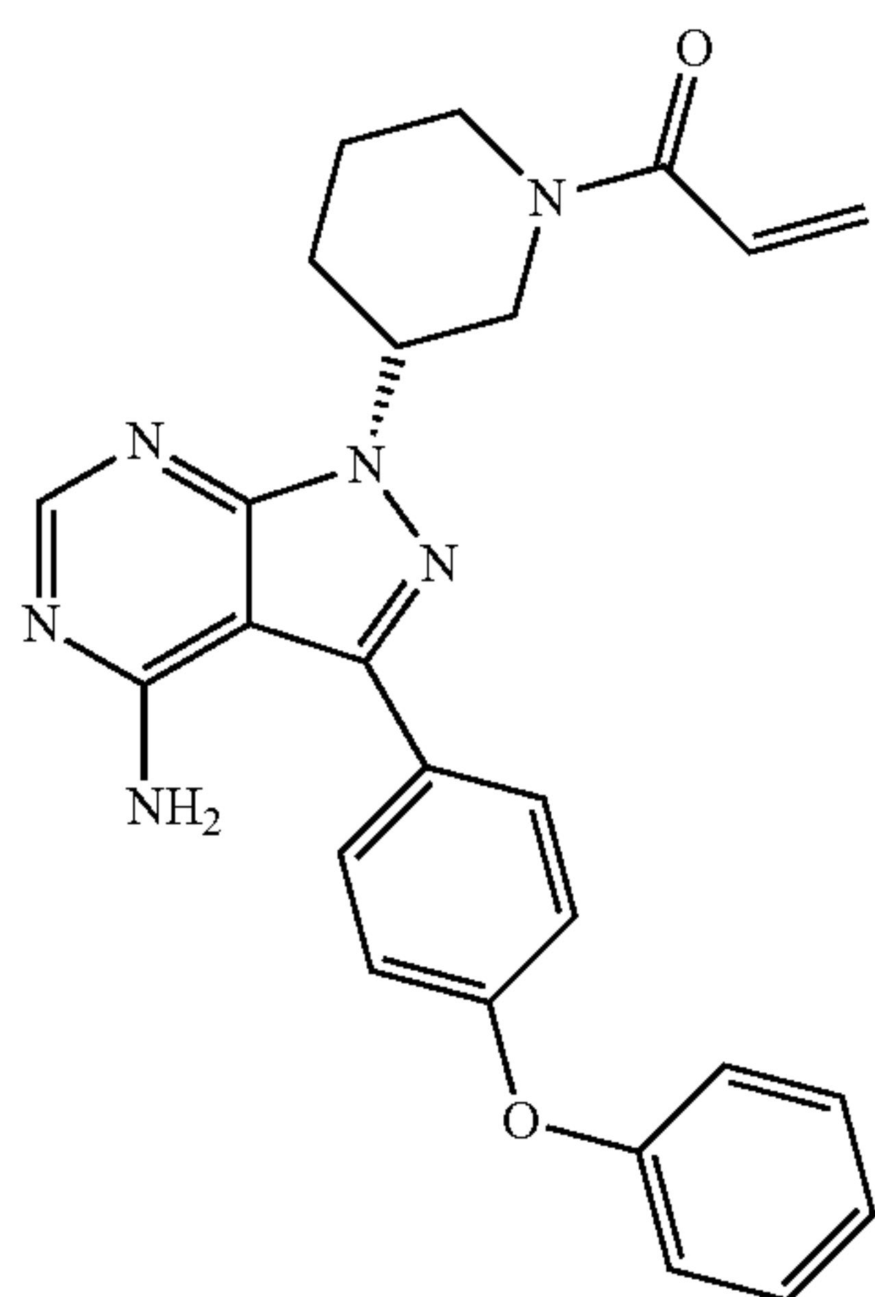
Ibrutinib
