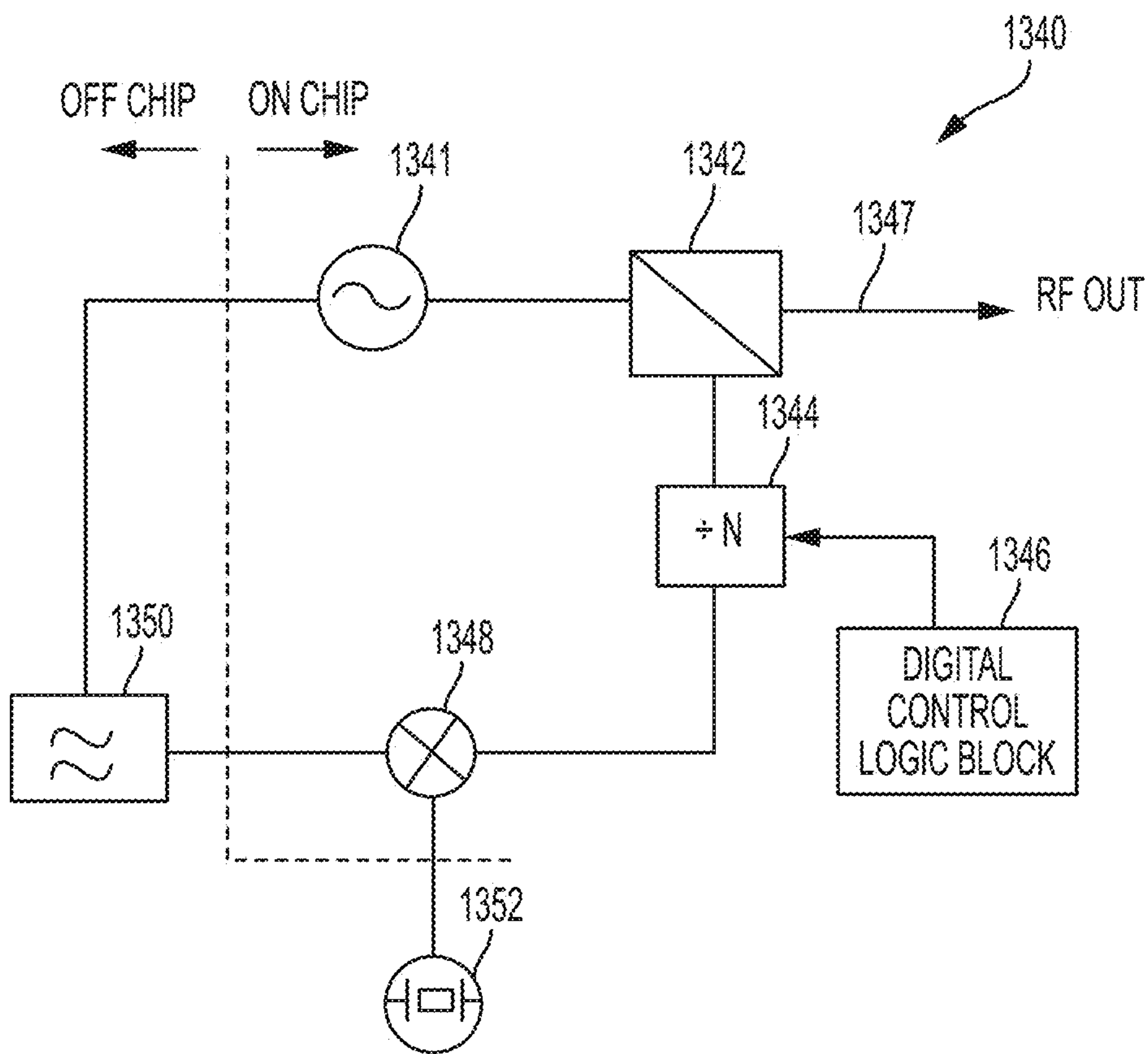
FIG. 13C
