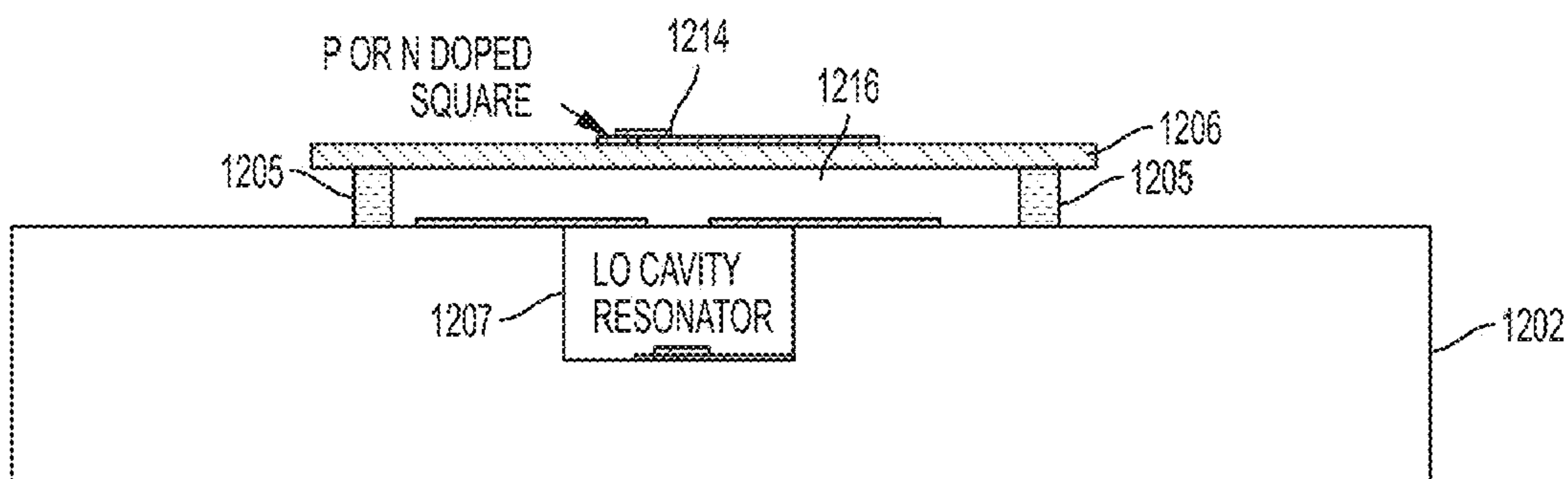
FIG. 12B
