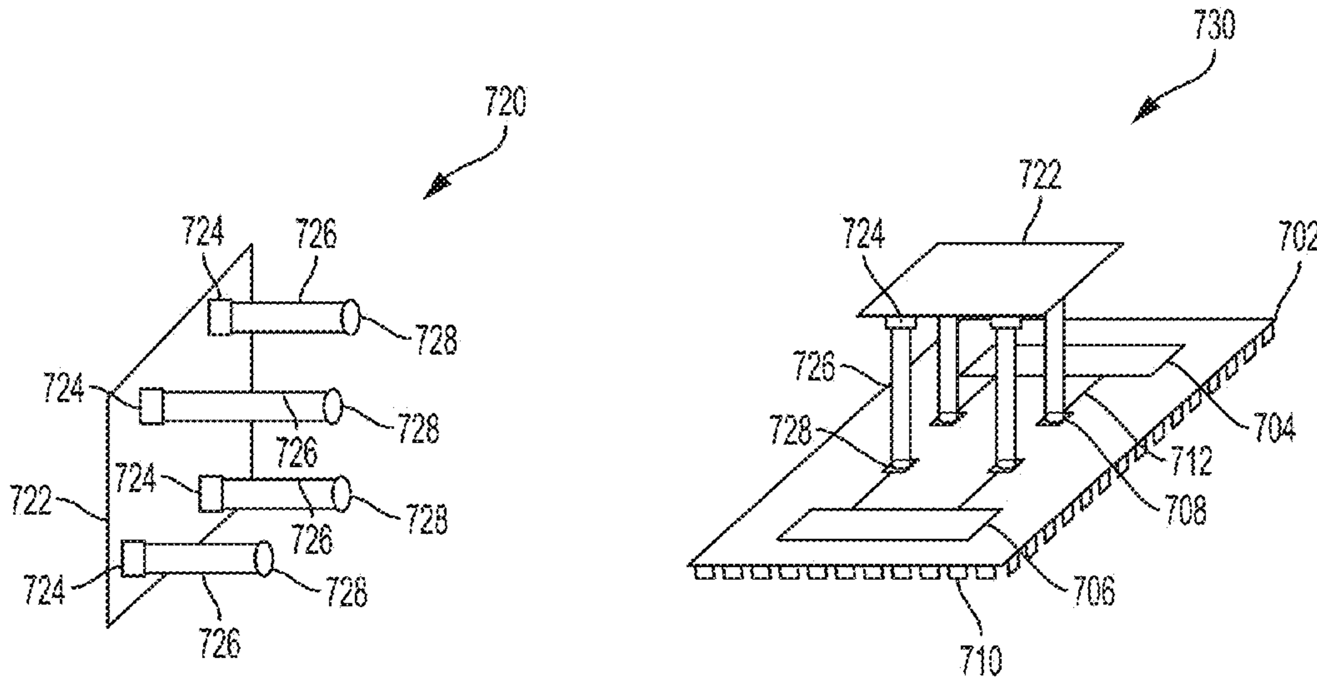
FIG. 7B
