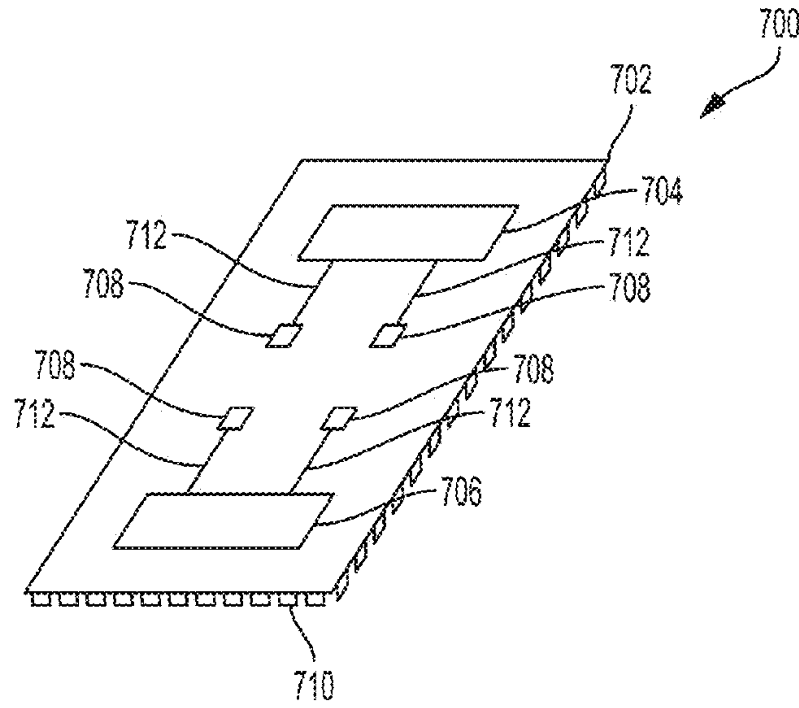
FIG. 7A
