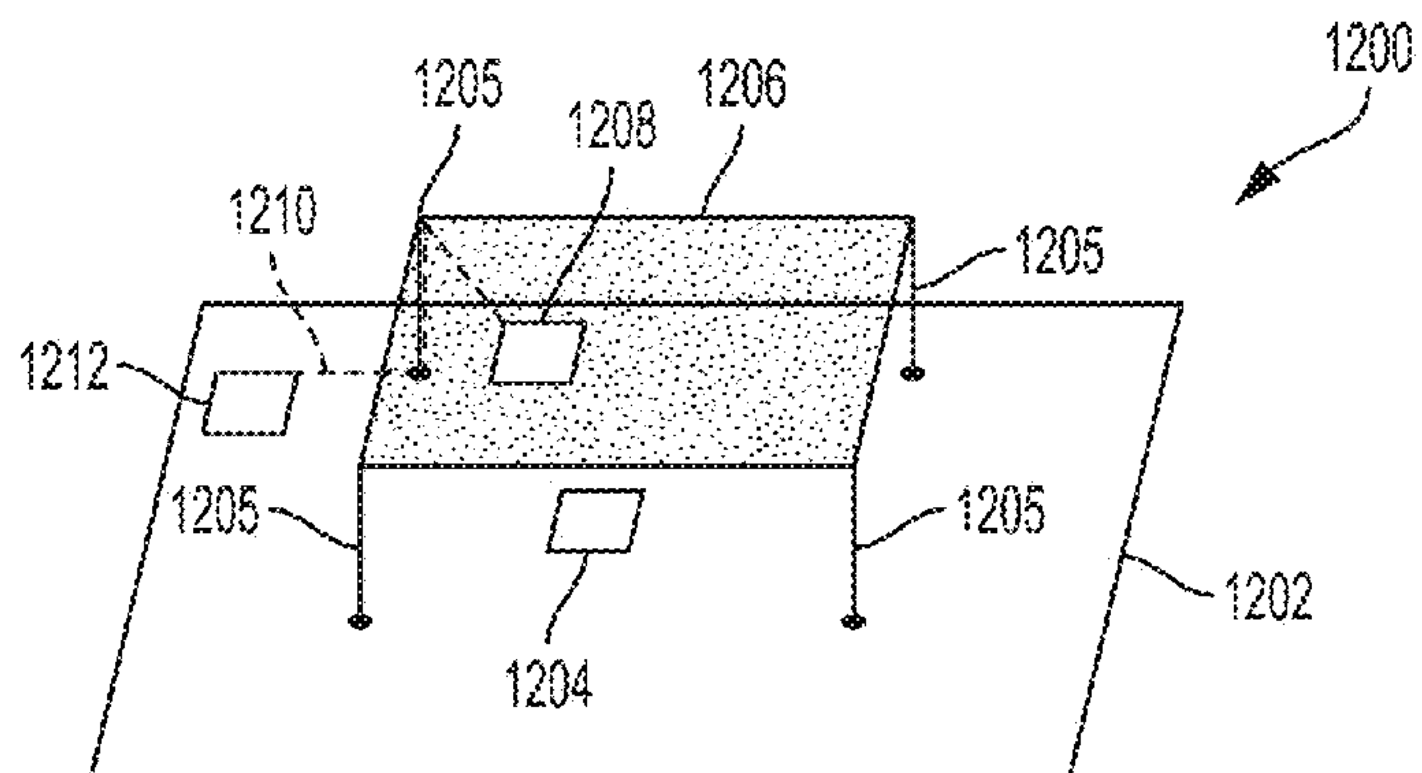
FIG. 12A
