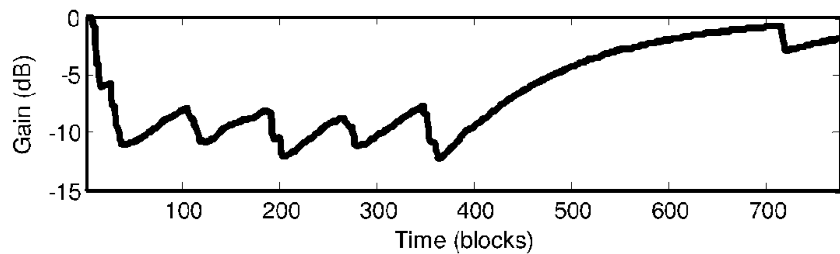
FIG. 10b b) DRC gain
