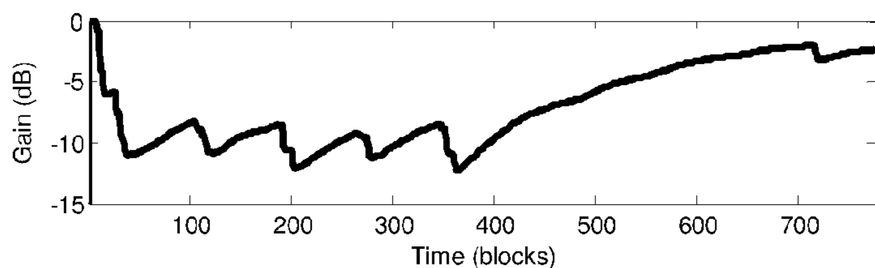
FIG. 10e e) Event-controlled DRC gain
