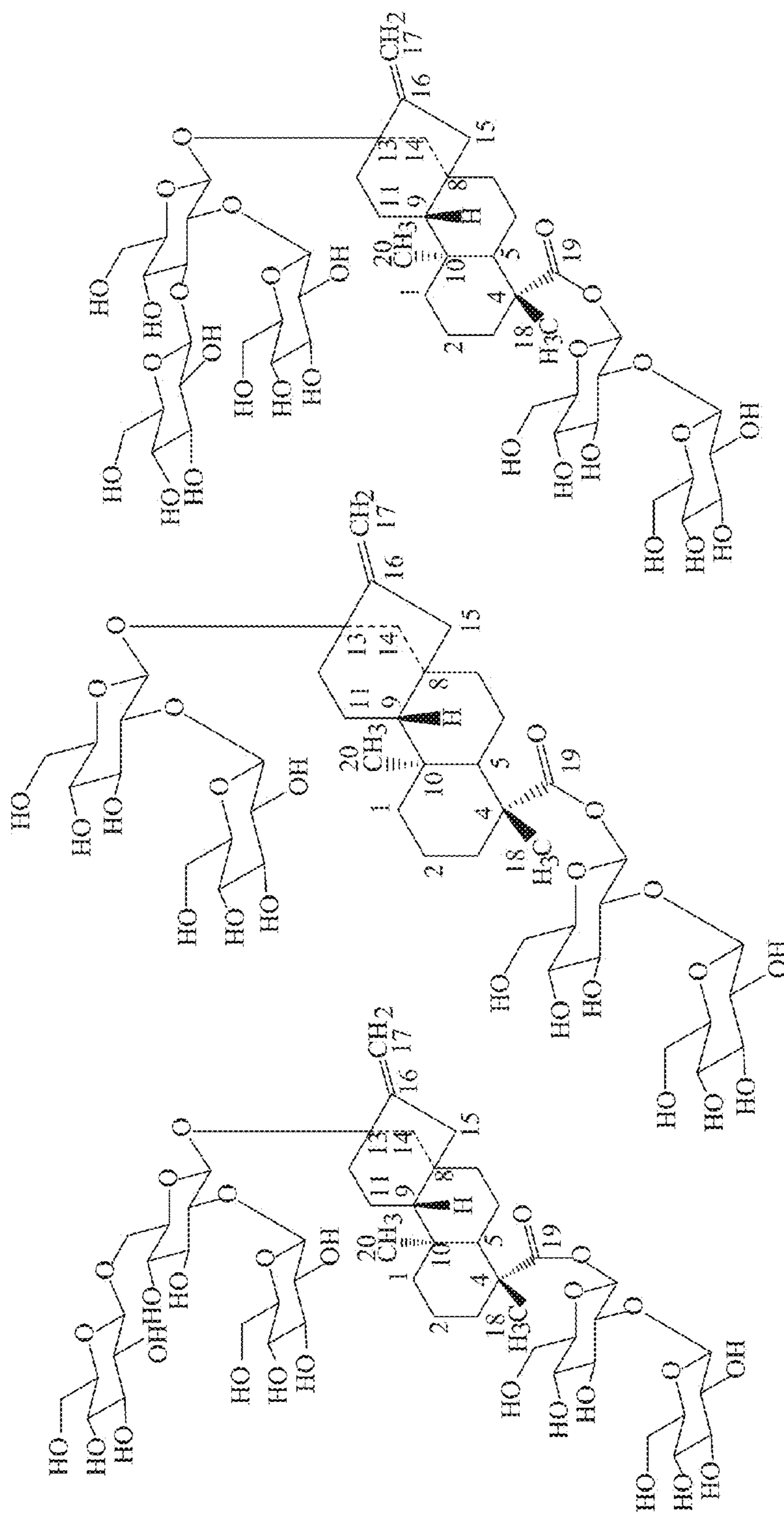
Rebaudioside D
