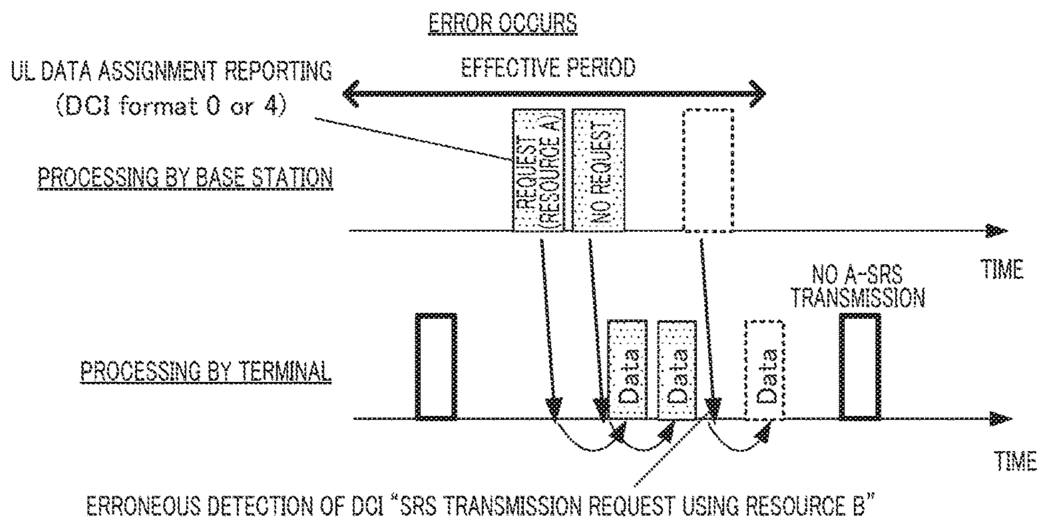
FIG. 7B
