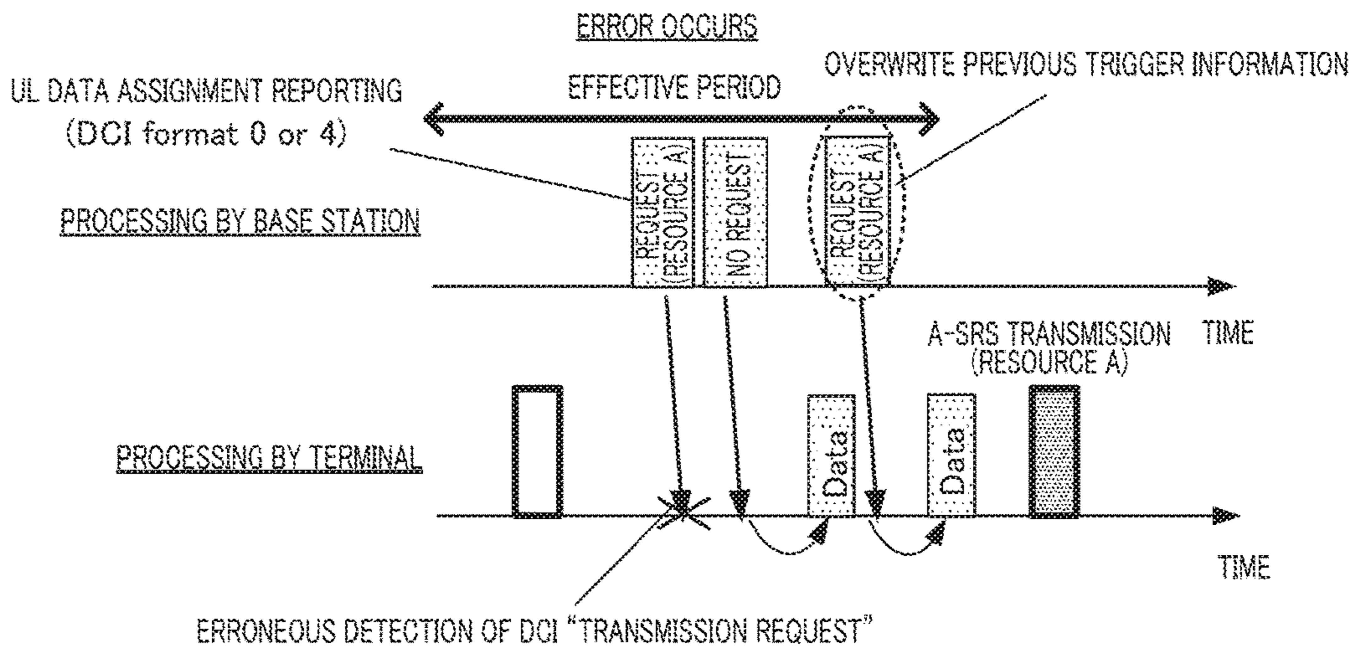
FIG. 6B
