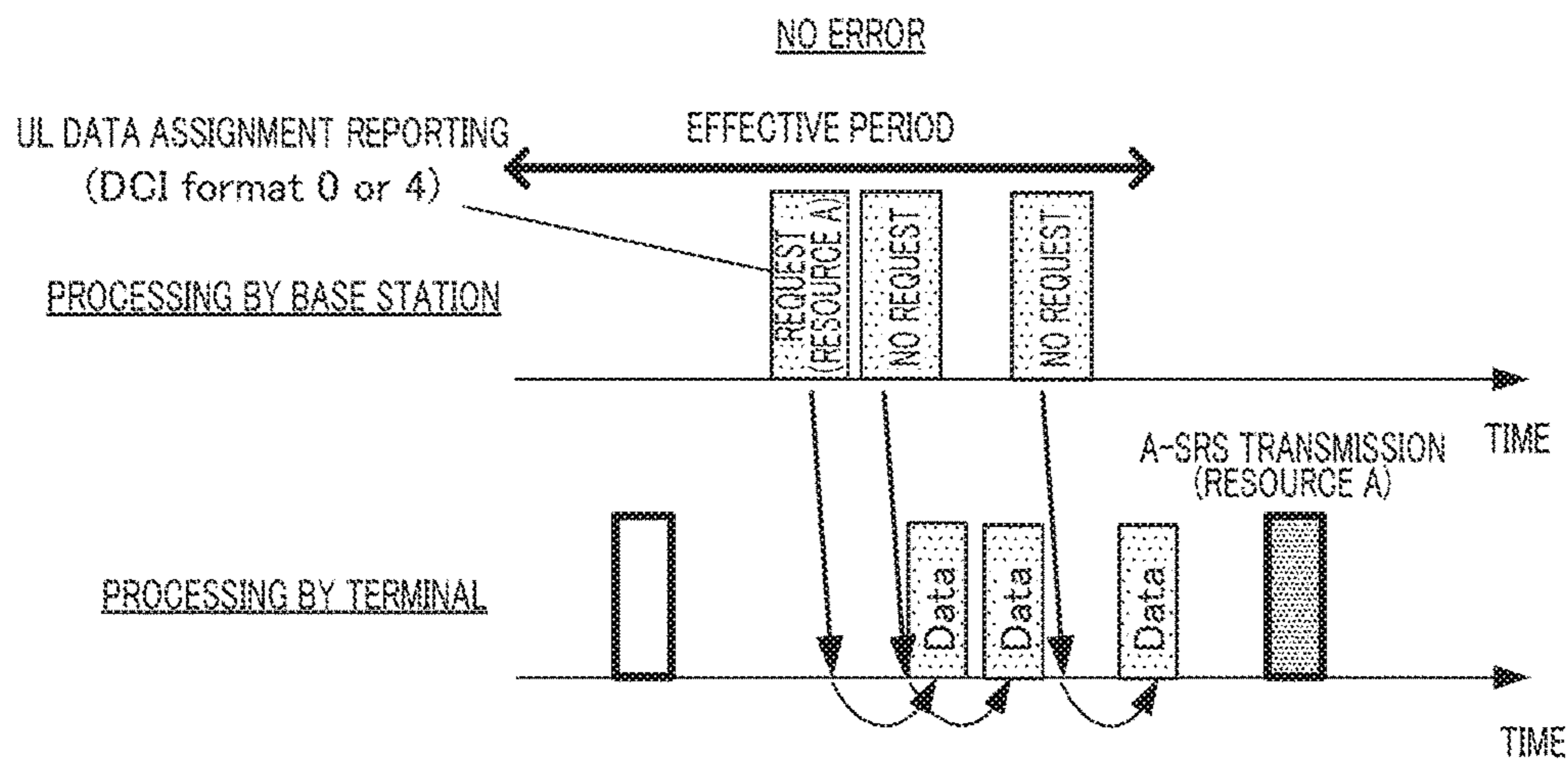
FIG. 7A
