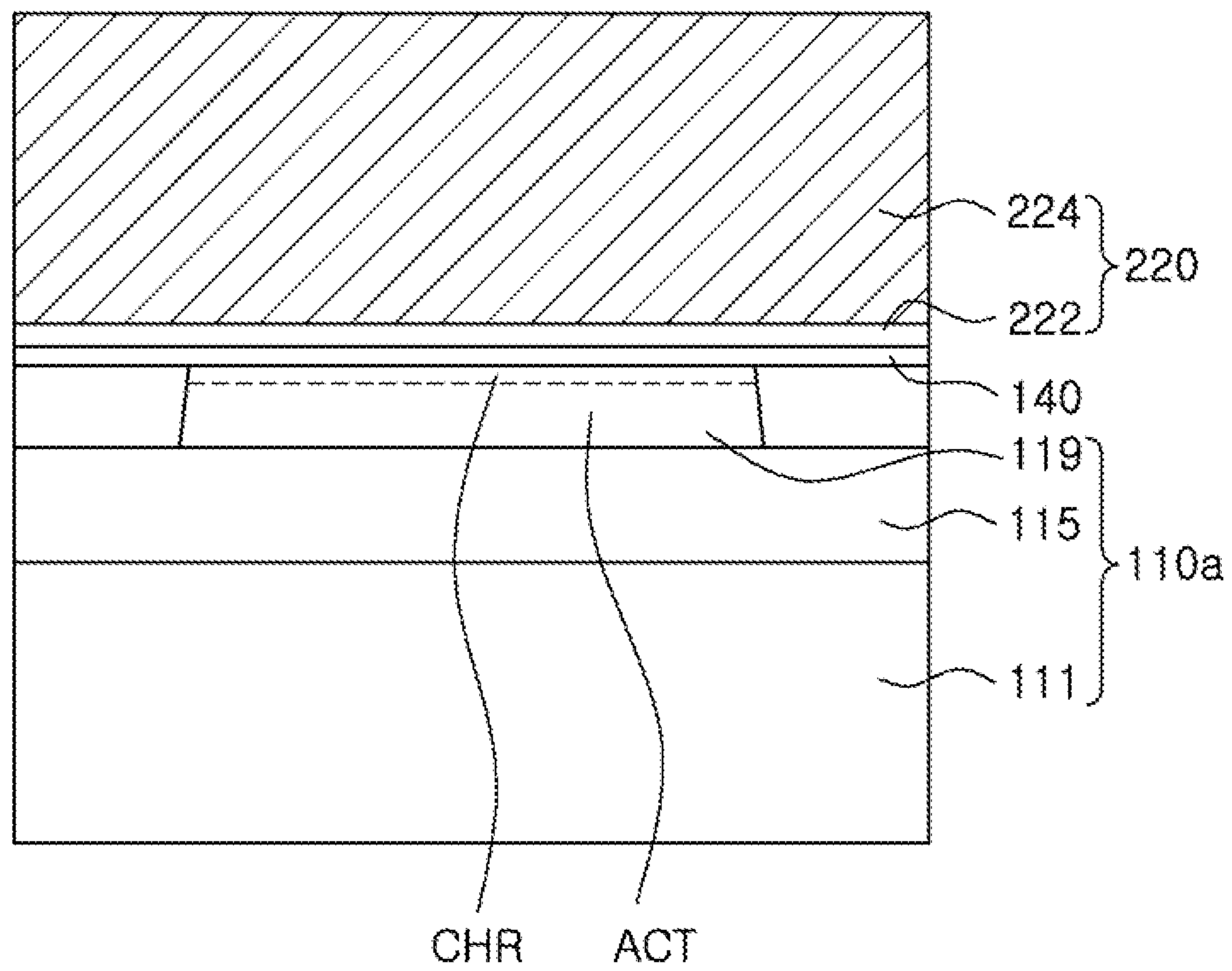
C - C' FIG. 7C
