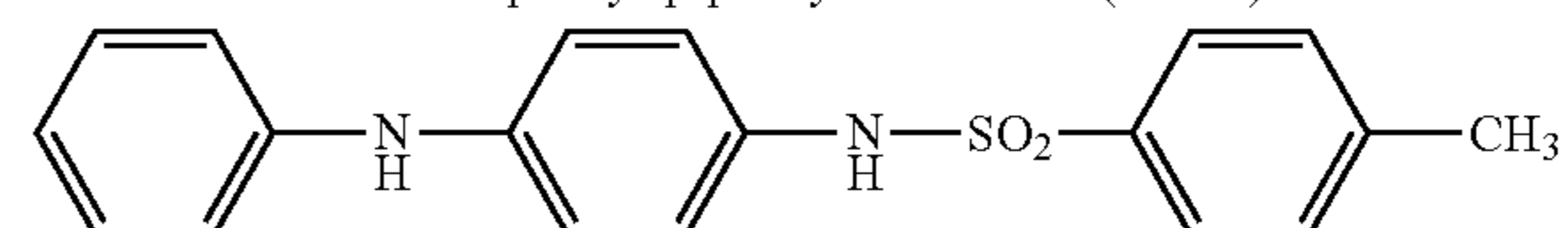
p'-(p-Toluenesulfonylamido)diphenylamine (TSDP)
