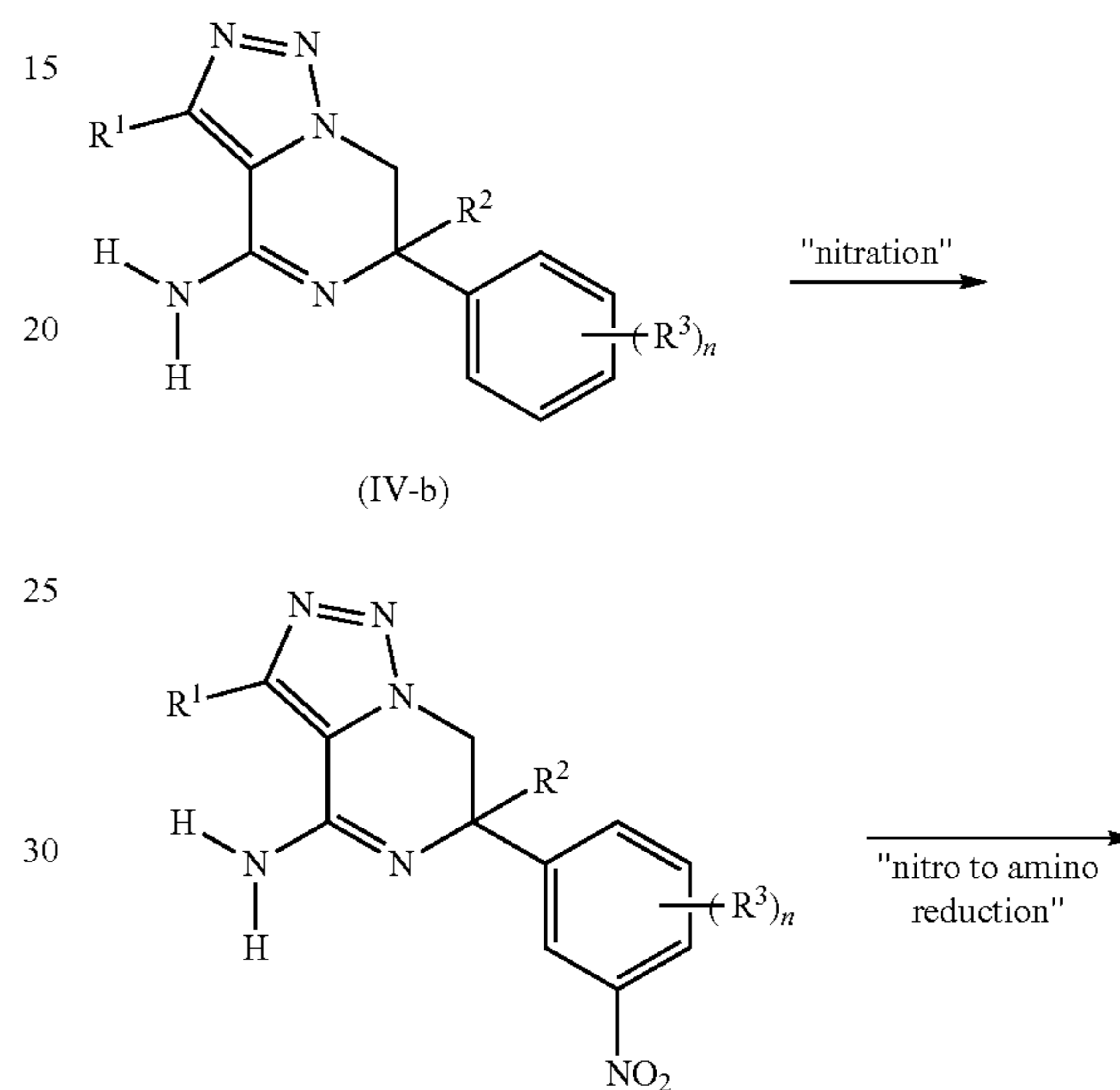
(II-c)
