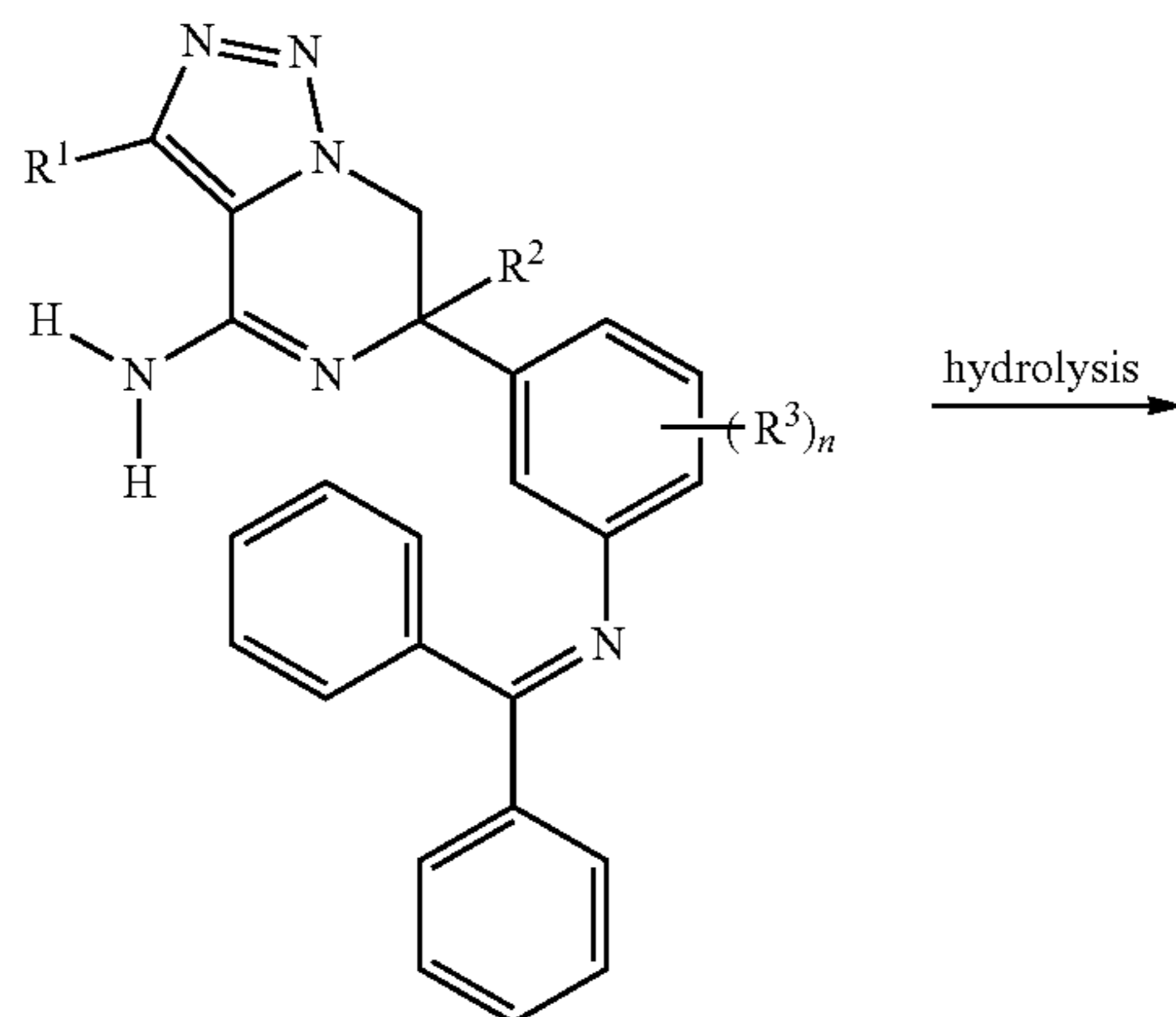
(II-b)
