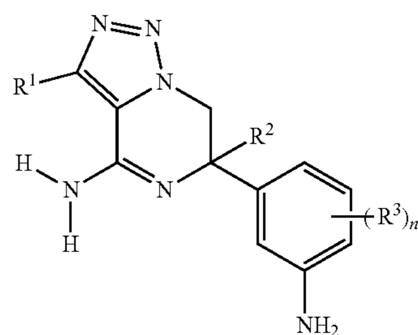
(II-a)
