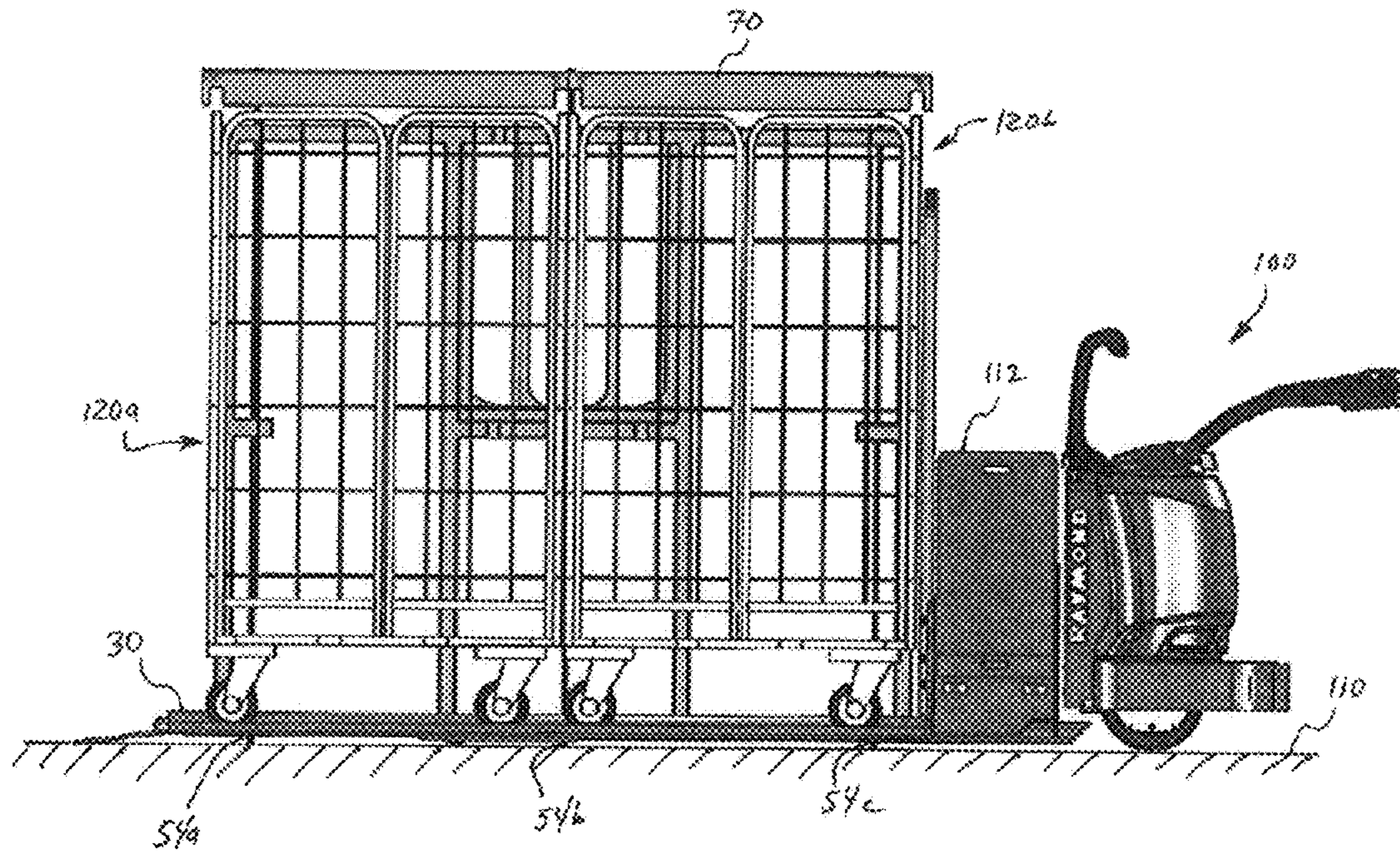
FIG. 7A
