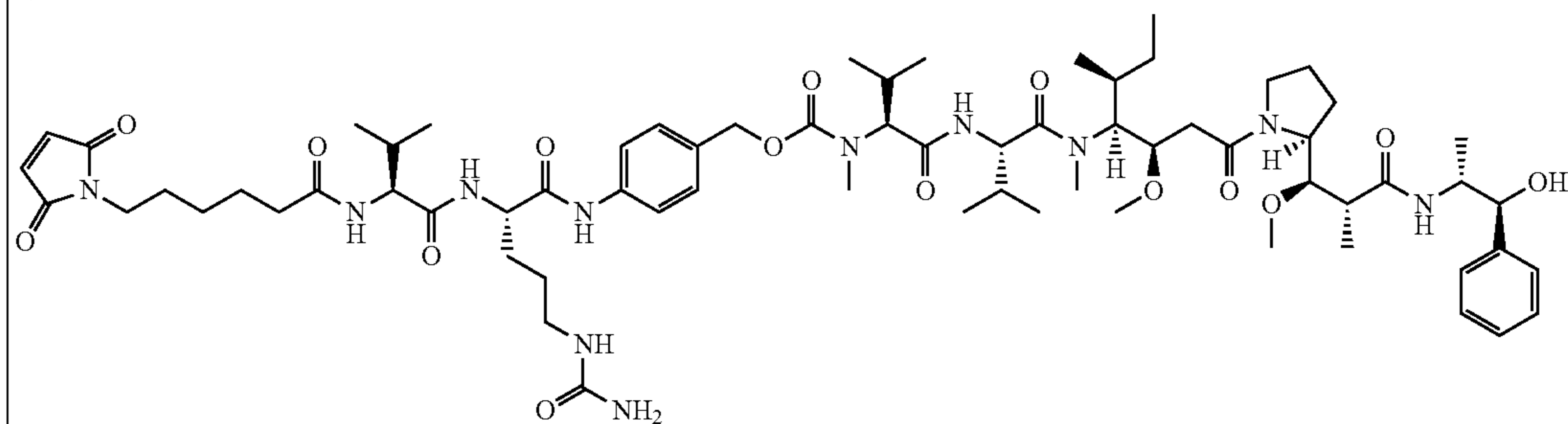
MC-Val-Cit-PABC-MMAE
