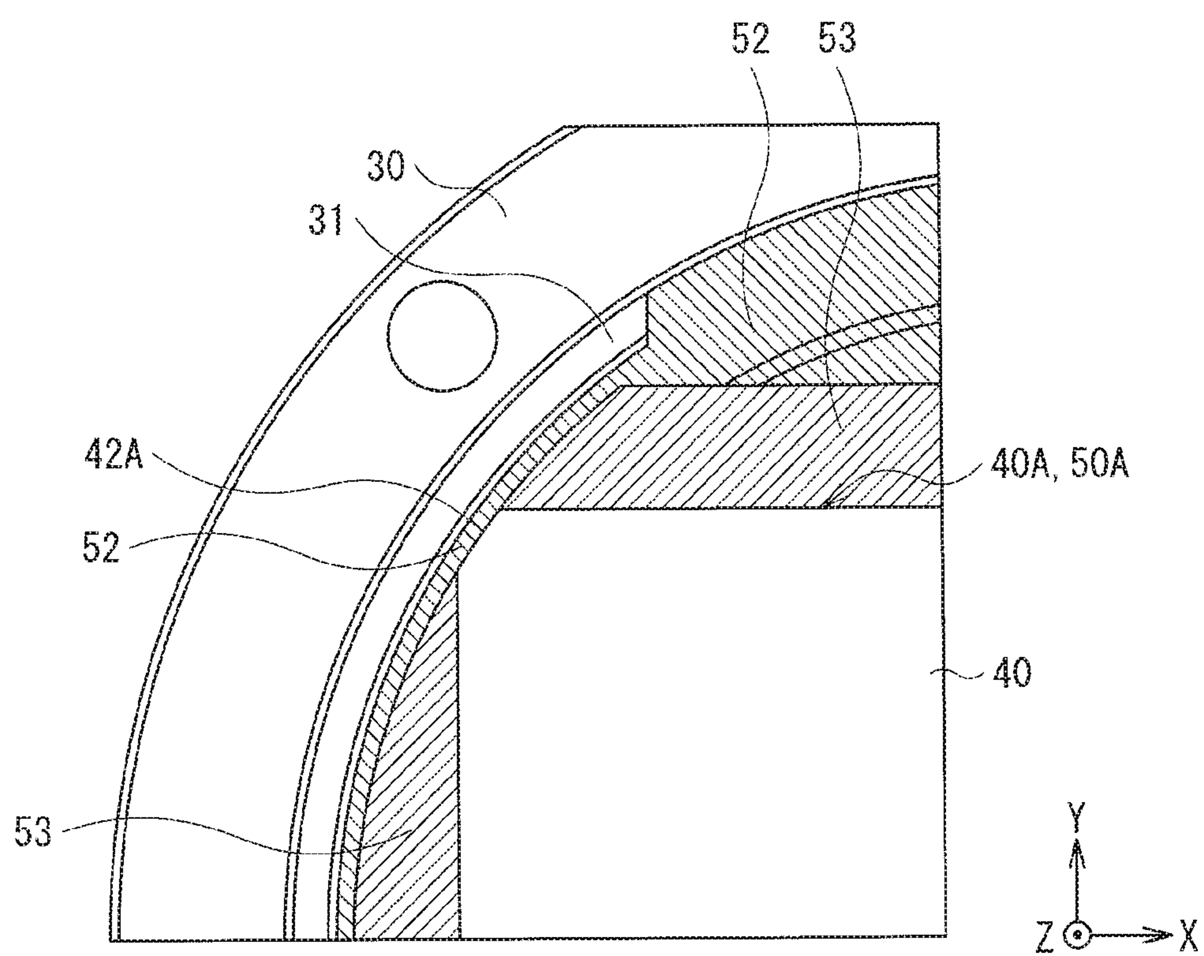
FIG. 10
