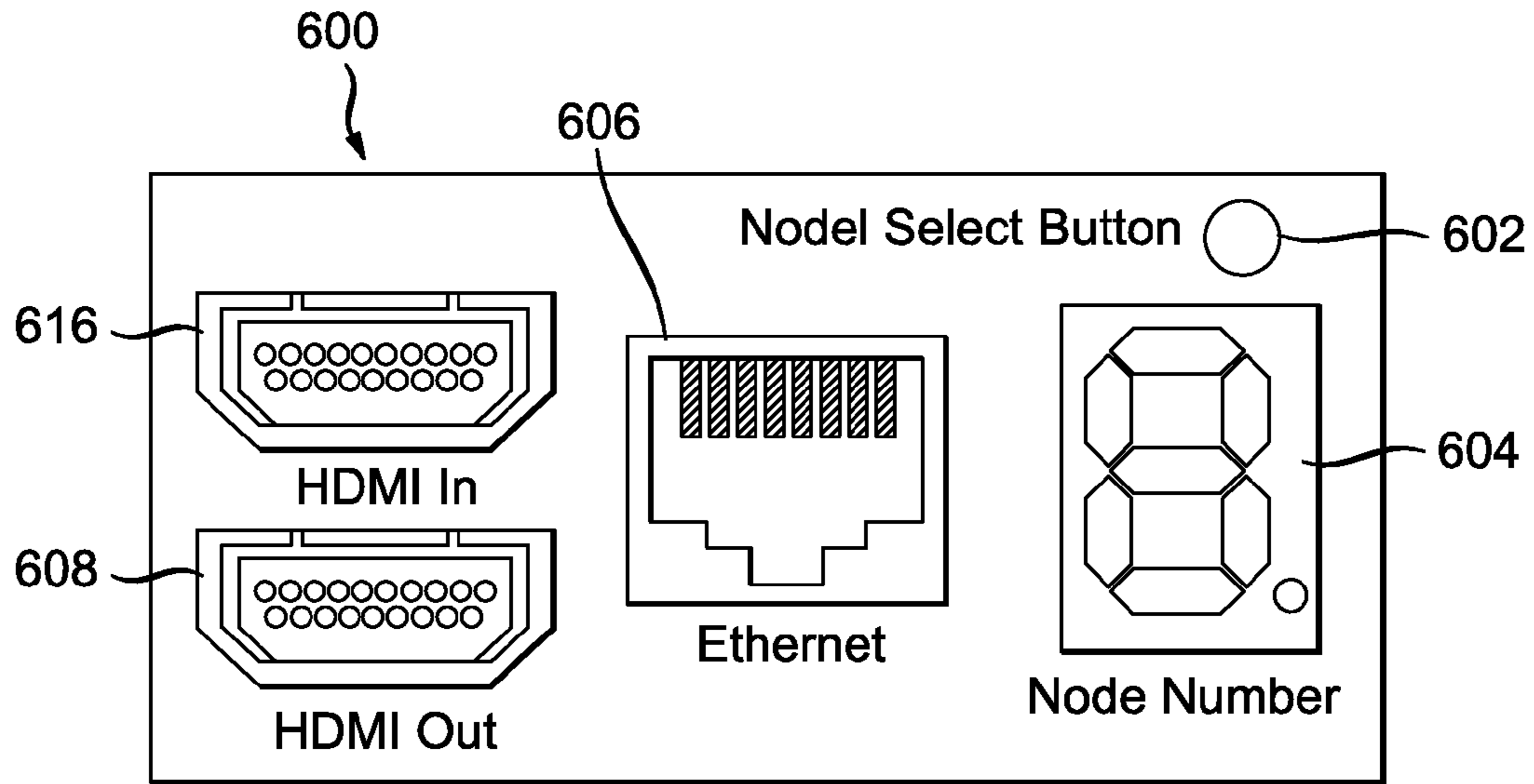
Simple AV Server Device Back Panel
