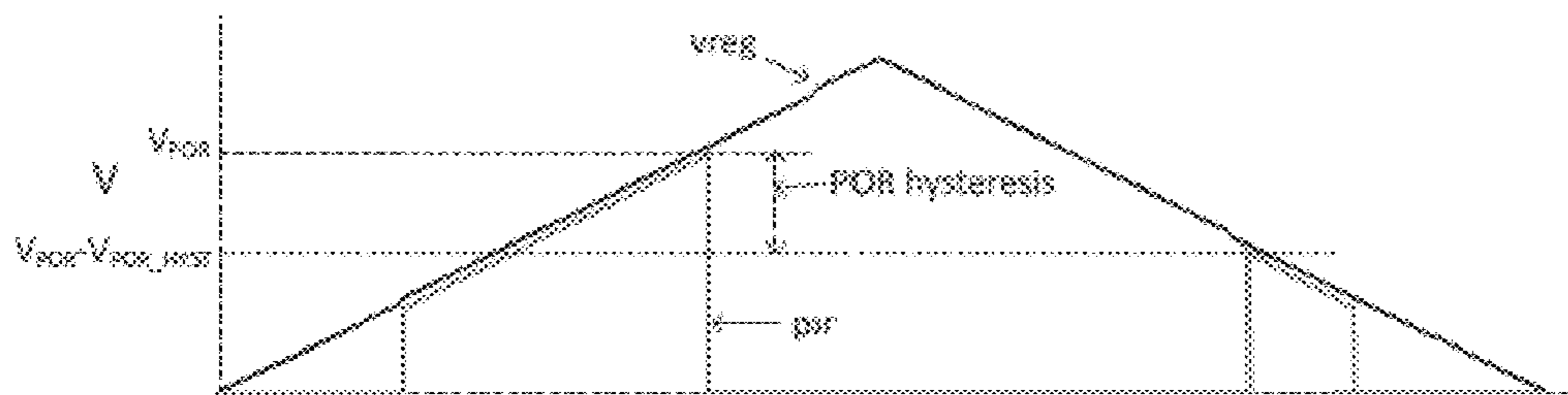
POR Threshold Voltages
