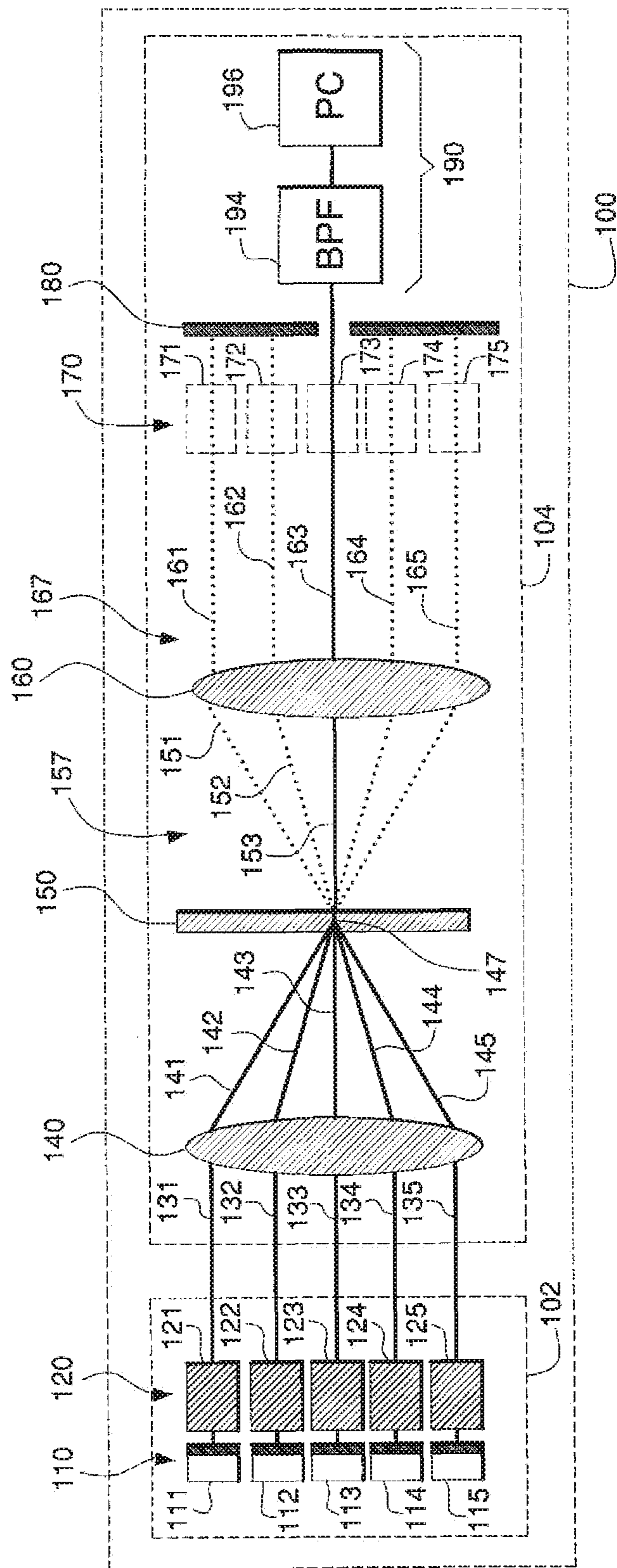
FIG. 1B
